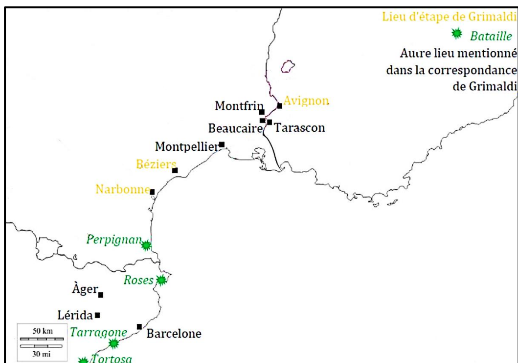
Figure 4. – Roussillon et Catalogne, 1642.
