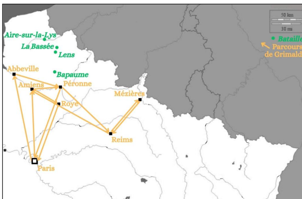
Figure 3. – Le nord de la France en 1641.
