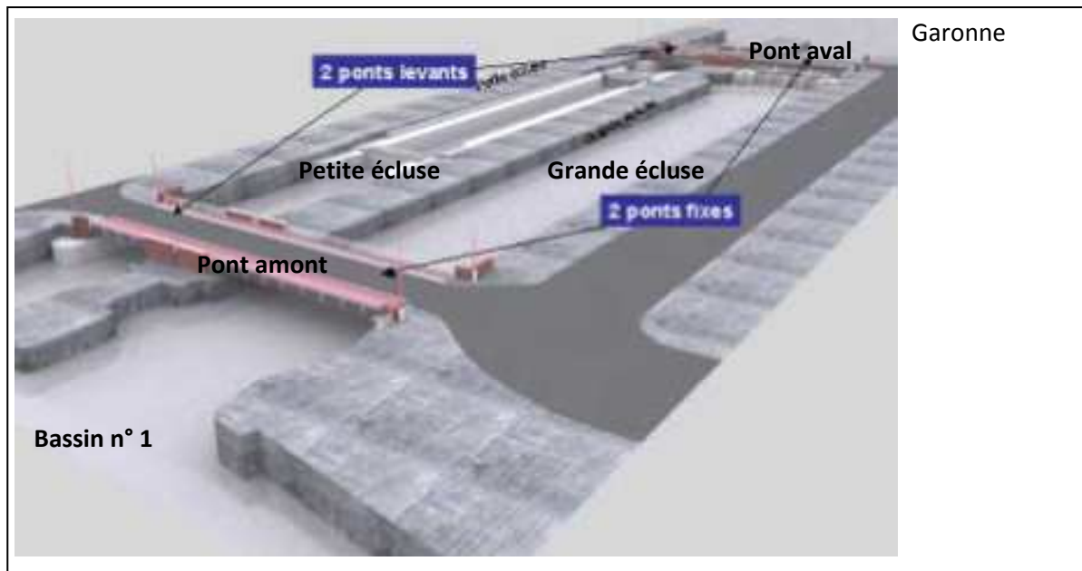
Figure n° P2-C3-F16. Les ponts du projet de modernisation des bassins à flot
