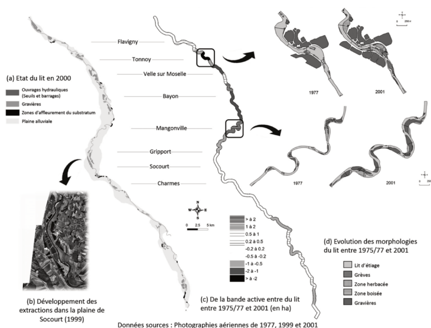
FIGURE 2.15 : Evolution de la dynamique de la Moselle à la suite de l'arrêt des extractions en lit mineur, d'après Beck and Corbonnois (2016)
