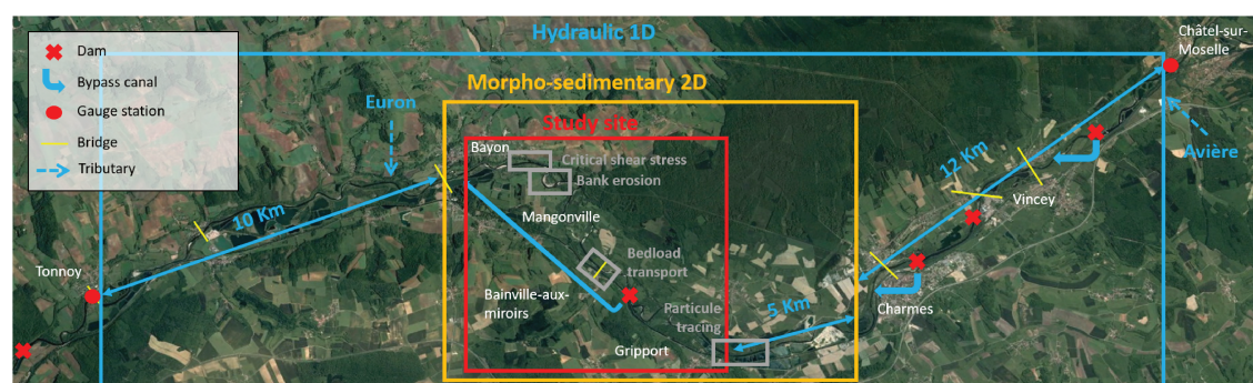
FIGURE 1.11 : Zone d'étude et emprises des différents modèles hydrauliques emboîtés, modèles de zooms en gris.
