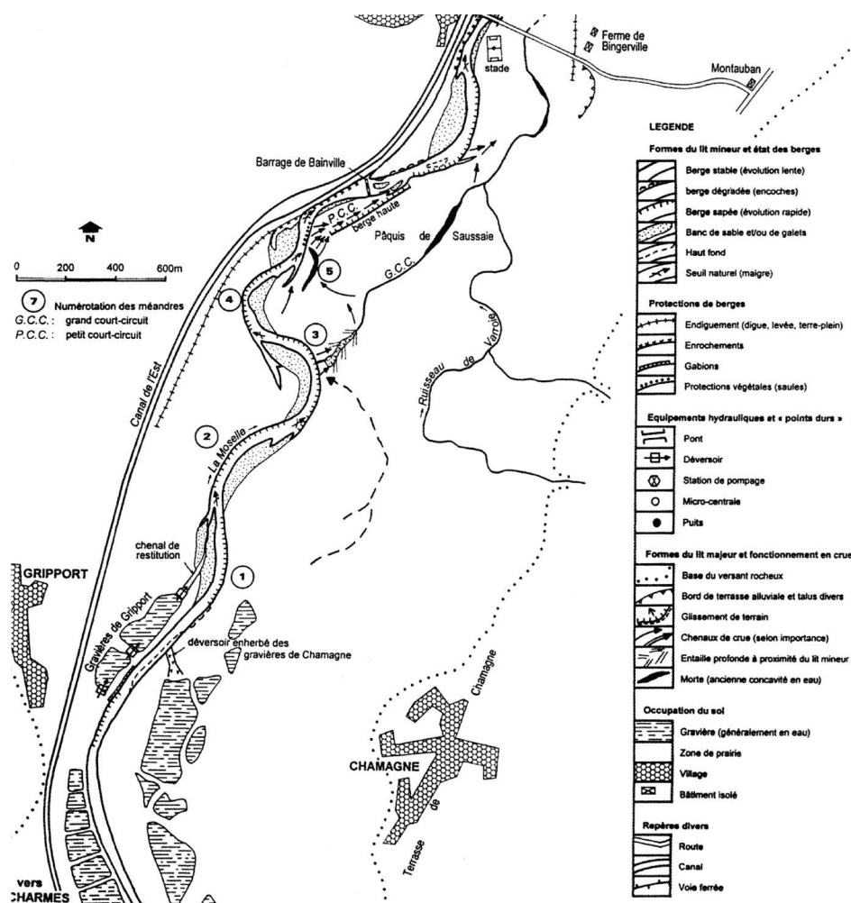
FIGURE 2.25 : Lit de la Moselle avec les principales structures du fond de vallée entre Charmes et Bainville en 2000, d'après Maire and Corbonnois (2000).
