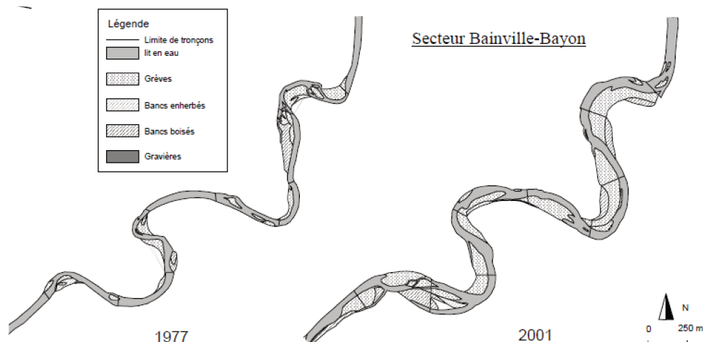
FIGURE 2.24 : Évolution de la bande active des méandres du grand travers, d’après Corbonnois et al. (2006)
