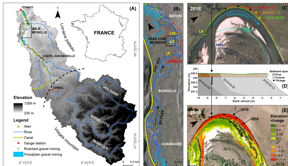
FIGURE 6.1 : (A) localisation du tronçon de la “Moselle sauvage” au sein du bassin versant de la Moselle, (B) extension longitudinale du modèle hydro-sédimentaire 2D “sto”, (C) suivi du recul de la berge concave du méandre de “la vache morte”, (D) profil en travers du recul de berge, (E) suivi du déplacement de traceurs placés dans la berge.
