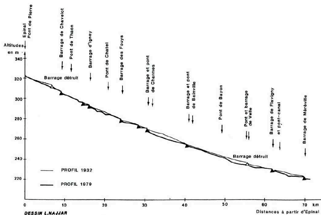
FIGURE 2.13 : Profil en long de la Moselle en 1932 et 1979, d'après Maire and Lasserre (1991)
