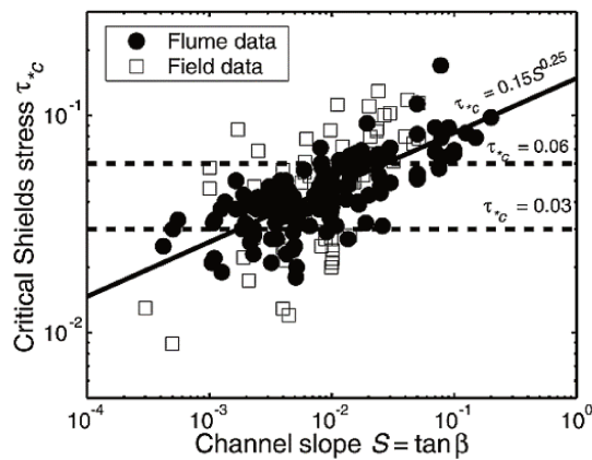
FIGURE 1.8 : Compilation de données montrant la variation du paramètre critique de Shields en fonction de la pente moyenne du fond, d'après Lamb et al. (2008).
