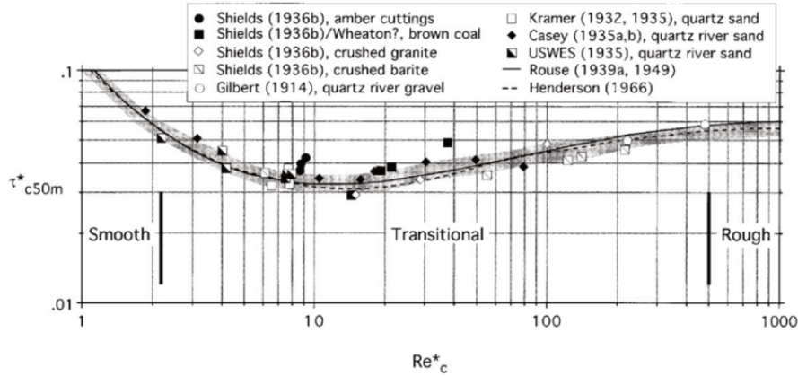
FIGURE 1.7 : Diagramme de Shields dans Garcia et al. (2000).
