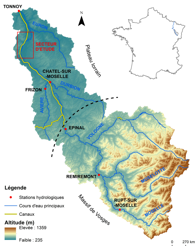
FIGURE 2.1 : Topographie du bassin versant de la Moselle en amont de Tonnoy
