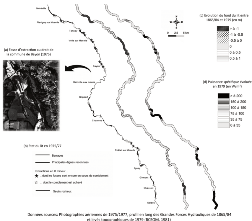
FIGURE 2.14 : Extraction de granulats en lit mineur et modification du cours d'eau, d'après Beck and Corbonnois (2016)
