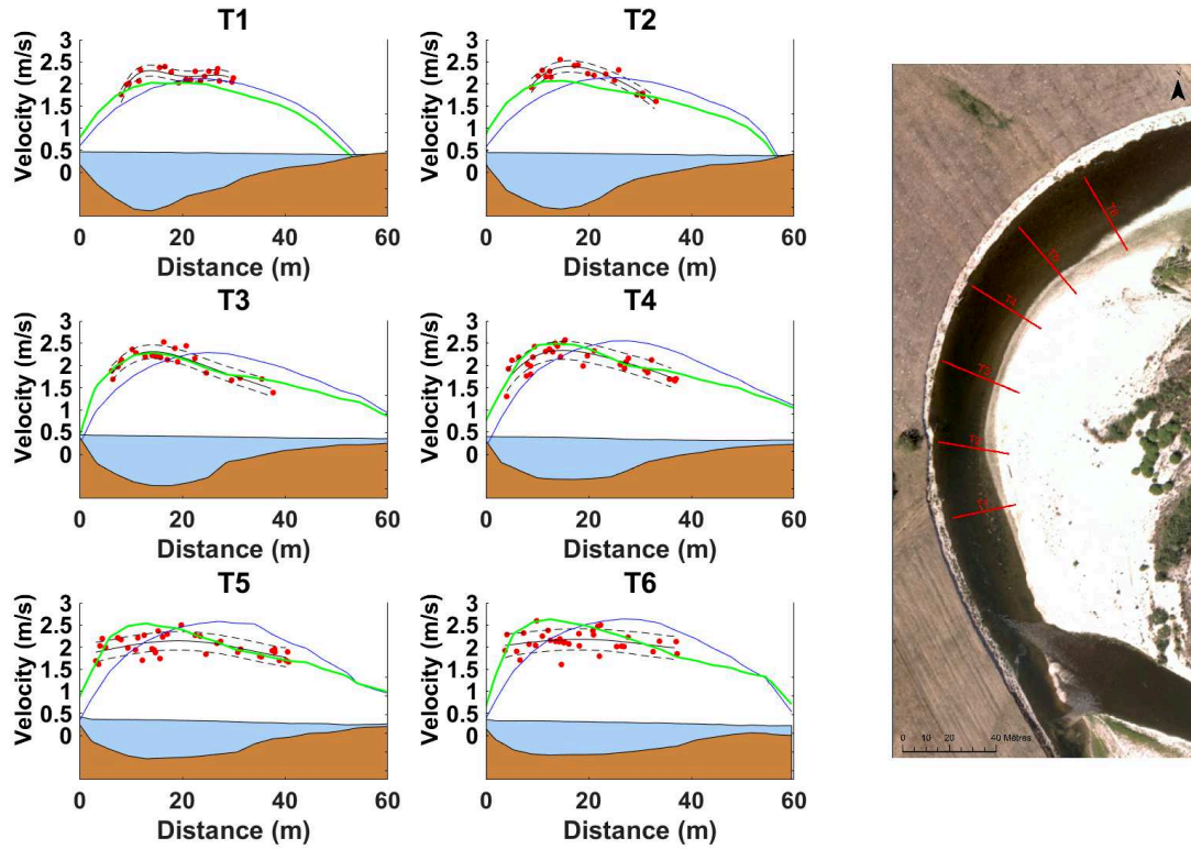
FIGURE 6.2 : Comparaison de profils de vitesse T_{n=1..6} mesurés par ADCP (points rouge) et modélisés avec (lignes vertes) ou sans (lignes bleues) correction, le long du méandre de "la vache morte", lors d'une crue de période de retour d'un an ( Q = 180 m^3/s ).
