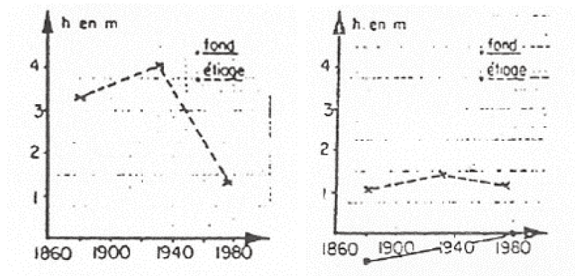
FIGURE 2.21 : Evolution du lit à Charmes (gauche) et Bainville (droite) (BCEOM, 1981)
