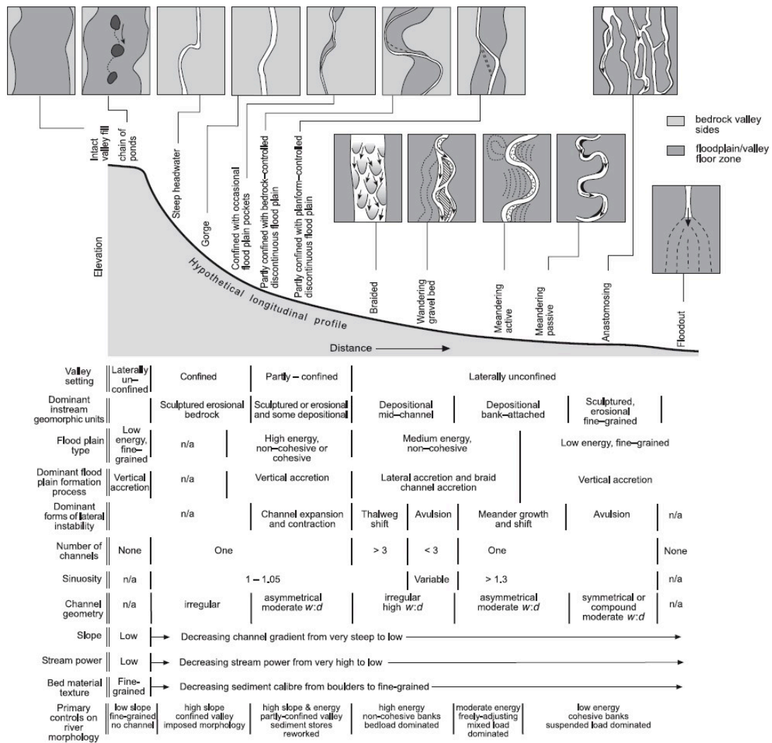
FIGURE 1.3 : Vue longitudinale et en plan des formes et processus fluviaux et des facteurs de contrôle associés, d'après Brierley and Fryirs (2013).
