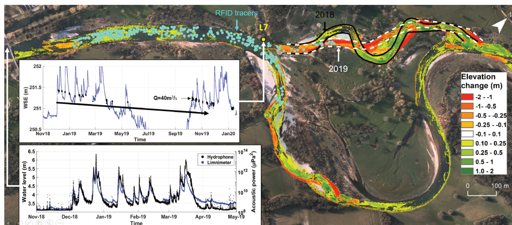
FIGURE 6.5 : Jeu de données sur le méandre recoupé : évolution bathymétriques issues des relevés LiDAR 2018 et 2019; Chronique temporelle de niveau d'eau mesurée par le limnimètre L7 à l'amont du recouplement (niveau d'eau en trait bleu et en points noirs niveaux d'eau pour une valeur de débit égale au module de 40m^3/s ); Chronique temporelle de la puissance acoustique enregistrée par l'hydrophone fixé à la pile du pont.
