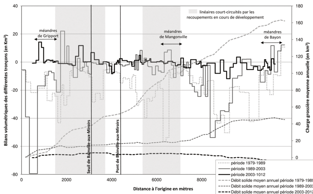
FIGURE 2.23 : Evolution des volumes charriés de 1979 à 2012 d'après, Beck and Corbonnois (2016)
