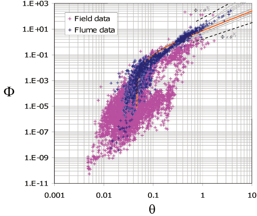
FIGURE 1.9 : Compilation de 8700 mesures collectées sur plus de 100 cours d'eau (pente 0.0001 < S < 0.1 ) et de 1317 mesures issues du laboratoire (matériaux quasi-uniformes) avec la courbe rouge représentant la relation de Meyer-Peter and Müller (1948), modifié d'après Recking (2012a) et Recking (2006).
