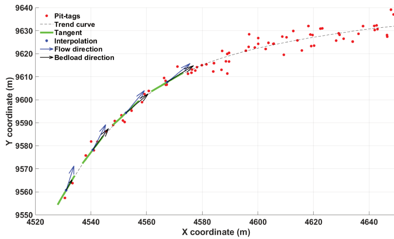
FIGURE 6.3 : Comparaison de la direction du transport sédimentaire modélisé le long du méandre de “la vache morte”, lors d’une crue de période de retour d’un an ( Q = 180 \text{ m}^3/\text{s} ) par rapport à la trajectoire de traceurs provenant de l’érosion de la berge concave.
