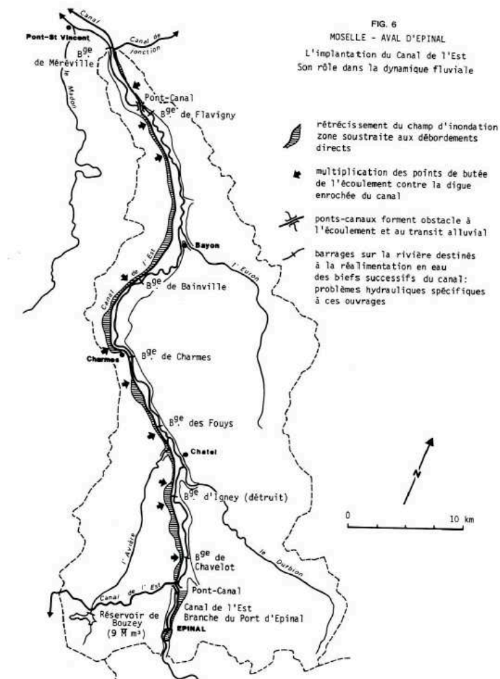
FIGURE 2.12 : Implantation du Canal de l'Est et son rôle dans la dynamique latérale de la Moselle, d'après Maire and Lasserre (1991)
