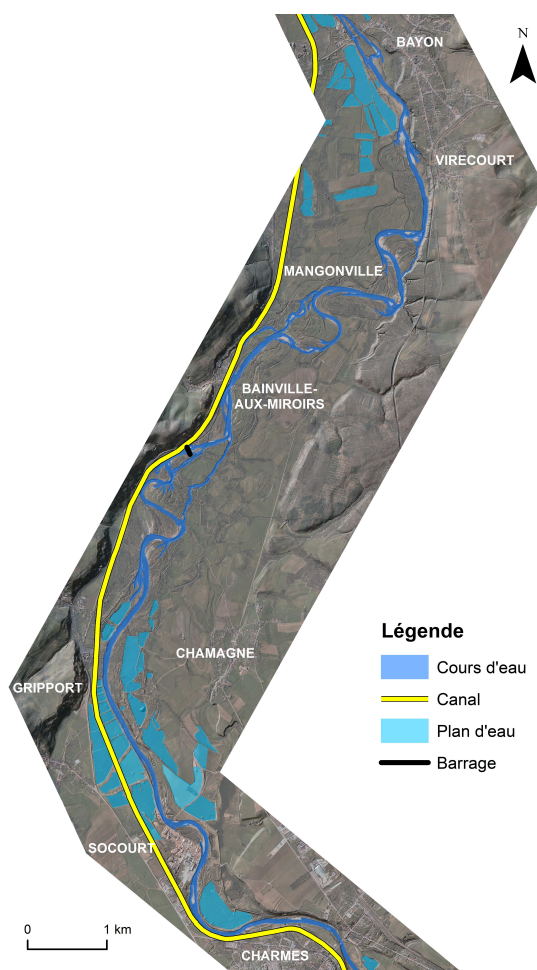
FIGURE 2.4 : Linéaire d'étude de la Moselle entre Charmes et Bayon
