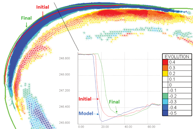
FIGURE 6.4 : Résultat préliminaire de la modélisation de l’érosion de la berge concave du méandre de “la vache morte”, simulée par le modèle hydro-morphologique “sto”, pour une crue de période de retour d’un an ( Q = 180 \text{ m}^3/\text{s} ).
