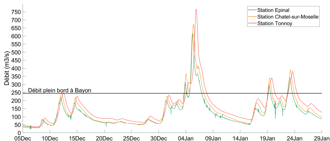
FIGURE 2.9 : Hydrogramme de la Moselle au cours de l'hiver 2017-2018 (Banque hydro)
