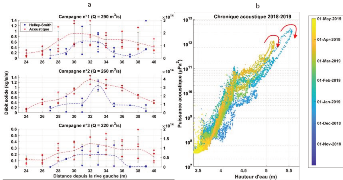
Figure 1 : Comparaison des mesures par prélèvements Helley-Smith et jaugeages acoustiques le long de la section en travers (a) et chronique de la variation de la puissance acoustique en fonction de la hauteur d'eau (b).
