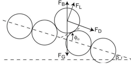
FIGURE 1.6 : Bilan des forces s'exerçant sur une particule au sein d'un écoulement, d'après Lamb et al. (2008).
