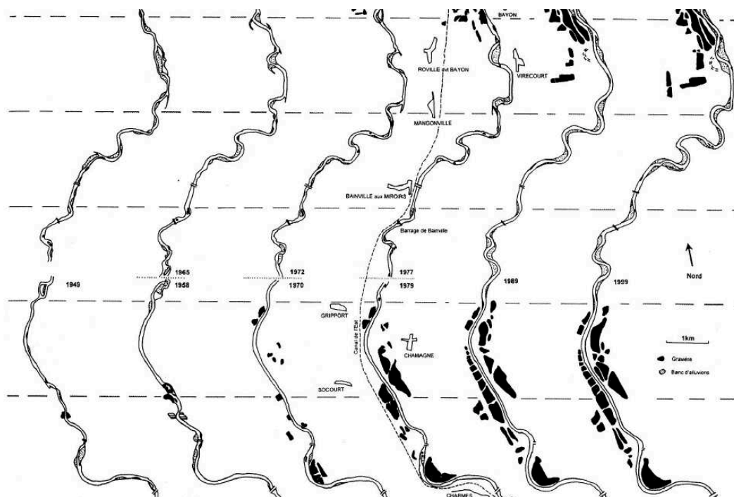
FIGURE 2.20 : Evolution du lit et du milieu riverain de la Moselle entre 1950 et 2000, d'après Maire and Corbonnois (2000)
