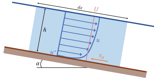
FIGURE 1.5 : Bilan des forces s'exerçant sur un volume d'eau en écoulement uniforme et répartition verticale des vitesses d'écoulement sur la colonne d'eau.
