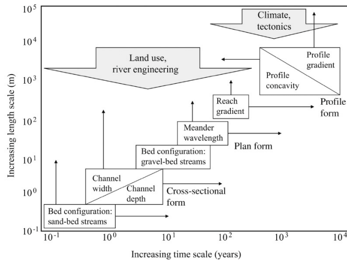
FIGURE 1.4 : Echelles temporelles et spatiales de l'ajustement des différentes composantes morphologiques du chenal. Les longueurs, indicatives, sont appliquées à un cours d'eau tempérés, d'après Knighton (1998).
