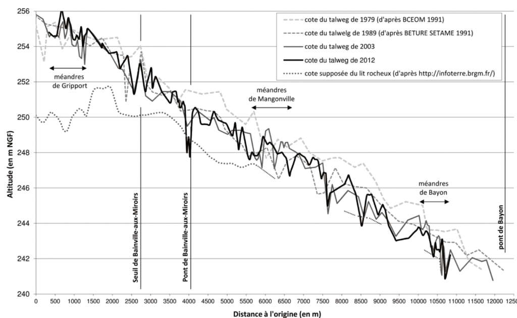
FIGURE 2.22 : Evolution du profil en long de la Moselle sur le secteur Gripport-Bayon, d'après Beck and Corbonnois (2016)
