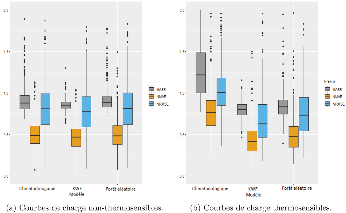
FIGURE 4.19 – Les boîtes à moustaches des erreurs MASE, NMAE et NRMSE par modèle de prévision (climatologique, KWF et forêt aléatoire).
