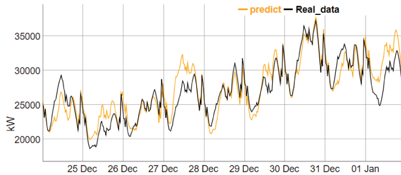
FIGURE 5.26 – Extrait des courbes prévisionnelles de la semaine de Noël en 2019 par le modèle GAM montrant l’adaptabilité du modèle GAM aux fluctuations des pertes durant les jours fériés : la courbe orange représente les prévisions tandis que la courbe noire correspond aux données réelles de pertes électriques.
