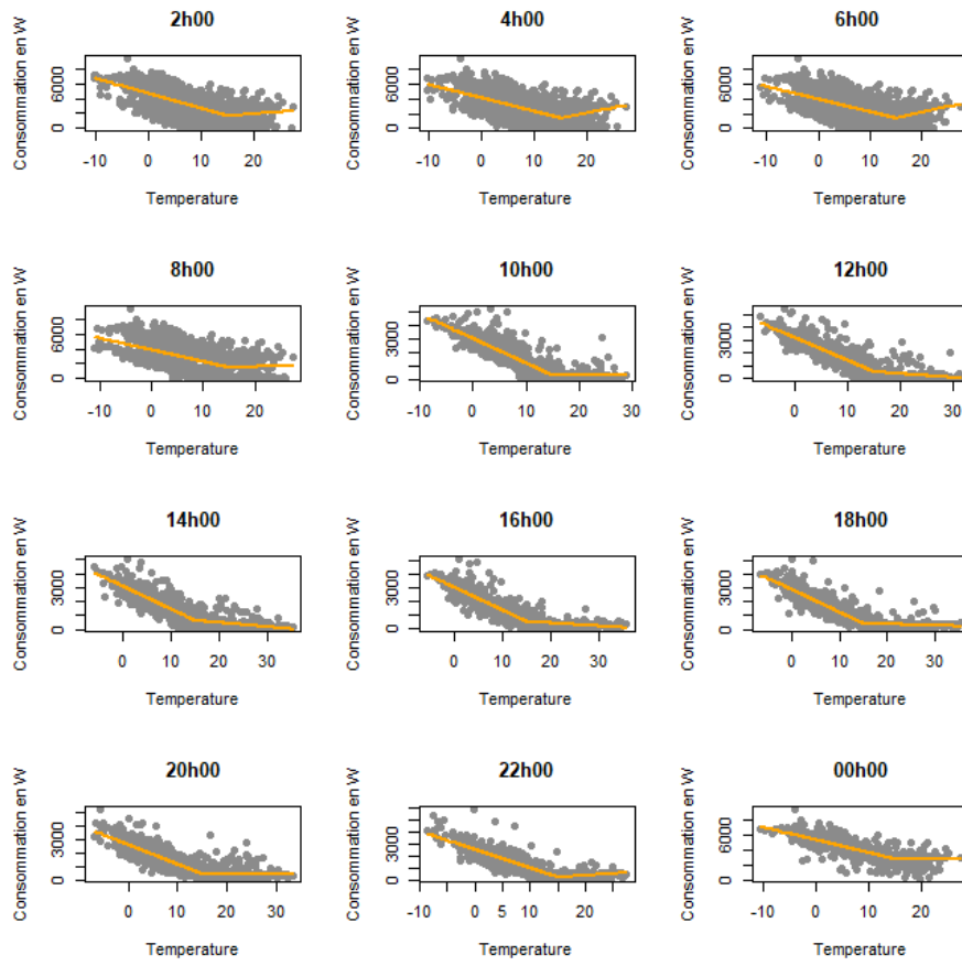
FIGURE 4.12 – Des nuages de points montrant la consommation d’électricité en W au pas demi-horaire (axe y) en fonction de la température extérieure en ^{\circ}\text{C} (axe x) à différentes heures de la journée du ménage thermosensible 2 de la figure 4.11b.
