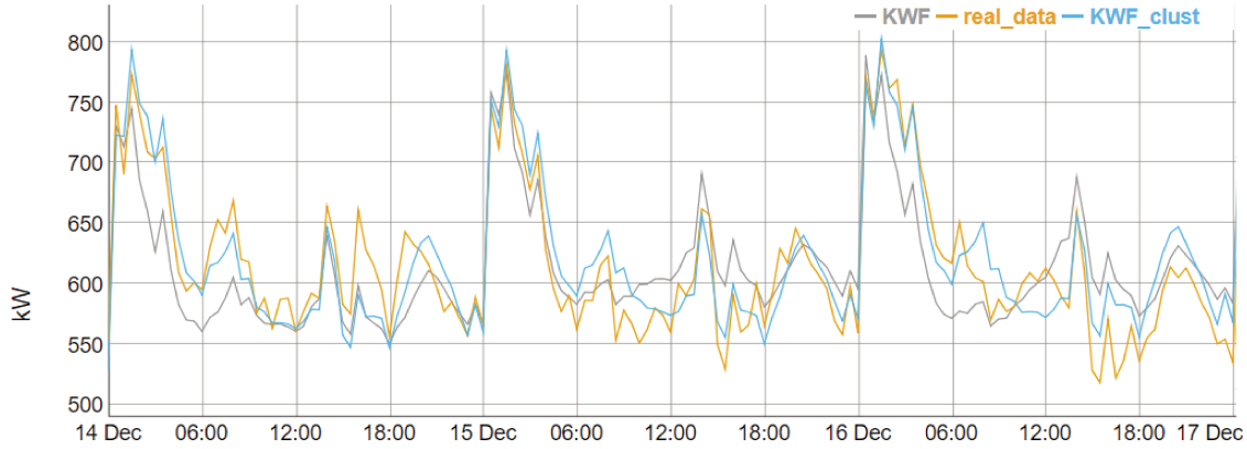
FIGURE 4.37 – Exemple de prévision à (J + 1) de la courbe de charge agrégée des ménages thermosensibles par le modèle KWF (courbe en gris) et par le modèle KWF avec clustering (courbe en bleu ciel). La courbe en orange représente la charge électrique agrégée réelle en kW.
