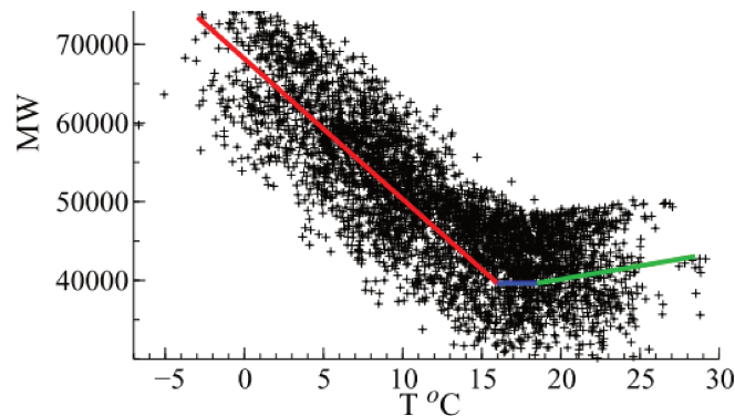
FIGURE 4.10 – Graphique montrant la relation entre la température moyenne journalière en ^{\circ}\text{C} et la demande moyenne journalière de la France en MW. [Source (DORDONNAT et al., 2008)].
