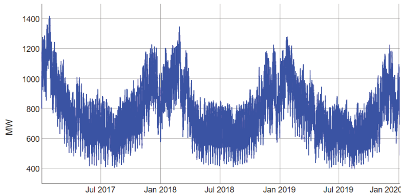
FIGURE 5.31 – Courbe de charge électrique du réseau de distribution pour la période du 1 janvier 2017 au 1 janvier 2020.
