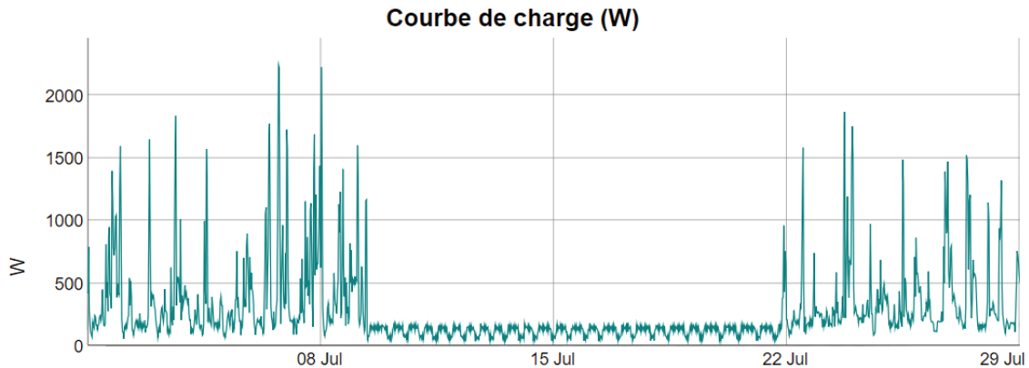
FIGURE 4.6 – Extrait d'une courbe de charge d'un ménage montrant une période de vacances entre le 09 juillet et le 21 juillet 2018.
