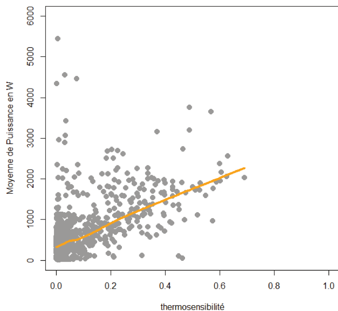
FIGURE 4.13 – Nuage de points montrant la moyenne de la consommation journalière des ménages dans le jeu de données en fonction de la thermosensibilité de ces derniers.
