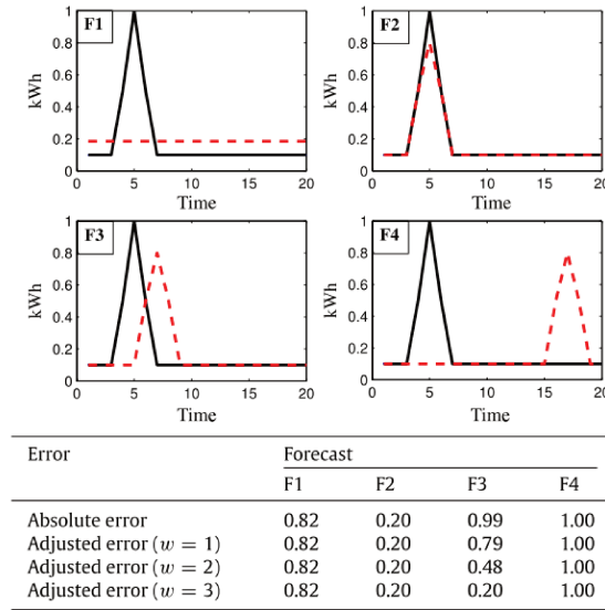
FIGURE 3.4 – Les quatre graphiques représentant les différentes prévisions F_1, F_2, F_3 et F_4 (ligne en pointillés rouge) d’une courbe de charge (ligne noire continue) ainsi que les erreurs absolues ( w=0 ) et ajustées ( w=1, 2 et 3 ) de la p -norme [source (HABEN, WARD et al., 2014)].
