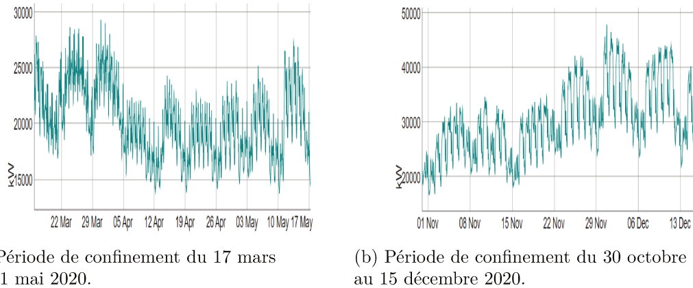
FIGURE 5.29 – L’impact des périodes de confinement sur les pertes d’électricité.
