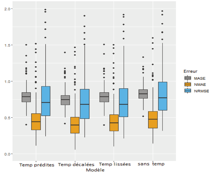
FIGURE 4.40 – Les boîtes à moustaches des erreurs de prévision à (J + 1) par les quatre modèles GAM : le modèle avec les prévisions de la température, le modèle avec la température décalée, le modèle avec les prévisions lissées de la température et le modèle sans température respectivement de gauche à droite.
