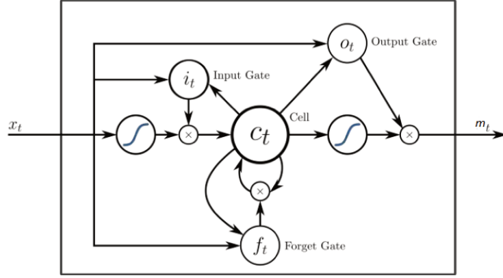
FIGURE 4.44 – Une repr sentation d'une cellule LSTM avec peephole , la porte d'entr e ( i_t ), la porte d'oubli ( f_t ) et la porte de sortie ( o_t ) [Source devoteam] 18 .
