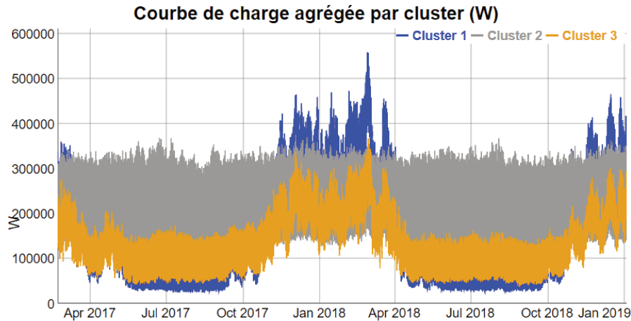
FIGURE 5.9 – Les courbes de charge électrique agrégées par cluster (cas où k = 3 ) de la période allant du 1 avril 2017 jusqu'au 30 janvier 2019.
