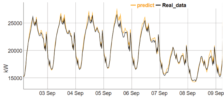
FIGURE 5.24 – Exemple des courbes prévisionnelles par le modèle GAM pour la semaine de 2 à 9 septembre 2019, avec les prévisions en orange et les données réelles de pertes en noir.
