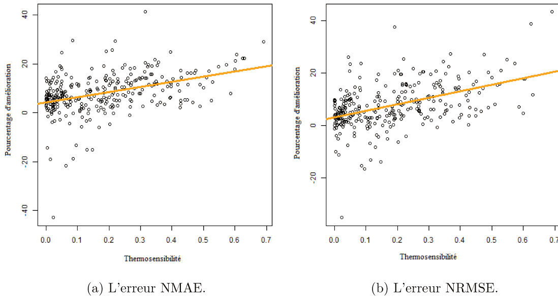
FIGURE 4.29 – Nuage de points du pourcentage de l'amélioration de l'erreur NMAE et l'erreur NRMSE du modèle KWF avec clustering par rapport au modèle KWF en fonction de la thermosensibilité du ménage.
