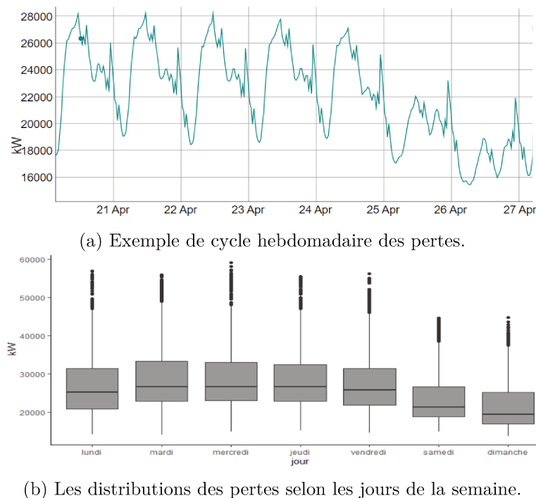
FIGURE 5.22 – Exemples de la saisonnalité hebdomadaire des données de pertes.
