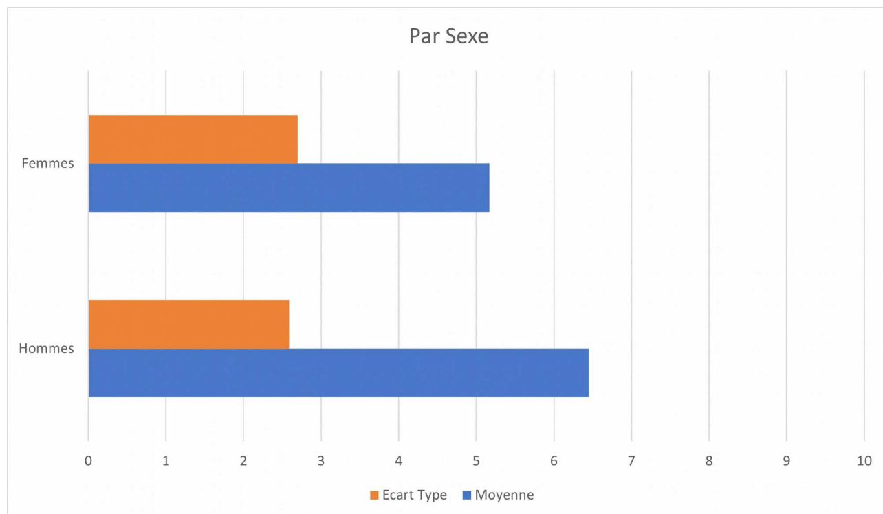
Figure 8: Écart type - Par sexe
