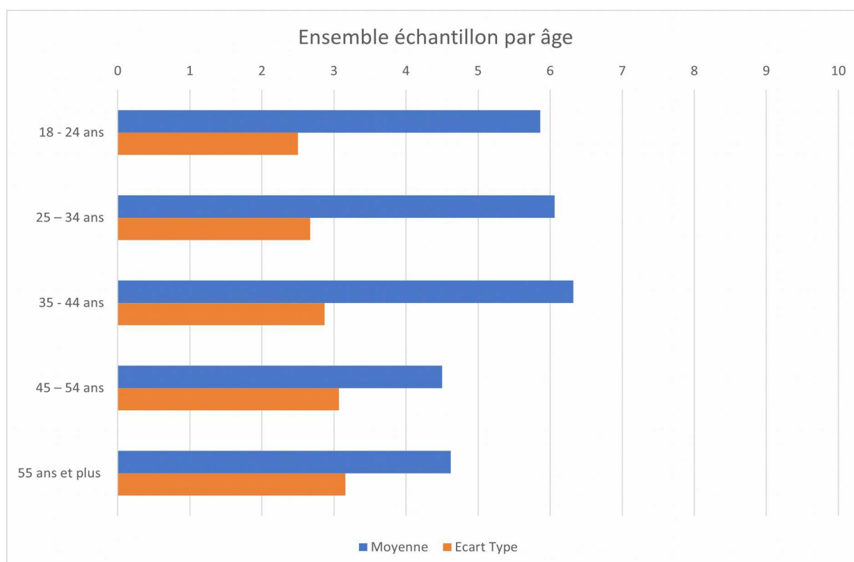
Figure 7: Écart type - Ensemble de l'échantillon par âge
