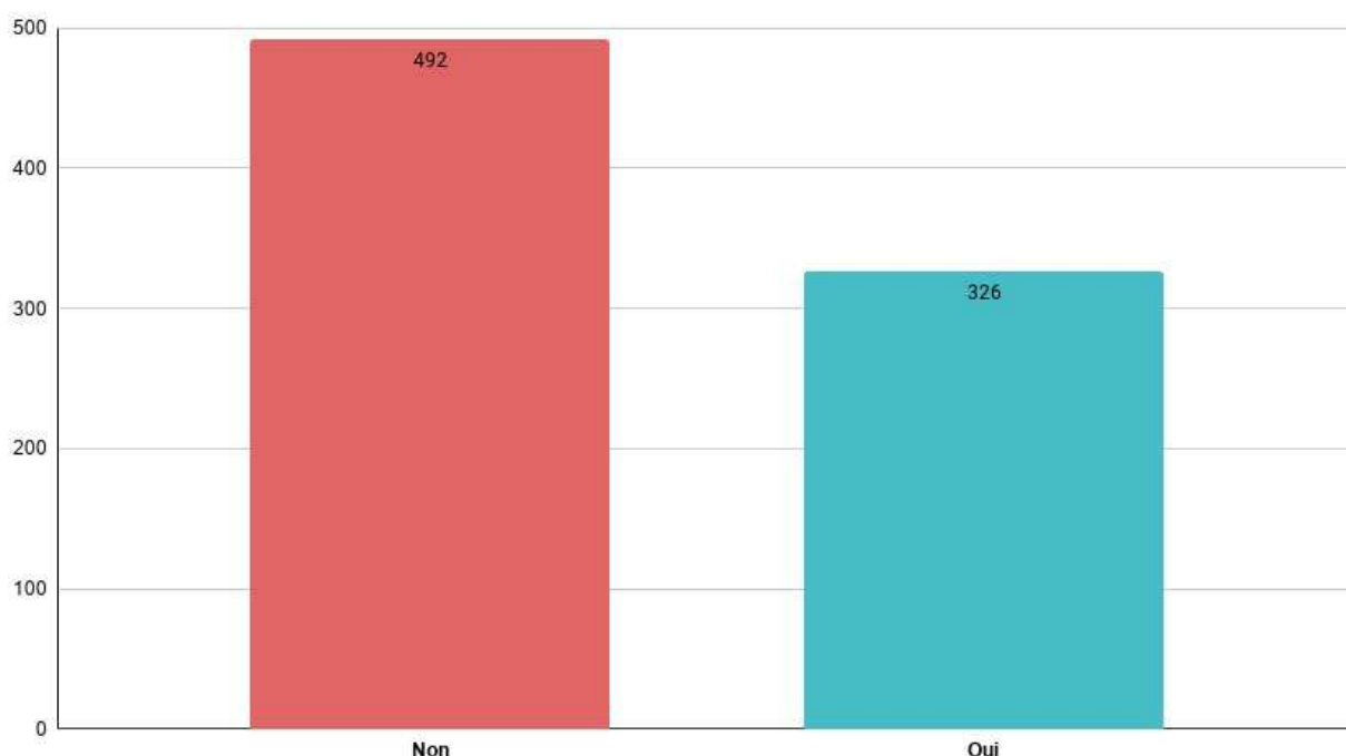
Figure 15 : Pensez-vous que les super-héros ont un impact dans votre vie personnelle ?
