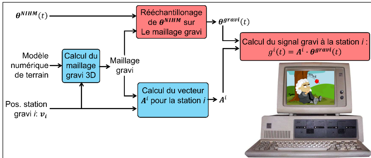
Figure 5.4 Schéma de principe du code de calcul hydro-gravimétrique direct. Les cases bleues correspondent aux calculs qui doivent seulement être effectués pour le premier pas de temps. Les cases rouges correspondent aux calculs qui doivent être effectués à chaque pas de temps.
