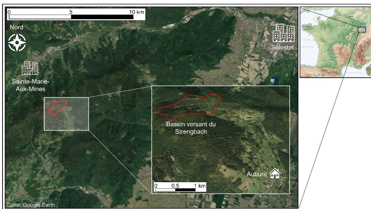
Figure 2.1 Localisation du bassin versant du Strengbach au sein du massif des Vosges.
