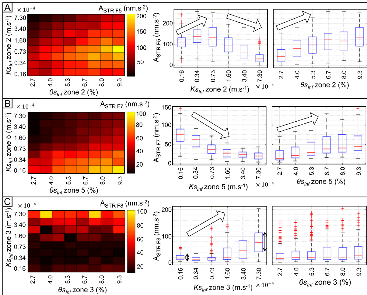
Figure 5.10 Influence des paramètres K_{s_{inf}} et \theta_{s_{inf}} des zones locales sur l'amplitude des variations temporelle de gravité aux station STR F5, STR F7 et STR F8. A) Pour la station STR F5 située en zone #2. B) Pour la station STR F7 située en zone #5. C) Pour la station STR F8 située en zone #3, on
