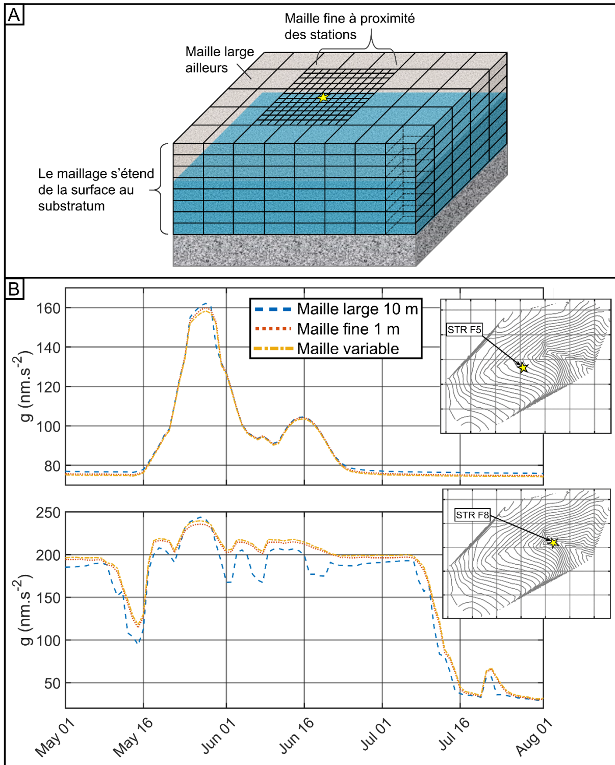
Figure 5.3 Recherche du maillage gravimétrique optimal. A) Schéma du maillage gravimétrique à pas variable, avec des mailles fines à proximité des stations gravimétriques et des mailles plus lâches ailleurs. B) Graphe du haut : Gravité calculée à la station STR F5 à partir du modèle NIHM13667 à un pas journalier en utilisant un maillage gravimétrique avec un pas fixe de 10 m (tirets bleus), un maillage fin avec un pas fixe de 1 m (pointillés rouges) et avec un maillage à pas variable (1 m à proximité des stations et 10 m ailleurs). B) Graphe du bas : Gravité calculée à la station STR F8.
