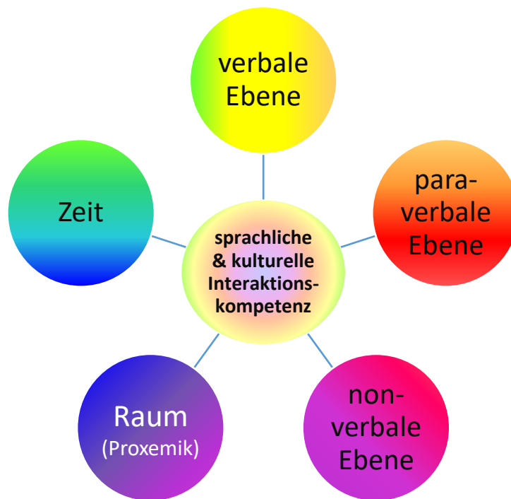
Abbildung 27: Beobachtungsrelevante Aktionsebenen
