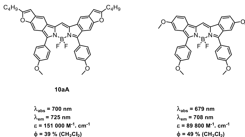
Figure 2-32 Comparaisons des propriétés spectroscopiques de 10aA et du BODIPY tétraméthoxy
