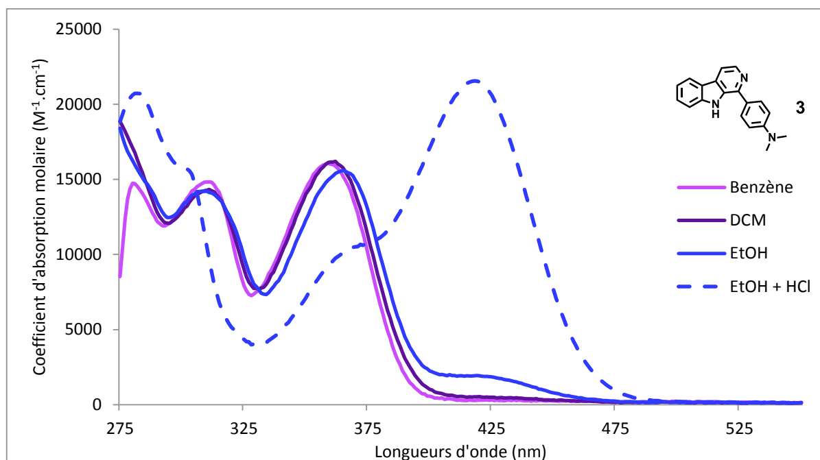
Figure 3-15 Spectre d'absorption du composé 3 enregistrés dans différents solvants
