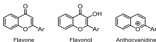
Figure 2-50 Structures des principaux flavonoïdes
