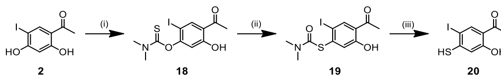
Figure 2-41 Schéma de synthèse du produit 20
