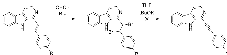
Figure 3-24 Synthèse envisagée pour la synthèse des dérivés ethynyles
