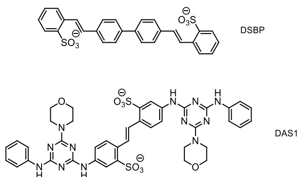
Figure 1-25 Structures de deux azurants optiques utilisés dans la lessive. Le DAS1 (pour 4,4'-bis[4-anilino-6-morpholino-1,3,5-triazin-yl]amino]stilbène-2,2'-disulfonate) et le DSBP (pour 4,4'-bis(2-sulfostyryl)biphényl)
