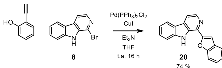
Figure 3-40 Schéma de synthèse de la molécule 20
