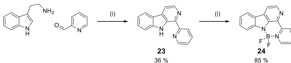
Figure 3-45 Schéma de synthèse du complexe de bore 24
