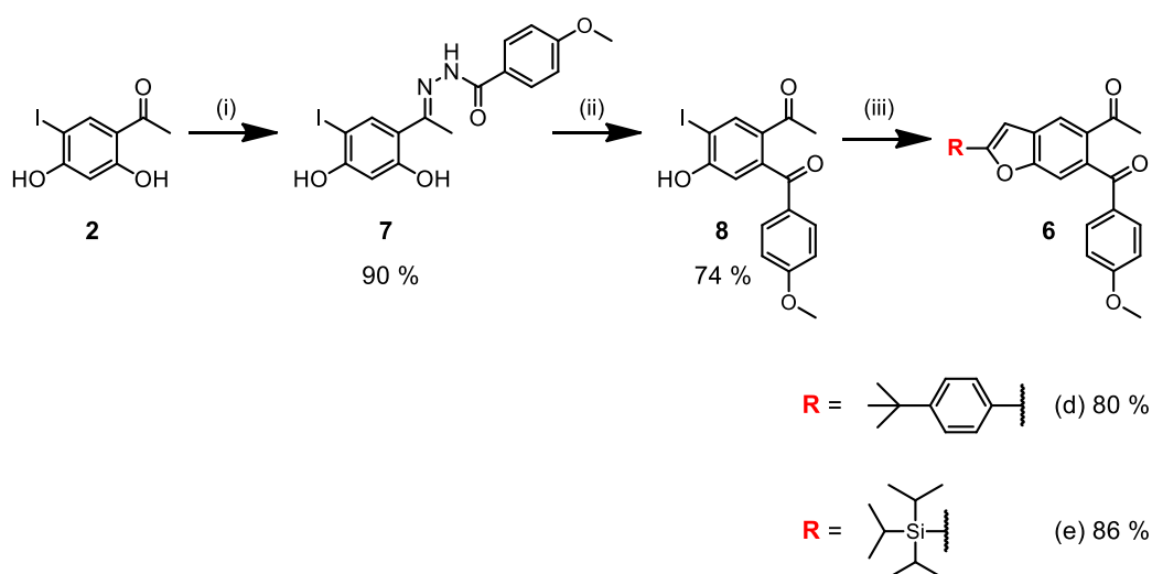
Figure 2-26 Voie de synthèse alternative du composé 6 réactif et conditions : (i) \text{PrOH} , \text{AcOH}_{\text{cat}} , 100 °C, 16h ; (ii) \text{Pb}(\text{OAc})_4 , THF, T.A., 2h ; (iii) \text{Et}_3\text{N} , \text{Pd}(\text{PPh}_3)_2\text{Cl}_2 , \text{CuI} , THF, T.A., 16h.
