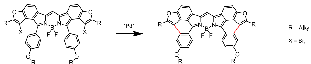
Figure 2-38 Perspectives d'un couplage de Heck intramoléculaire
