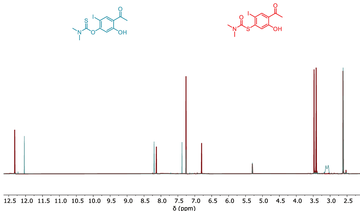
Figure 2-43 Superposition des spectres RMN 1 H (400 MHz, CDCl 3 ) des composés 18 et 19
