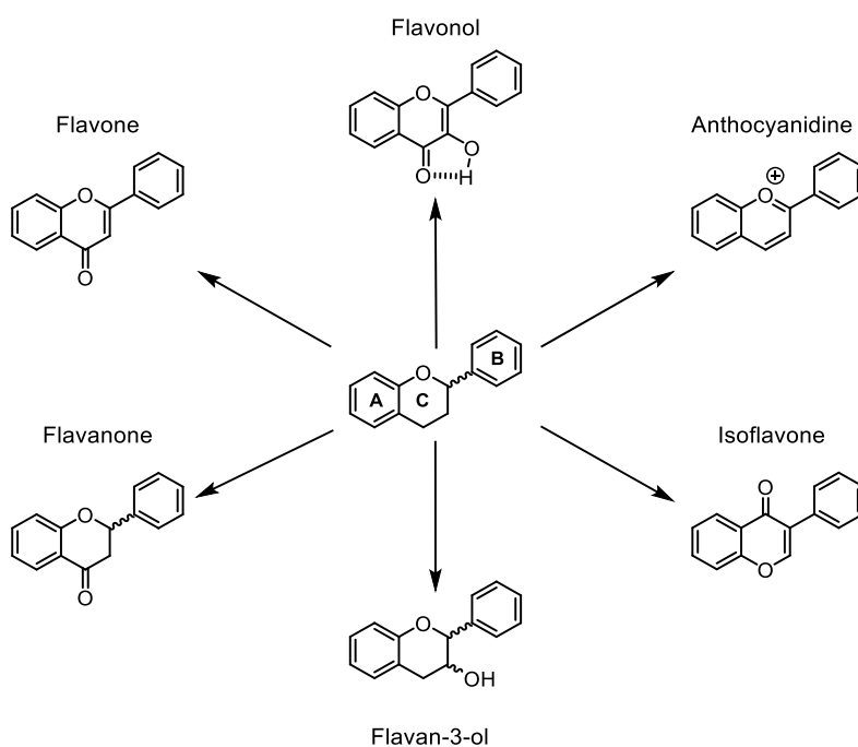
Figure 1-29 Structures des principaux flavonoïdes
