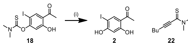
Figure 2-45 Schéma réactionnels du couplage de Sonogashira sur le composé 18 Réactifs et conditions : (i) : hexyne, \text{Et}_3\text{N} , \text{Pd}(\text{PPh}_3)_2\text{Cl}_2 , hexyne, \text{CuI} , THF, T.A., 16h.
