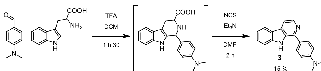
Figure 3-13 Schéma de synthèse du composé 3
