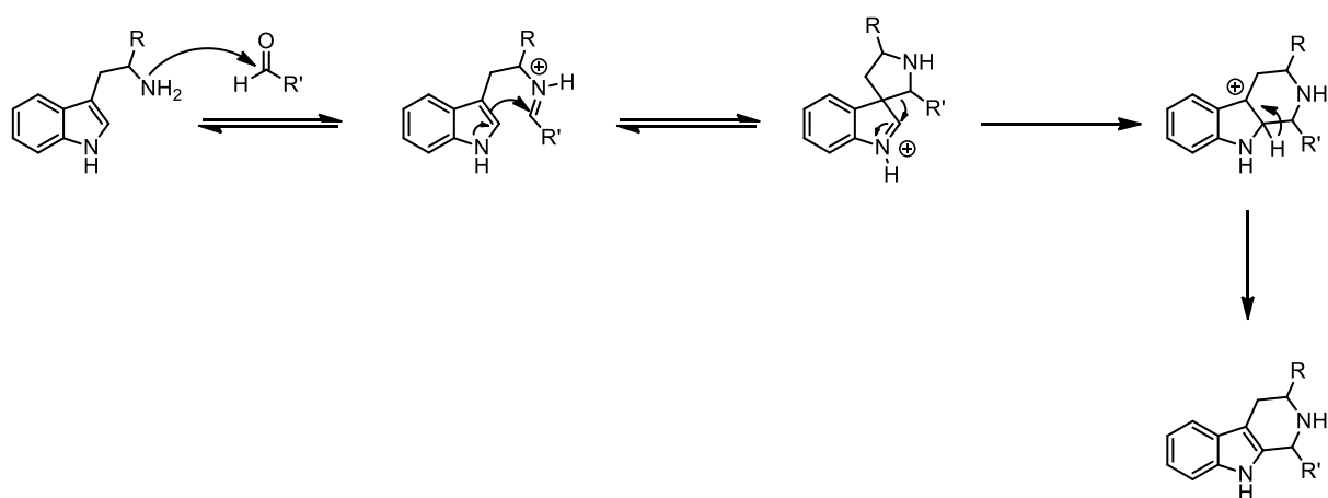
Figure 3-6 Mécanisme de la réaction de Pictet-Spengler
