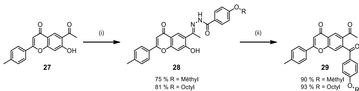
Figure 2-54 Schéma de synthèse des dicétones 29 réactifs et conditions : (i) \text{PrOH} , \text{AcOH}_{\text{cat}} , 100^\circ\text{C} , 16\text{h} ; (ii) \text{Pb}(\text{OAc})_4 , \text{THF} , T.A., 2\text{h}
