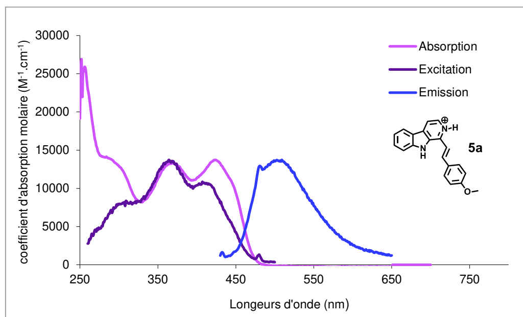
Figure 3-21 Spectres d'absorption, d'émission et d'excitation du composé 5a dans le DMSO avec TFA
