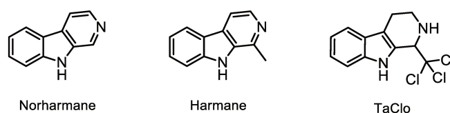
Figure 3-3 Structure de différentes \beta -carbolines
