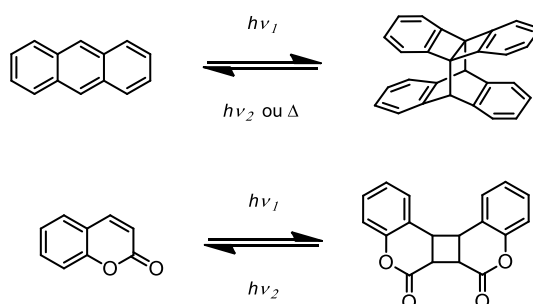
Figure 1-14 Exemples de dimérisation photoinduite
