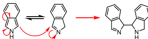
Figure 2-8 Mécanisme de polymérisation des isoindoles
