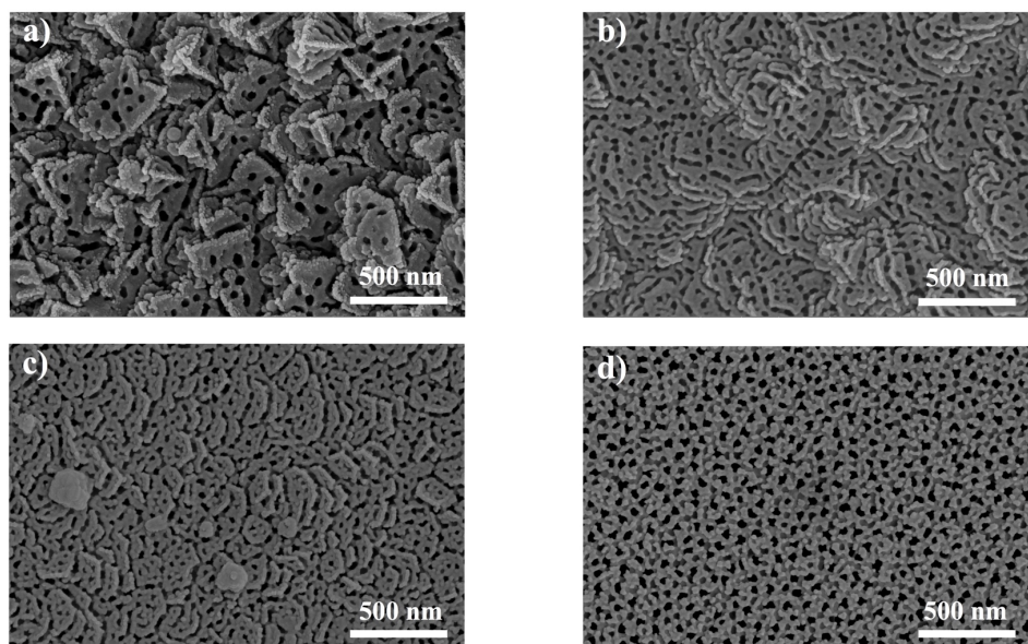
Figure 31 : Images MEB après anodisation électrochimique de la surface d'échantillons pour lequel le film de titane est déposé à des vitesses différentes (a) : 4,54 \text{ \AA/s} , (b) : 8,26 \text{ \AA/s} , (c) : 11,12 \text{ \AA/s} et (d) : 12,72 \text{ \AA/s} .
