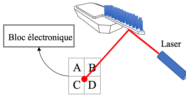
Figure 86 : Principe de lecture de la fréquence de résonance.
