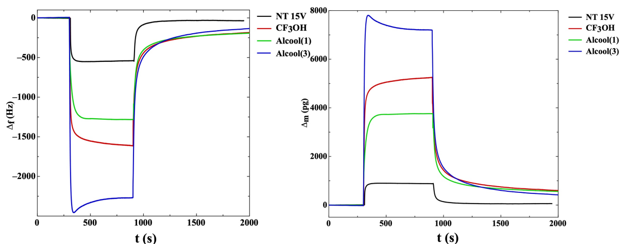
Figure 104 : Évolution de la fréquence de résonance et de la masse adsorbée des microleviers TL-NCL dont les deux faces (DN) sont recouvertes par des nanotubes de \text{TiO}_2 (15V, 900s) fonctionnalisés avec des molécules donneuses de liaisons hydrogène lorsqu'ils sont soumis pendant 10 minutes à un flux d'air contenant 594 ppm de DMMP. Les molécules greffées sont (Alcool(1) en vert, Alcool(3) en bleue et \text{CF}_3\text{OH} en rouge).
