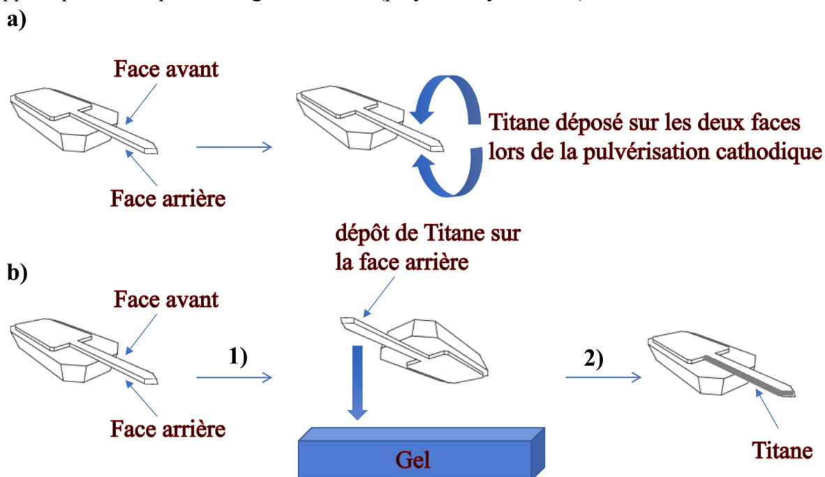
Figure 47 : Méthode de dépôt sur une seule face, (a) Problème observé lors du dépôt de titane par pulvérisation cathodique, (b) méthode de dépôt sur la face arrière d'un microlevier.
