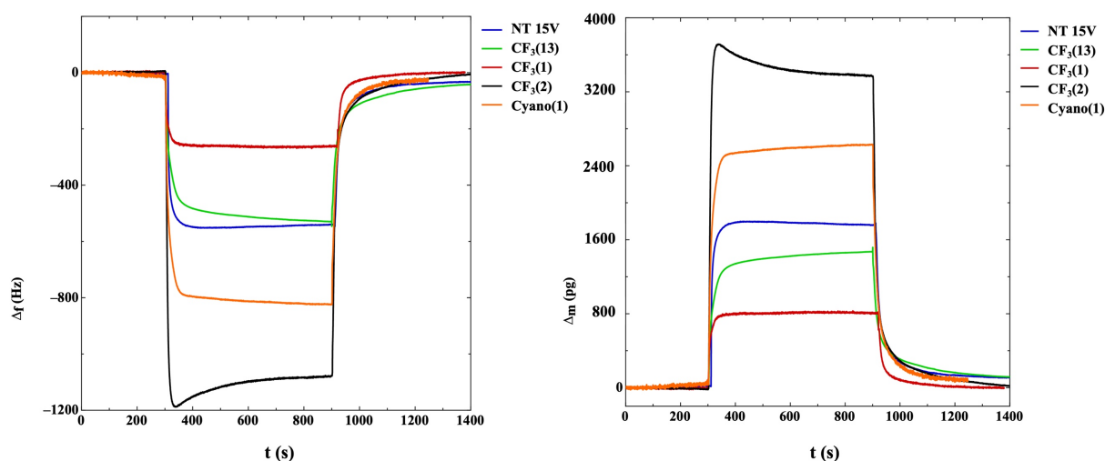
Figure 102 : Evolution de la fréquence de résonance et de la masse d'un microlevier TL-NCL dont les deux faces (DN) sont recouvertes par des nanotubes de \text{TiO}_2 (15V, 900s) et fonctionnalisés avec des molécules acceptrices de liaisons hydrogène ( \text{CF}_3(13) en vert, \text{CF}_3(1) en rouge, \text{CF}_3(2) en noire et Cyano(1) en orange), lorsqu'il est soumis pendant 10 minutes à un flux d'air contenant 594 ppm de DMMP.
