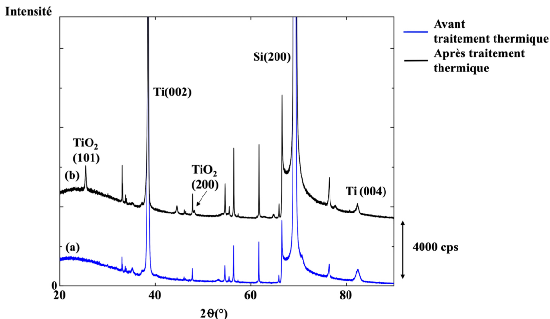
Figure 42 : (a) Diffractogramme de rayons X d'un substrat anodisé dans les conditions B, (b) Diffractogramme de rayons X du même échantillon recuit à 450^\circ\text{C} sous air.
