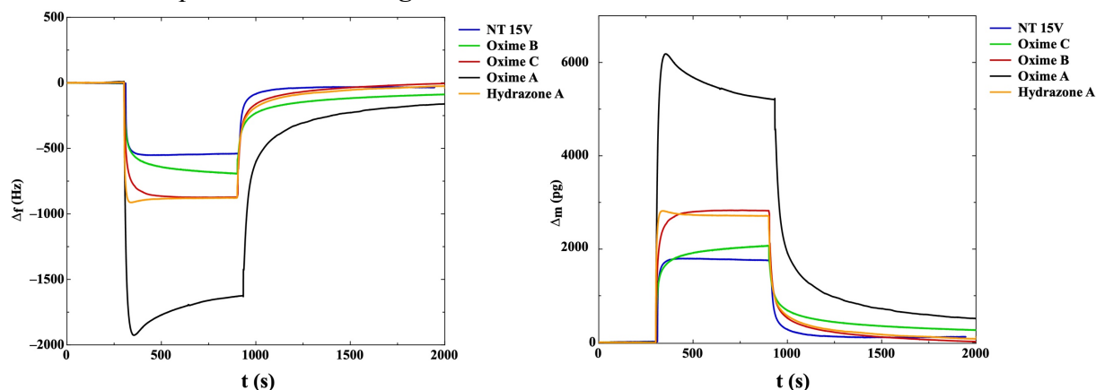
Figure 108 : Évolution de la fréquence de résonance et de la masse d'un microlevier TL-NCL dont les deux faces (DN) du microlevier sont recouvertes par des nanotubes de \text{TiO}_2 (15V,900s) fonctionnalisés avec les oximes A, B et C et avec l'Hydrazone A lorsqu'il est soumis pendant 10 minutes à un flux d'air contenant 594 ppm de DMMP. A titre comparatif, les deux graphiques représentent également la variation de fréquence et de masse d'un levier nanostructuré et non fonctionnalisé soumis au même protocole.
