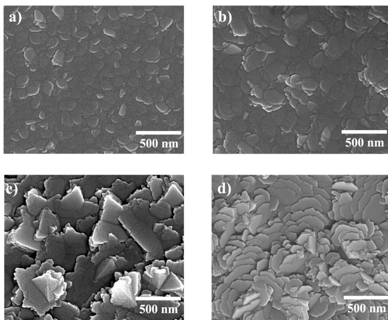
Figure 24 : Images MEB de la surface des échantillons obtenue pour une vitesse de dépôt de 4,55 Å/s. L'épaisseur de titane déposée est (a) 644 nm, (b) 1060 nm, (c) 2215 nm et (d) 4756 nm.
