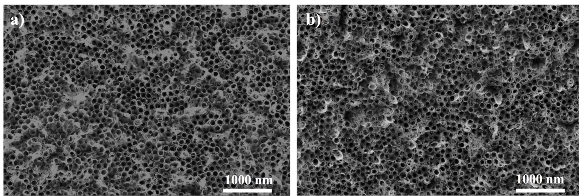
Figure 43 : Images MEB des nanotubes de \text{TiO}_2 (a) avant traitement thermique, (b) après traitement thermique à 450^\circ\text{C} sous air pendant 4 heures.
