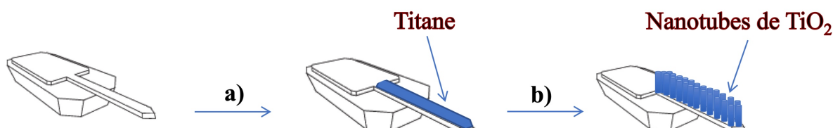
Figure 18 : Principe de la synthèse (a) : dépôt d'une couche de titane par pulvérisation cathodique, (b) : synthèse des nanotubes de \text{TiO}_2 par anodisation électrochimique.
