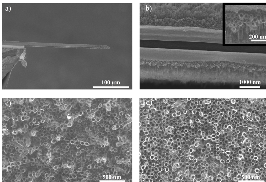
Figure 55 : Images MEB d'un microlevier dont une couche de titane est déposée sur la face avant à 60^\circ\text{C} et anodisé sur les deux faces (a) microlevier nanostructuré sur deux faces, (b) : zoom sur la tranche du microlevier, (c) : nanostructuration sur la face avant, (d) : nanostructuration sur la face arrière.
