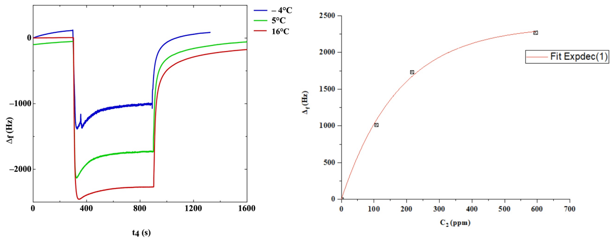
Figure 109 : Évolution de la fréquence de résonance d'un microlevier TL-NCL dont les deux faces (DN) du microlevier sont recouvertes par des nanotubes de \text{TiO}_2 (15V, 900s) et fonctionnalisé avec l'Alcool(3) lorsqu'il est soumis pendant 10 minutes à un flux d'air contenant 594, 216 et 107 ppm de DMMP. Traitement des chutes de la fréquence de résonance avec un algorithme de Levenberg-Marquardt.
