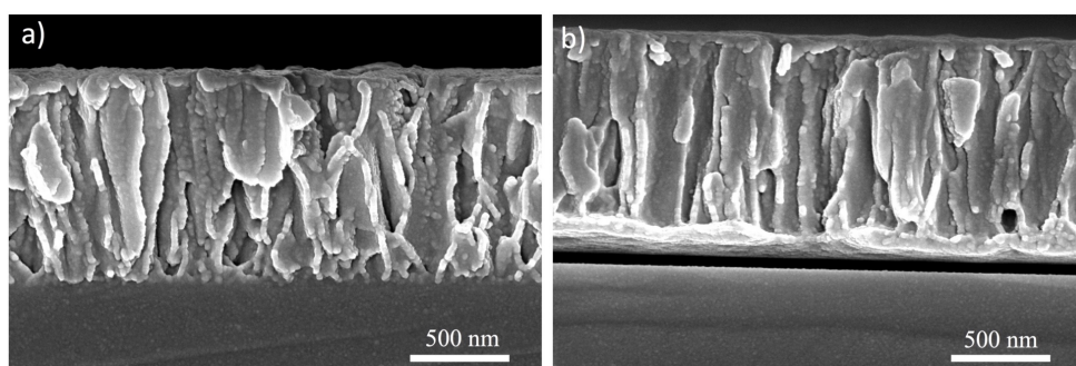
Figure 21 : Dépôts de titane par pulvérisation cathodique après modification du facteur de correction (135%) observés sur la tranche par MEB avec une puissance de déposition de (a) 4,83 \text{W}/\text{cm}^2 et (b) 9,65 \text{W}/\text{cm}^2 .
