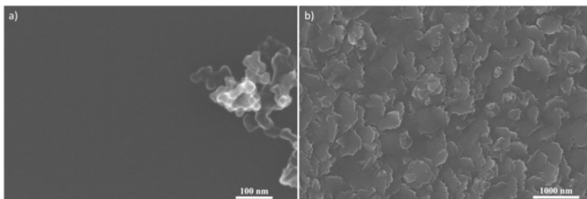
Figure 93 : Images MEB (a) d'un levier TL-NCL nu et (b) d'un levier TL-NCL recouvert d'une couche de 2,2 \mu\text{m} de titane déposé par pulvérisation cathodique et d'une couche superficielle de \text{TiO}_2 .
