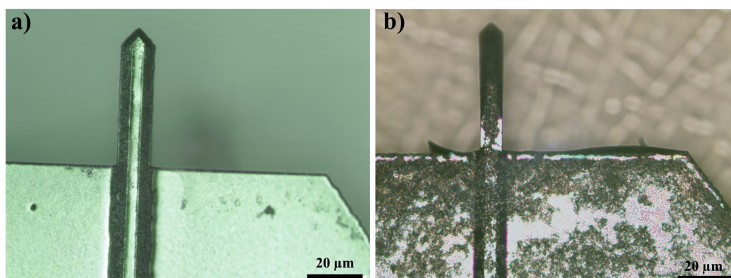
Figure 54 : Image par microscopie optique d'un levier dont une couche de titane déposé sur la face avant (a) à 60^\circ\text{C} et (b) à 25^\circ\text{C} a été anodisée.
