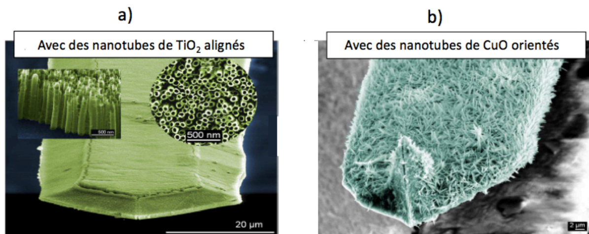
Figure 17 : (a) Microleviers nanostructurés avec un réseau de nanotubes de \text{TiO}_2 , (b) Microleviers nanostructurés avec un réseau de nanotubes de \text{CuO} .
