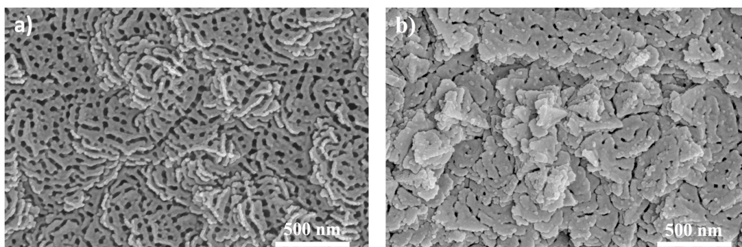
Figure 36 : Images MEB après anodisation (a) dans les conditions standard sans acide et (b) en présence d'acide phosphorique à une concentration ( 3 \cdot 10^{-2} mol), observées vue du dessus.
