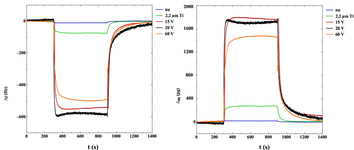
Figure 100 : Evolution de la fréquence de résonance et de la masse de trois microleviers TL-NCL recouverts par des nanotubes de \text{TiO}_2 (DN) et exposés pendant 10 minutes à 594 ppm de DMMP. Chacun des trois leviers a été soumis à une tension d'anodisation différente (15V, 20V, 60V) durant la synthèse des nanotubes.
