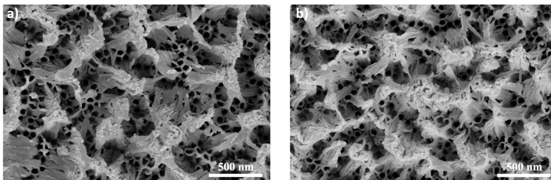
Figure 35 : Images MEB vue du dessus après anodisation à 45°C de deux substrats recouverts de 2 \mu\text{m} de titane dans une solution contenant (a) 0,5% en masse de \text{NH}_4\text{F} et (b) 0,75% en masse de \text{NH}_4\text{F} .
