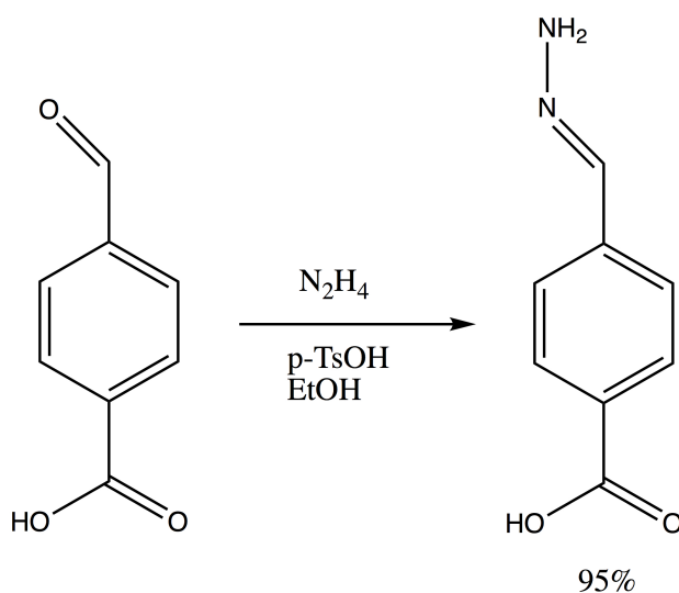
Figure 71 : Synthèse de l'hydrazone A.
