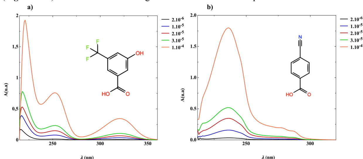
Figure 82 : Courbes d'étalonnage (a) pour la molécule avec une fonction alcool fluoré présentée en figure 15-3 pour une fenêtre spectrale de 215-355 nm et (b) pour la molécule avec une fonction cyano présentée en figure 16-5 pour une fenêtre spectrale de 215-320 nm.
