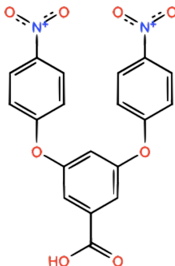
Figure 105 : Molécule constituée d'une fonction acide carboxylique utilisée pour le greffage sur la nanostructure de \text{TiO}_2 et deux fonctions nitro ( \text{NO}_2 ) comme sites actifs.
