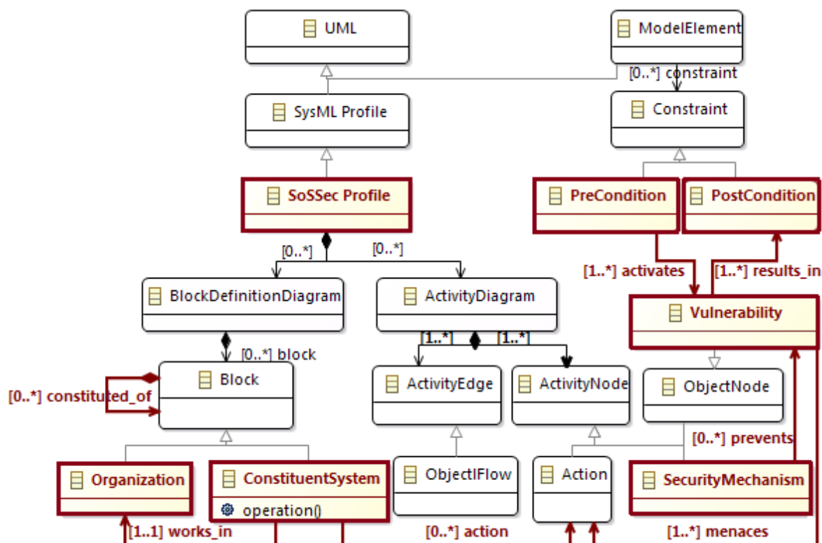
Fig. I.2.8 SoSSecML abstract syntax (MetaModel)
