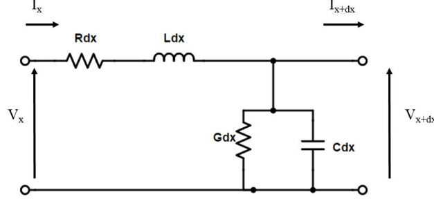
FIGURE E.2 – Element infinitésimal d'une ligne de transmission qui relie une source à une charge, appliquant le modèle à constantes réparties
