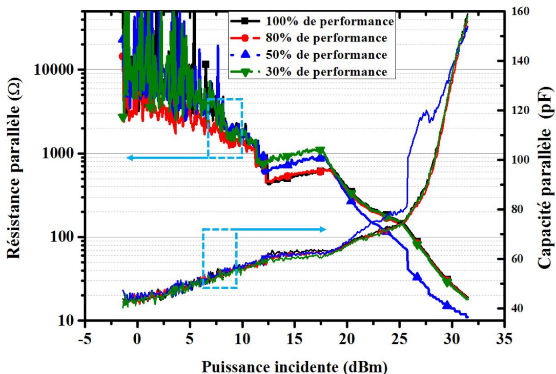
FIGURE 4.34 – Comparaison des impédances des puces implémentant différentes valeurs de gigahertz, donc ayant différentes performances
