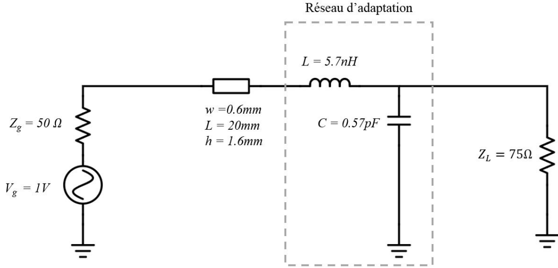
FIGURE E.12 – Schéma du circuit pour la comparaison entre formules de transfert de puissance
