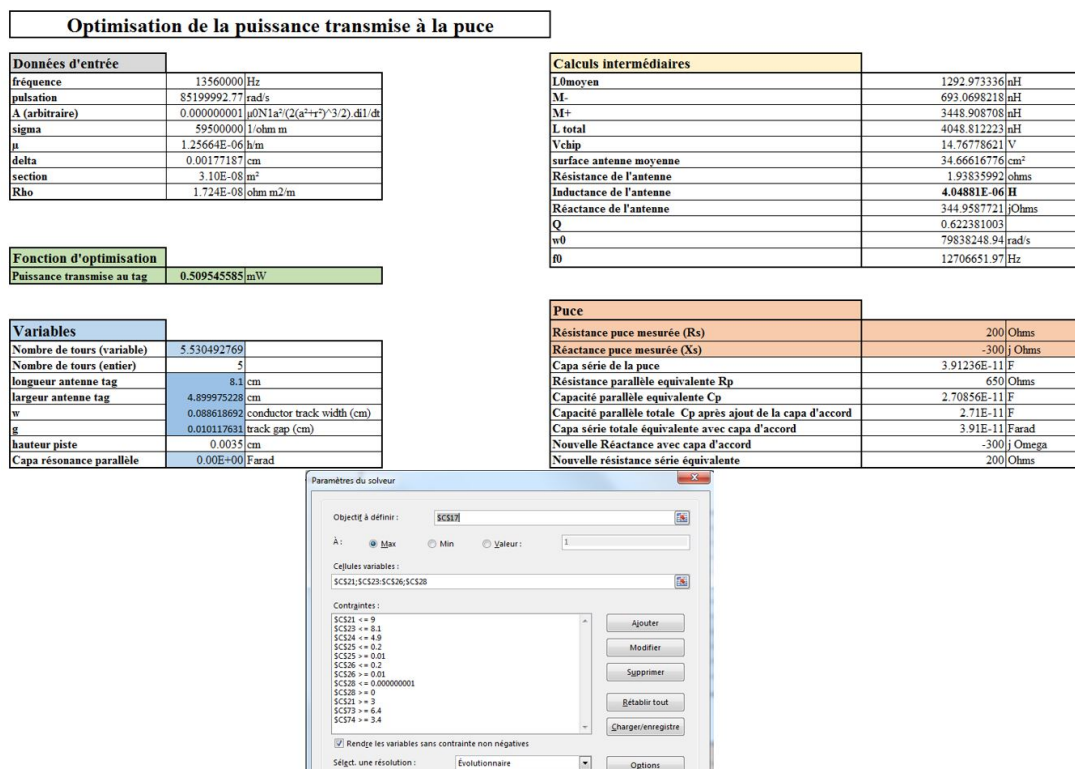
FIGURE 4.48 – Implémentation sous excel de l'optimisation de la puissance transmise à une puce. D'autres cellules contenant tous les calculs intermédiaires ne sont pas montrées faute de place
