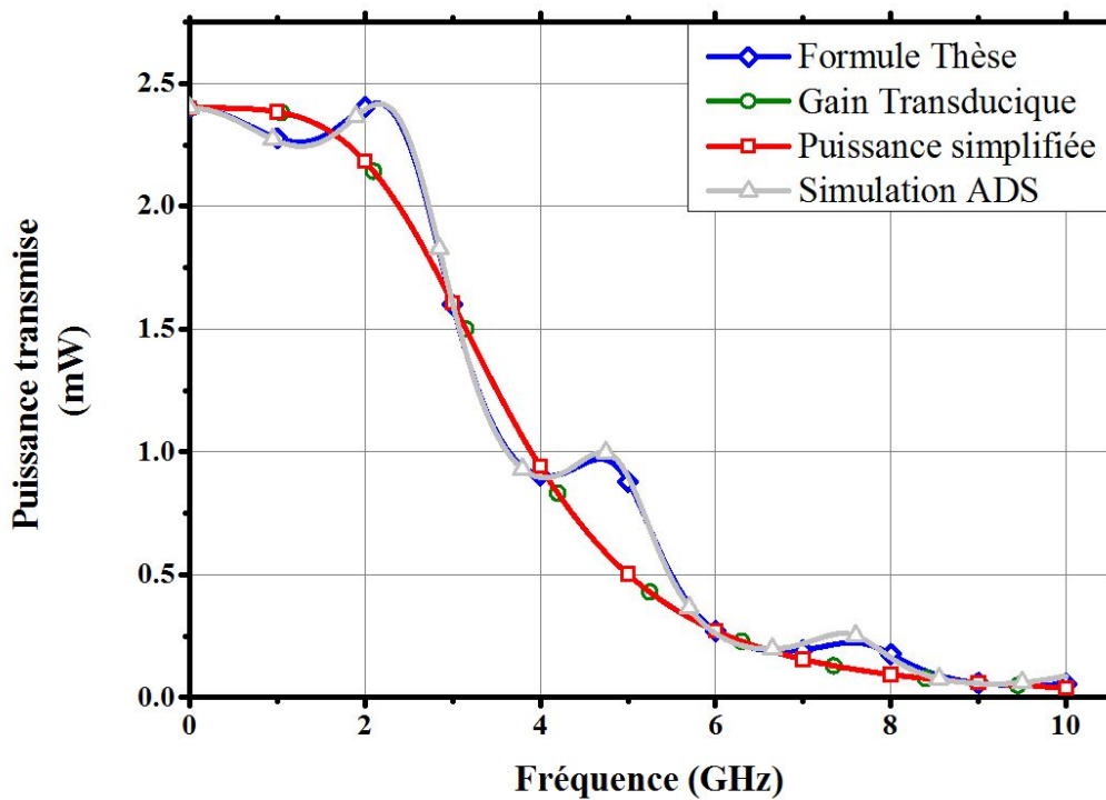
FIGURE E.14 – Comparaison entre les formules de calcul du transfert de puissance entre une source et une charge à travers un réseau d'adaptation et une ligne. Les courbes obtenues sont comparées à la grise issue de simulations ADS
