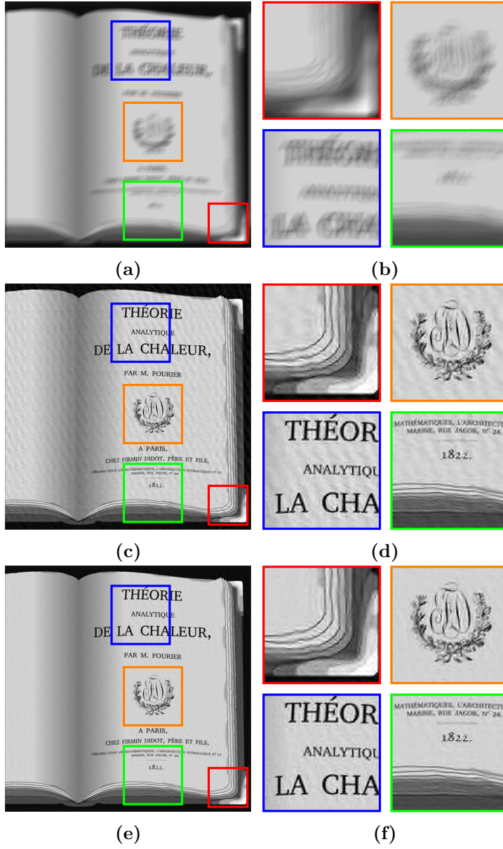
Figure 1.10 – Un exemple de déconvolution (1.45) montrant l'importance de la méthode de seuillage. En haut l'image dégradée avec un flou de mouvement et un bruit Gaussien i.i.d. de niveau 5.10^{-3} le \text{pSNR} = 17.85\text{dB} . Les deux matrices \Theta ont été construites avec le même nombre de coefficients (qui correspond à 57 opérations par pixels). Au milieu : la méthode de seuillage simple \text{pSNR} = 23.71\text{dB} . En bas : le seuillage pondéré (1.41), \text{pSNR} = 24.07\text{dB} . Au delà de l'augmentation du \text{pSNR} , on observe que les artefacts de restauration sont réduits significativement.
