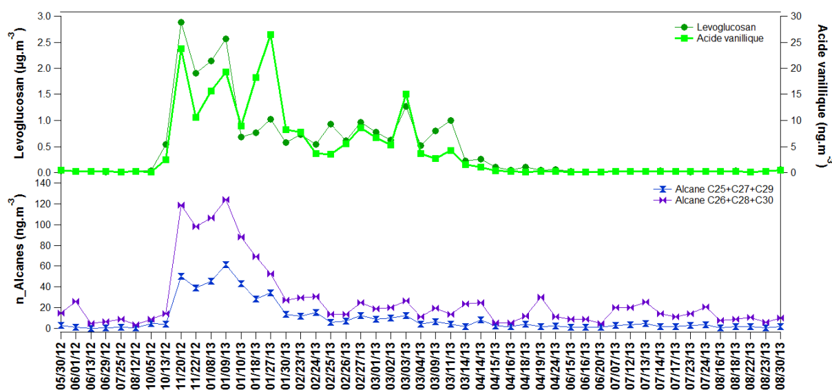
Figure III.7 : Evolution temporelle du levoglucosan, de l'acide vanillique, des alcanes impaire (C25-C27-C29) et des alcanes paire (C26-C28-C30).
