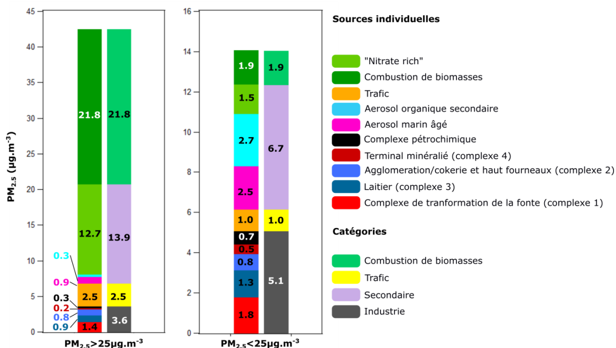
Figure III.15 : Contribution ( \mu\text{g.m}^{-3} ) des sources estimées avec le modèle ME-2 corrigé pendant ( n=17 ) et hors épisodes ( n=32 ) de PM 2.5 .
