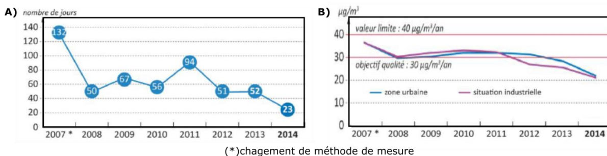
Figure I.13 : A) Evolution du nombre de jours avec au moins une station dépassant le seuil journalier de 50\mu\text{g.m}^{-3} pour les \text{PM}_{10} B) Evolution des moyennes annuelles en particules en suspension \text{PM}_{10} (AirPACA, 2014).
