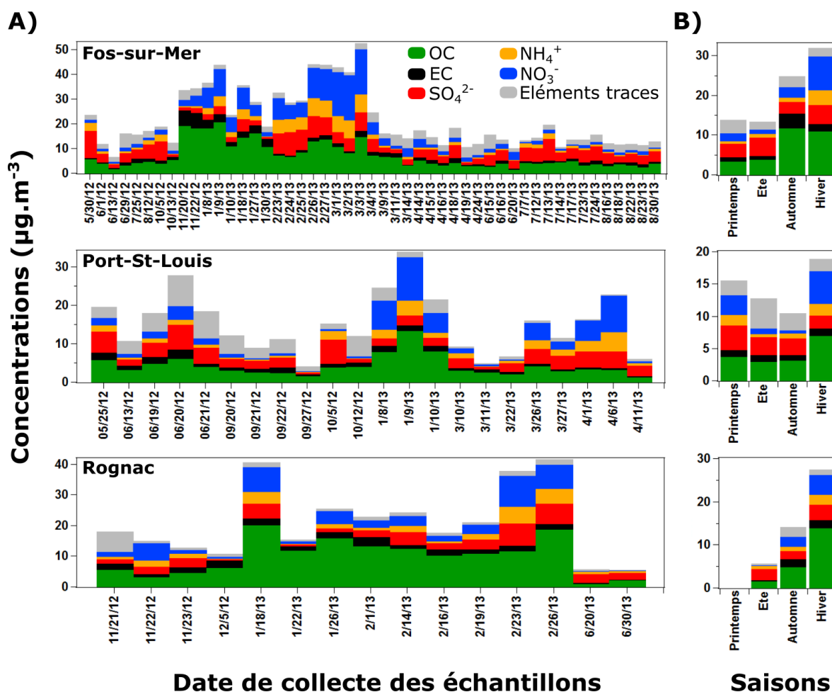
Figure III.6 : Composition des PM 2.5 A) séries temporelles (ensemble des échantillons analysés) B) variabilité saisonnière. Printemps : 20mars–20juin ; Eté : 20juin–22sep ; Automne : 22sep-20déc ; Hiver : 20déc-20mars.
