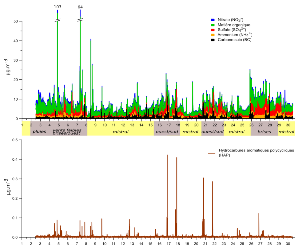
Figure I.17: Concentrations des principales fractions chimiques et des HAP dans les particules (PM 1 ) obtenues pour le site de Fos-sur-Mer en juin 2011 (Dron et al., 2015).
