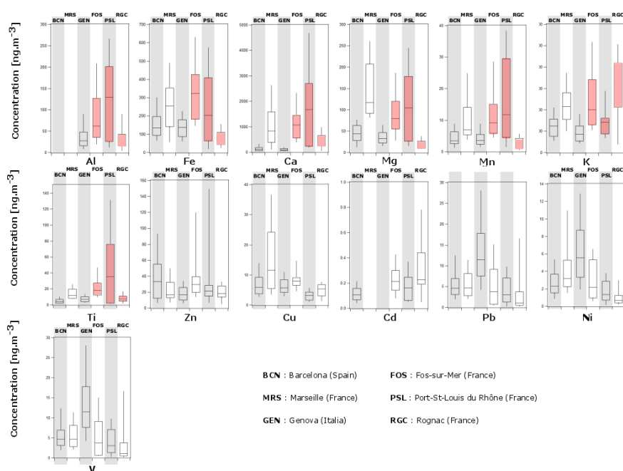
Figure III.8 : Concentration médianes des principaux éléments traces pour les trois sites: Fos sur Mer (FOS), Port Saint Louis (PSL) et Rognac (RGC) ; et comparaison avec 3 villes méditerranéennes (Barcelone, Marseille, Gènes) (Données 2011-2012, Salameh et al., 2015).
