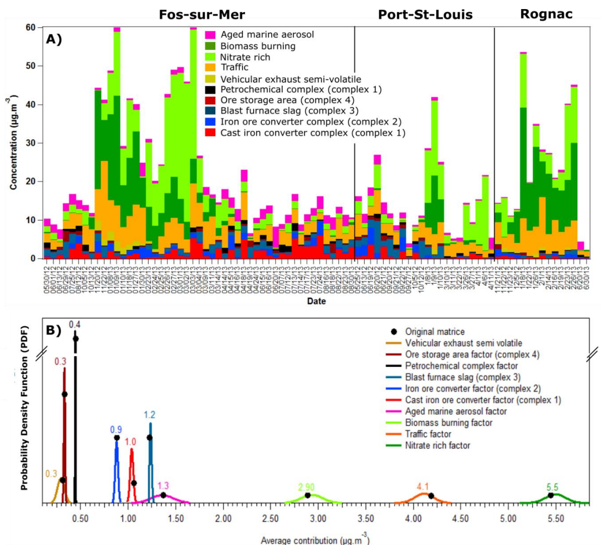
Figure III.11 : A. Evolutions temporelles des facteurs obtenus par l'approche ME-2 pour les trois sites d'étude ; B. Contribution moyenne des différents facteurs tous sites confondus. Les densités de probabilités sont établies en faisant varier aléatoirement 30 fois l'ensemble des variables de la matrice de données. L'incertitude analytique fixe les bornes hautes et basses du domaine de concentrations explorées pour chaque composé. Les marqueurs représentent le résultat pour la matrice d'origine.
