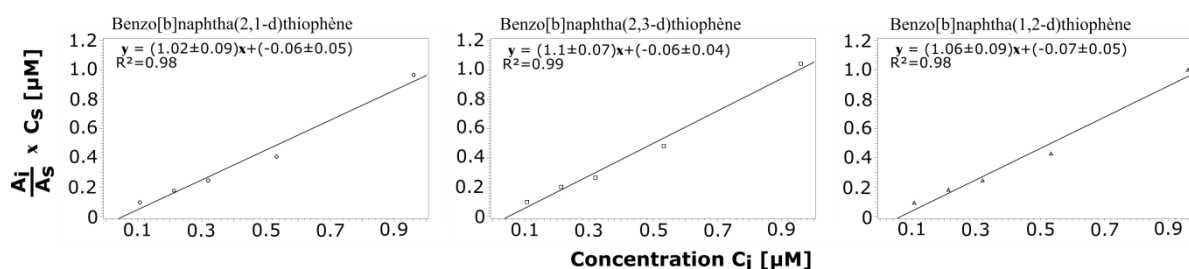
Figure II.15 : Gamme étalon pour les trois SHAP analysés. A_i et C_i sont respectivement la réponse et la concentration du composé, A_s et C_s , respectivement la réponse et la concentration (5µM) du standard interne.
