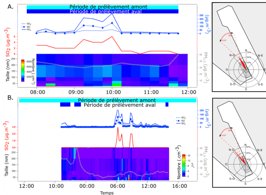
Figure II.5 : Exemple d'un couple d'échantillon « amont/aval » A. Sélectionné (14/12/2013) B. Non sélectionné (13-14/12/2013) pour le site du terminal minéralier. La couleur « bleu ciel » et « bleu foncé » représente, respectivement, les périodes durant lesquelles, l'échantillon amont et aval ont été prélevés
