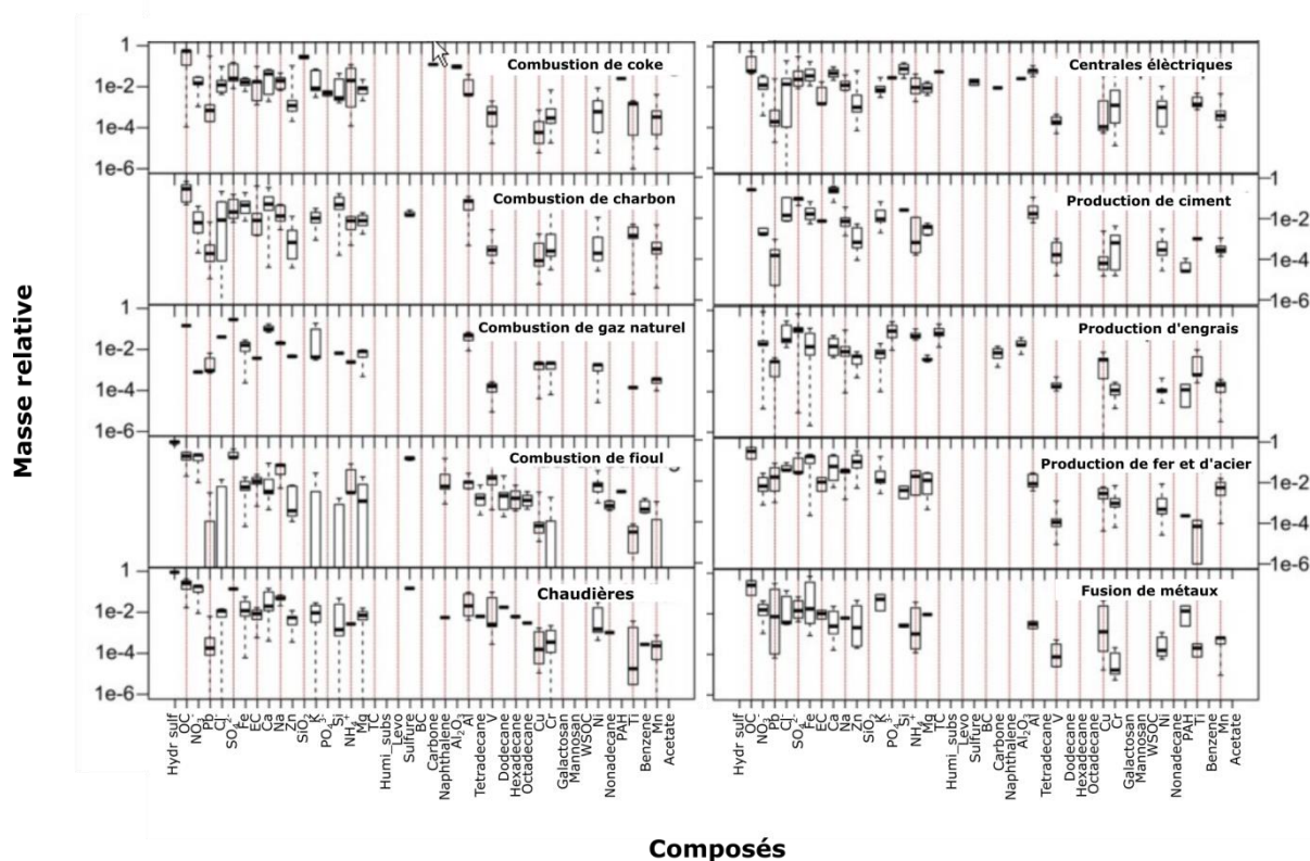
Figure I.8 : Distributions statistiques des 43 espèces chimiques les plus abondantes (par ordre d'abondance décroissant) dans les profils industriels regroupés par catégories (Pernigotti et al., 2016).
