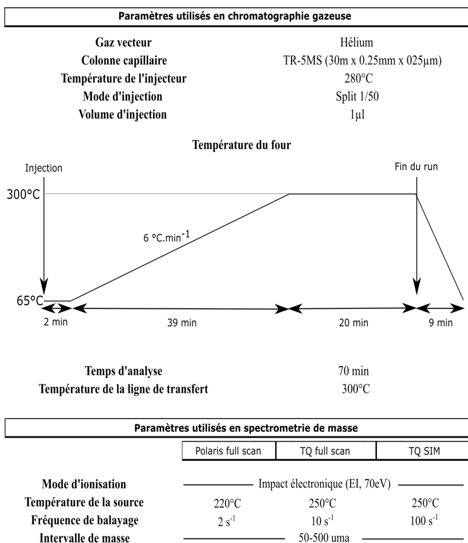
Figure II.12 : Paramètres analytiques utilisés pour les analyses de la spéciation chimique de l'aérosol en GC/MS.
