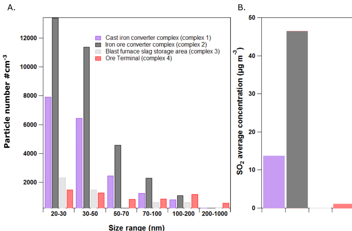
Figure III.1 : A) Nombre moyen de particule en fonction de la taille (UPF) et B) Concentration moyenne en SO 2 observées sur le site aval pour chaque complexe industriel durant le prélèvement des échantillons.
