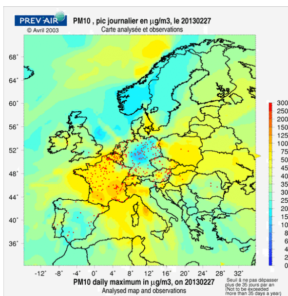
Figure III.14 : Modélisation analysée Prev'Air et observations pour les PM 10 , le 27 février 2013 ( http://www.prevair.org/ )
