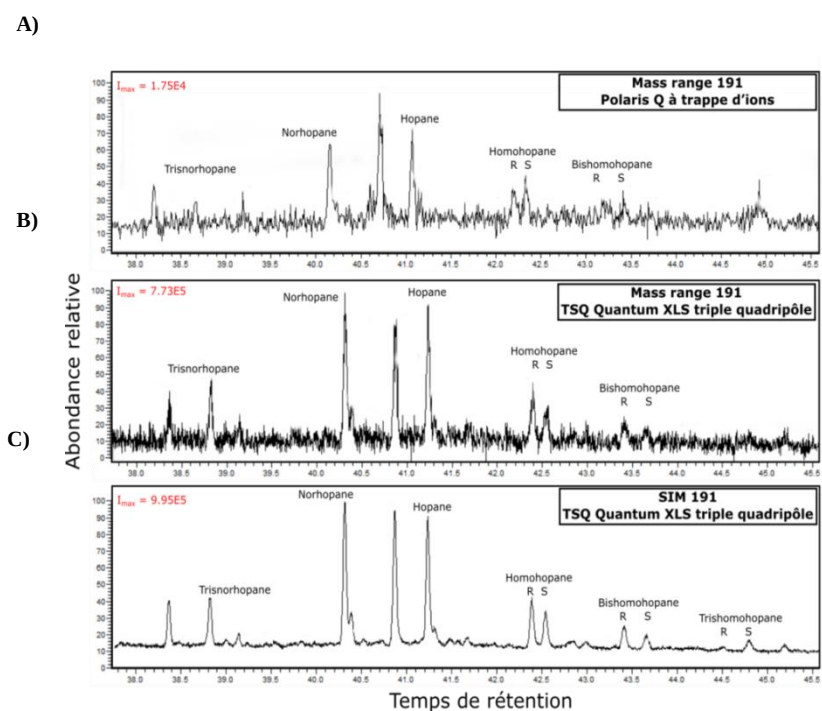
Figure II.11 : Exemple de chromatogramme pour un échantillon prélevé sur le site de Port-St-Louis du Rhône en hiver. Avec les deux systèmes analytiques en mode : A) Chromatogramme des hopanes avec le polaris en mode « mass range » (appel d'ion), B) Chromatogramme des hopanes avec le tiple quadripôle en mode « mass range » et C) Chromatogramme des hopanes avec le tiple quadripôle en mode « SIM »
