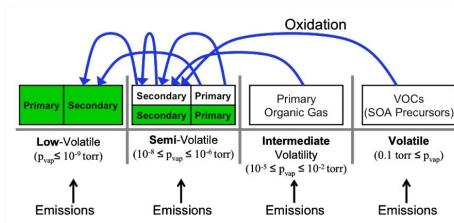
Figure I.3 : Schéma d'émission et d'évolution de l'OC dans l'atmosphère. Les cases de couleur verte représentent la phase particulaire (Fuzzi et al., 2015).
