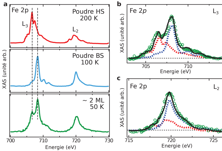
Figure XI. – Coexistence des états haut et bas spin des molécules de Fe-phen révélée par des mesures d'absorption des rayons X sur le seuil du fer. a , Spectres XAS mesurés sur de la Fe-phen massive dans l'état haut spin (panneau du haut), dans l'état bas spin (panneau du milieu) et sur un échantillon de 2 ML de Fe-phen déposées sur un substrat de Cu(100). Reproduction du seuil b , L_3 et c , L_2 du fer du spectre obtenu pour l'échantillon de 2 ML de Fe-phen à partir des spectres de référence obtenus sur la Fe-phen massive.
