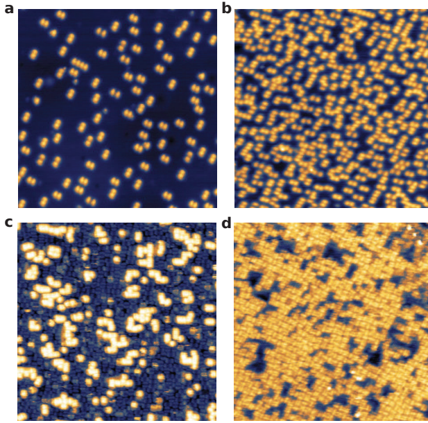
Figure VIII. – Croissance couche par couche de molécules de Fe-phen sur une surface de Cu(100). Topographies obtenues pour des taux de recouvrement de a 0.1 ML, b 0.4 ML, c 1.4 ML and d 1.8 ML. Les images ont une taille de 40 nm \times 40 nm.
