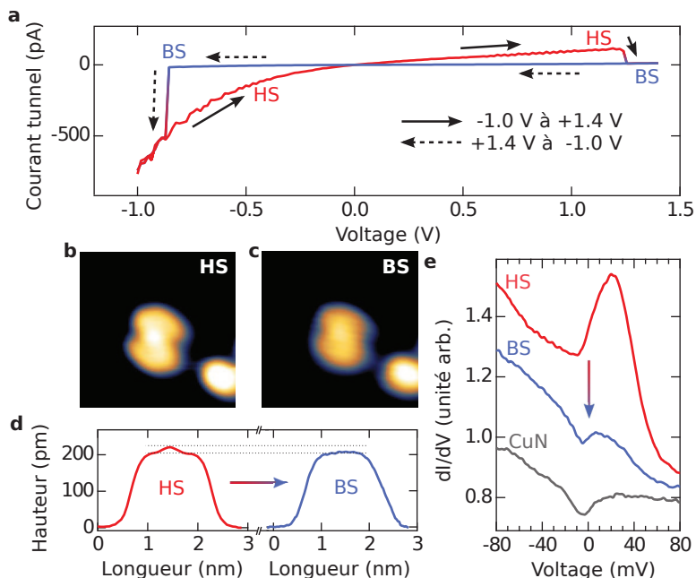
Figure XIII. – Commutation de l'état de spin et l'état de conductance d'un molécule de Fe-phen sur une surface de CuN/Cu(100). a , Courbe I(V) mesurée sur une molécule unique. La courbe montre deux états de conductance avec une hystérèse. Topography de la molécule sondée lorsqu'elle est dans l'état de b , haute conductance et c , basse conductance. Les topographies suggèrent que la molécule est dans b , l'état haut spin et c , l'état bas spin, respectivement. d , Profils de hauteur de la molécule représentée dans les topographies b et c . e , Spectres dI/dV de la molécule lorsqu'elle est dans l'état de haute et basse conductance. Toutes ces données permettent d'attribuer l'état de haute conductance (basse conductance) à l'état haut spin (bas spin). Les images ont une taille de 3.7 \text{ nm} \times 3.7 \text{ nm} .
