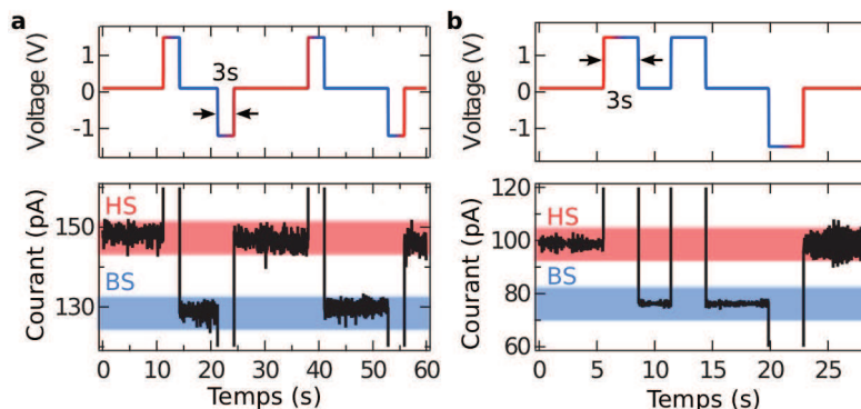
Figure XIV. – Commutation de l'état de spin d'une molécule de Fe-phen induite par une impulsion de tension. a, Série d'impulsion de tension appliquée sur la molécule en fonction de temps et le courant tunnel correspondant. L'état de spin de la molécule peut être commuté par l'application d'une impulsion de tension et la conductance de la jonction permet de lire l'état de spin. b, Expérience similaire à celle présentée en a qui montre l'importance de la polarité du pulse.
