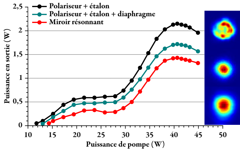
FIG. A.8 : Puissance en sortie à 1617 nm en fonction de la puissance de pompe incidente, pour trois cavités différentes. À droite, profils spatiaux du faisceau.
