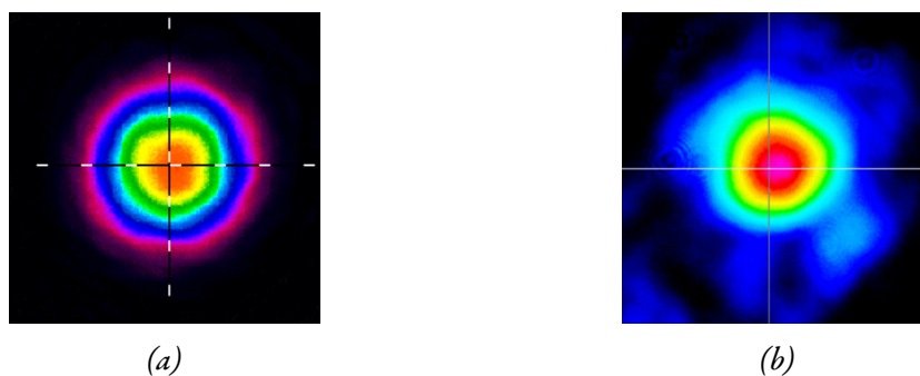
FIG. 3.4 : Profils transmis par une fibre cristalline de diamètre 800 \mu\text{m} (a) et 400 \mu\text{m} (b) d'un faisceau gaussien à 900 nm. La longueur des fibres cristallines est de 30 mm.
