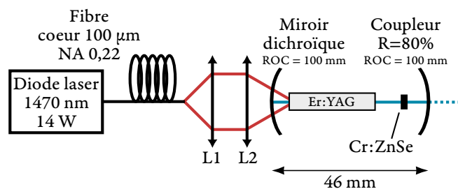
FIG. 3.13 : Représentation schématique de la source laser à cavité courte, pompée à 1470 nm et déclenchée passivement.
