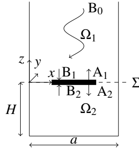
FIGURE 2.14 – Ligne microruban
