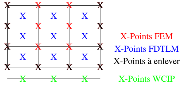
FIGURE 2.13 – Nombre d'inconnues.
