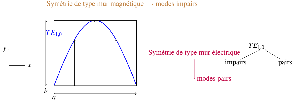
FIGURE 3.3 – Symétries dans le guide.
