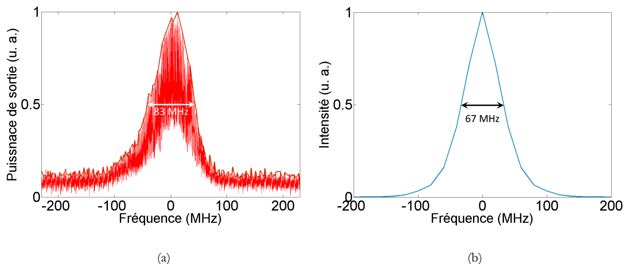
Figure 4- 26 : Caractérisation spectrale des impulsions QS du laser DFB monomode longitudinal avec [BDN] = 6 \times 10^{22} \text{ m}^{-3} pour un guide de largeur de diffusion W = 2,5 \text{ } \mu\text{m} . a) Interférogramme mesuré à l'analyseur FP et son enveloppe calculée. b) Calcul de la FFT d'une impulsion laser mesurée.
