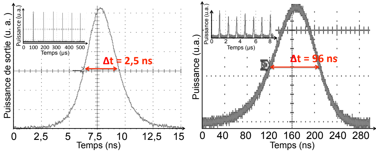
Figure 4- 21 : Traces temporelles du laser DFB avec un réseau de Bragg de profondeur 80 nm pour des concentrations en absorbant saturable [\text{BDN}] = 4,2 \times 10^{23} \text{ m}^{-3} (à gauche), et [\text{BDN}] = 1,2 \times 10^{22} \text{ m}^{-3} (à droite).
