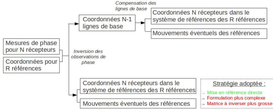
FIGURE 2.3 – Différentes stratégies de mise en référence.
