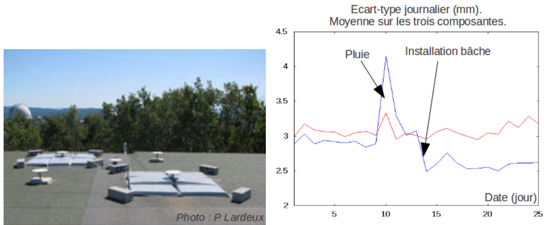
FIGURE 2.25 – Étude de l'effet de l'environnement sur l'amplitude des multitrajets.
