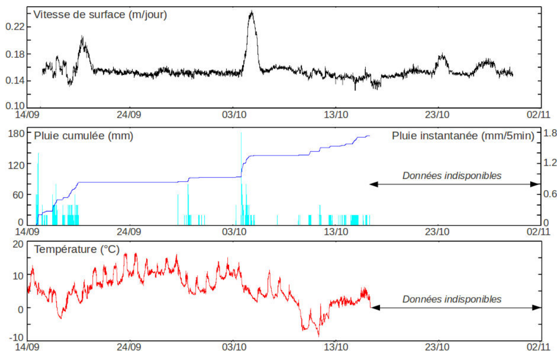
FIGURE 3.23 – Variations temporelles de la vitesse de surface du glacier d’Argentière et leur corrélation avec des paramètres météorologiques.
