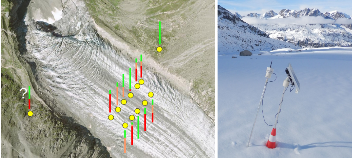
FIGURE 3.17 – Fonctionnement des Geocubes sur le glacier d'Argentière. Gauche : Bilan du fonctionnement ; vert : fonctionnement correct, orange : récepteur incliné, rouge : dysfonctionnement ou absence de données (fond de carte : geoportail.fr). Droite : Cas de dysfonctionnement : Geocube incliné et panneau solaire dos au soleil.
