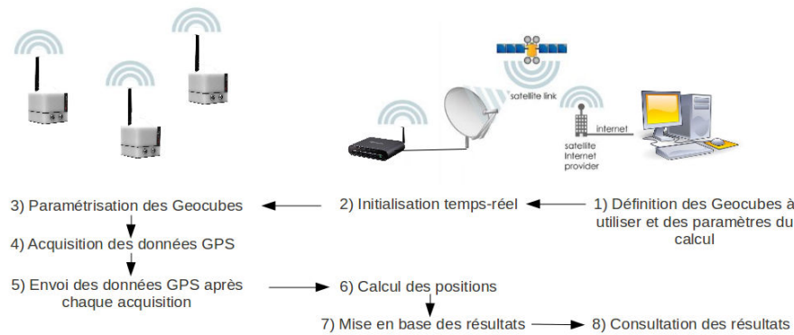
FIGURE 2.11 – Fonctionnement du positionnement en temps-réel.
