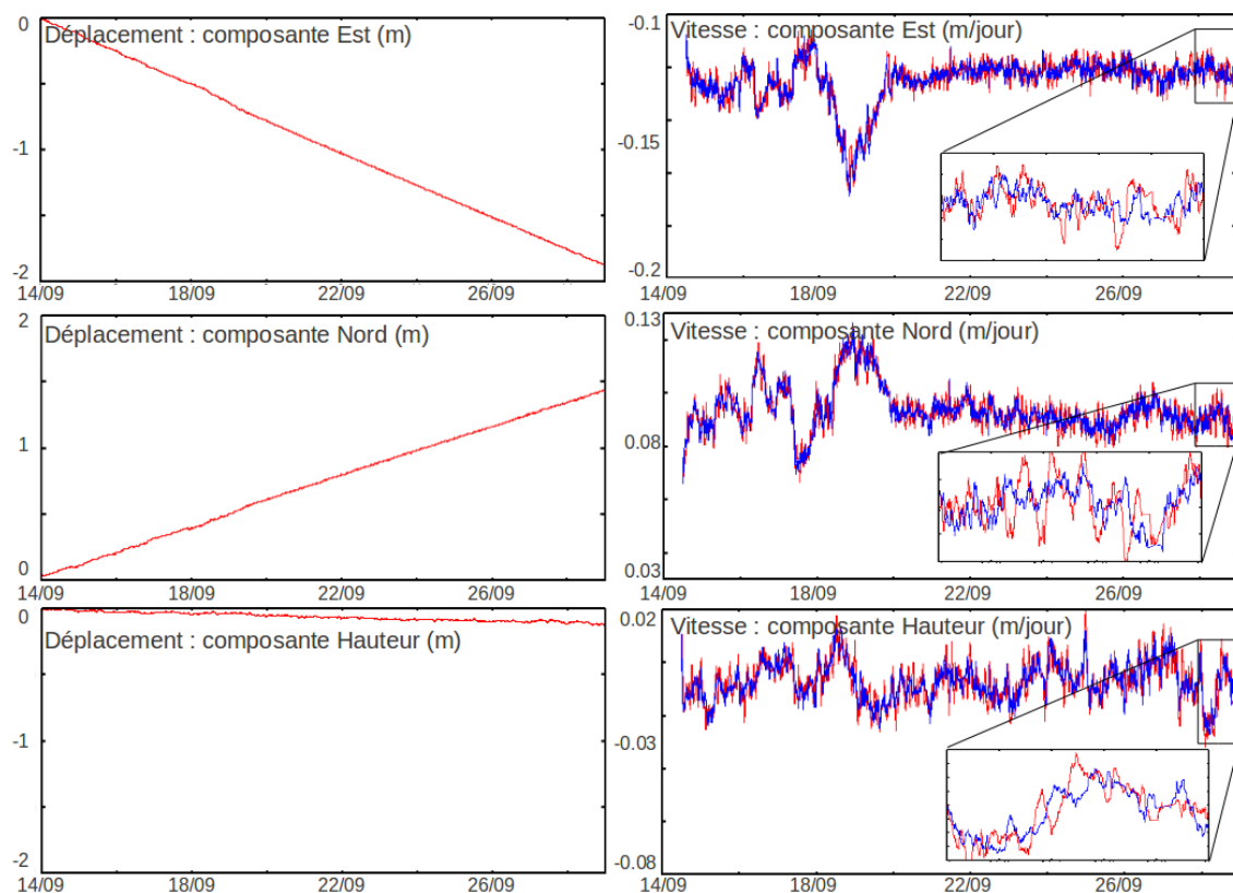
FIGURE 3.19 – Séries temporelles de positions (gauche) et de vitesse (droite) pour un récepteur placé sur le glacier.
