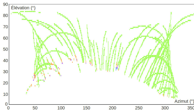
FIGURE 2.29 – Carte de résidus. Vert : résidu faible, orange : résidu modéré, violet : résidus élevés.
