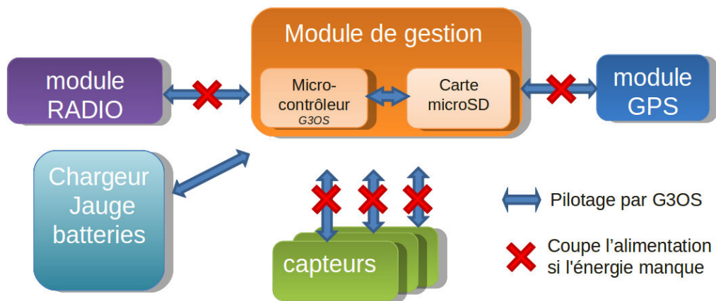
FIGURE 1.9 – Fonctionnement du module de gestion (illustration : O.Martin).
