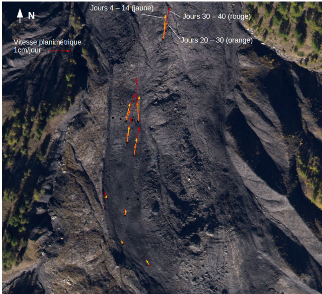
FIGURE 3.10 – Variations spatio-temporelles de la vitesse de glissement.
