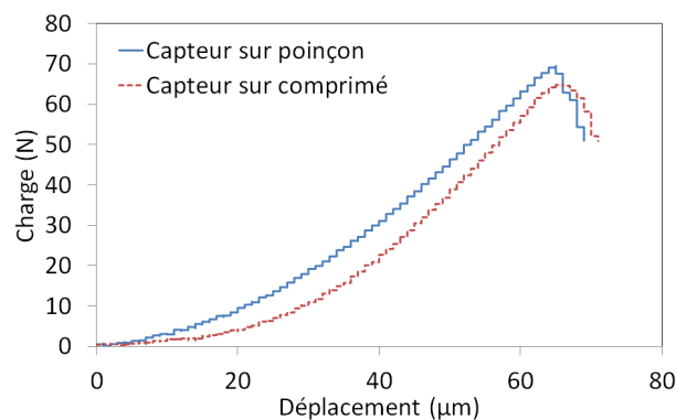
Figure 3.17 – Courbes de charge-déplacement de deux comprimés de granulés G160-500μ mis en forme à 300 MPa : pour l'un le capteur est placé sur le poinçon supérieur, pour l'autre le capteur est directement placé au contact du comprimé.
