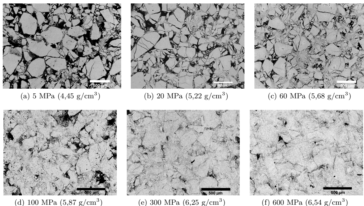
Figure 4.4 – Micrographies de comprimés crus de granulés G160-500μ compactés à : a) 5 MPa, b) 20 MPa, c) 60 MPa, d) 100 MPa, e) 300 MPa, f) 600 MPa.
