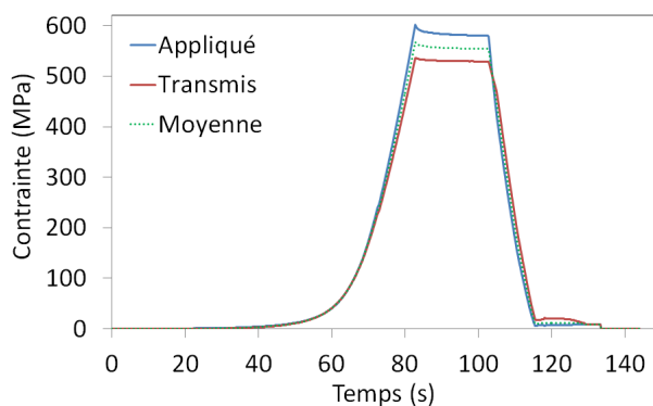
Figure 2.13 – Evolution des contraintes appliquée, transmise et moyenne lors de la compaction de granulés G160-500 \mu avec une hauteur de chambre de 12 mm.
