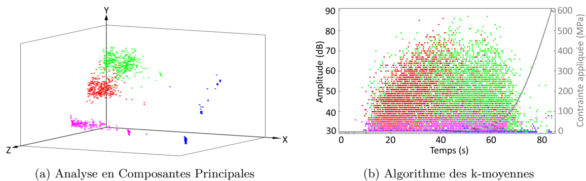
Figure 3.45 – Familles de salves déduites de l'analyse en composantes principales des données d'EA acquises lors de la compaction de granulés G160-500 \mu à la vitesse de compression 0,1 mm/s : a) représentation 3D dans un espace non physique, b) représentation des salves en amplitude au cours de la compaction.
