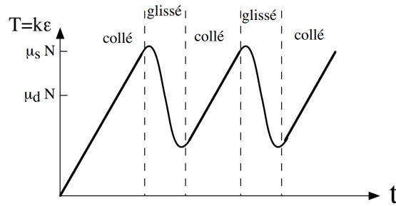
Figure 1.3 – Modèle Stick-Slip [11].
