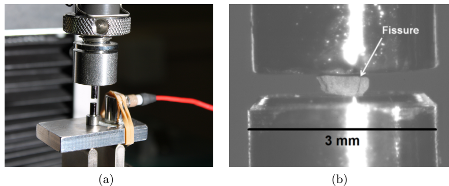
Figure 2.14 – a) Dispositif de micro-compression de granulé d' \text{UO}_2 et fixation du capteur d'émission acoustique, b) fragmentation d'un granulé G160-500 \mu .
