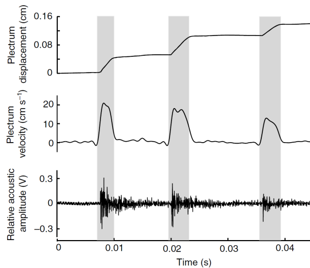
Figure 1.4 – Mesures simultanées du déplacement et de la vitesse de déplacement d'un morceau d'antenne (plectum) contre un morceau de carapace et des signaux acoustiques induits, lors du mouvement « collé-glissé » [12].
