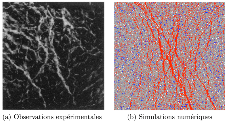
Figure 1.5 – Réseaux de forces au sein de milieux granulaires sous charge : a) observation expérimentale des chaînes de force, formées suite à l’application d’une force de 200 N sur des billes de verre de 3 mm de diamètre, et révélées par biréfringence [18], b) mise en évidence des chaînes de forces normales de compression (en rouge) et des forces de traction (en bleu) au sein d’un échantillon numérique composé de particules consolidées non convexes, simulées par la méthode de dynamique des contacts [22].
