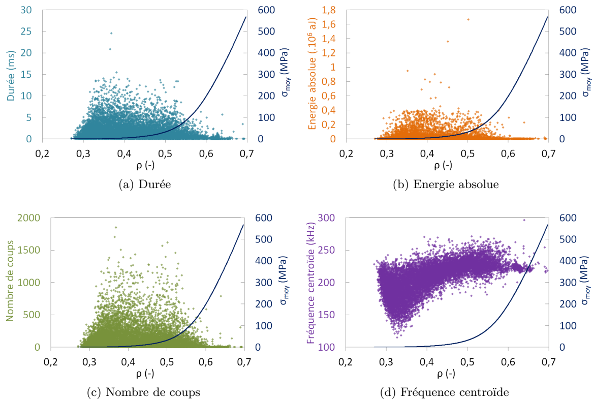
Figure 3.38 – Salves acquises lors de la compaction de granulés G160-500 \mu représentées en : a) durée, b) énergie absolue, c) nombre de coups, d) fréquence centroïde.
