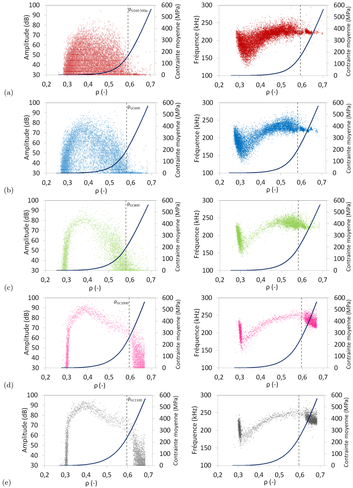
Figure 4.22 – Emission acoustique et courbe de densification lors de la compaction jusqu'à 600 MPa de granulés : a) non consolidés G160-500 \mu , b) GC600, c) GC800, d) GC1000, e) GC1100
