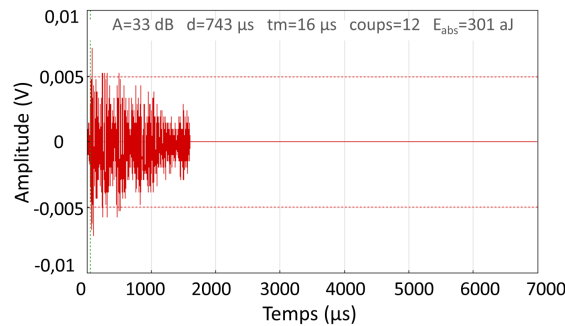
Figure 3.31 – Salve assimilée à un signal continu tronqué, observée lors de la compaction des granulés G45-160μ jusqu'à 0,05 MPa.
