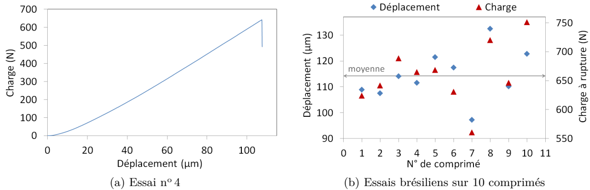
Figure 3.6 – Essais brésiliens sur des comprimés équivalents à des granulés G160-500μ : a) évolution de la charge en fonction du déplacement du poinçon supérieur, b) valeurs des charges et déplacements pour les 10 essais.
