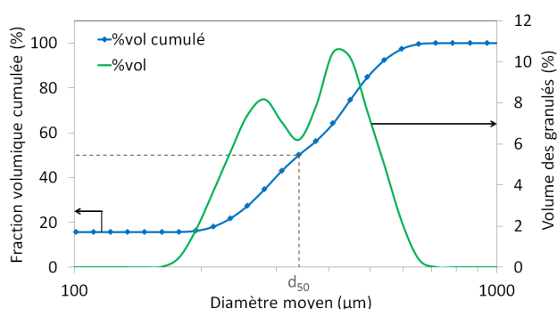
Figure 2.7 – Distribution granulométrique des granules G160-500μ mesurée par granulométrie laser ( d_{50} = 340 \mu\text{m} ).
