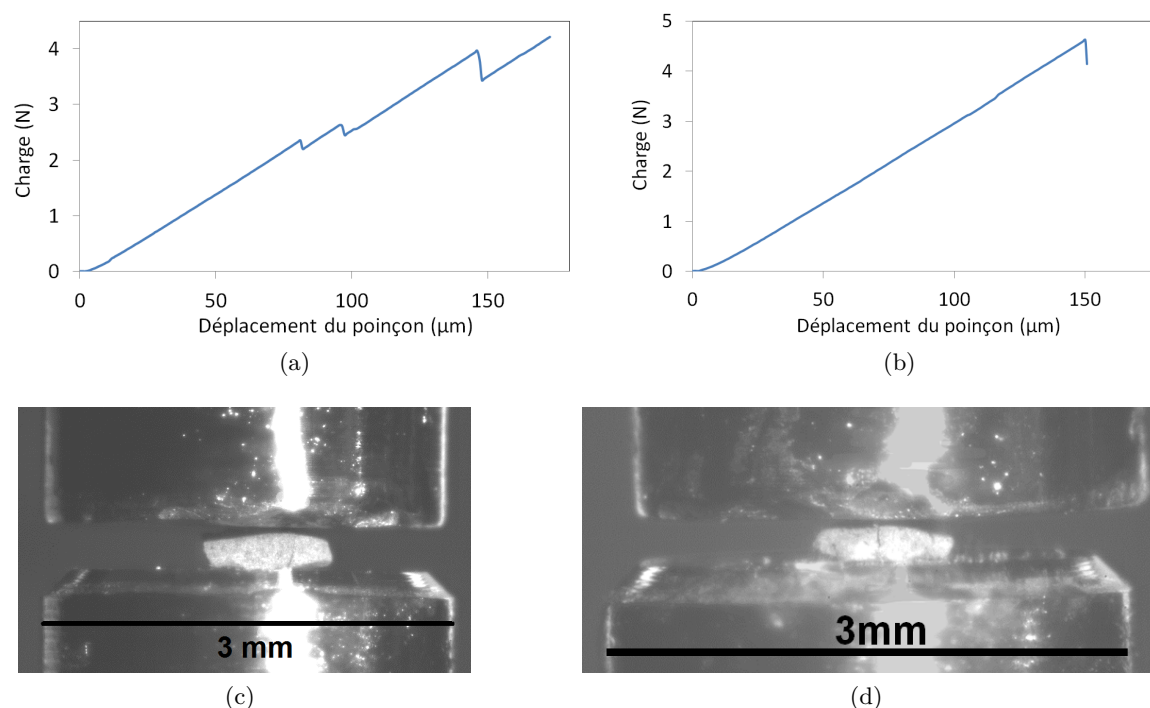
Figure 4.17 – Cisaillements par essai brésilien de granulés GC1000 à l'aide de la machine de micro-compression (cf. §2.3.2.1, p.67) - Courbes de charge et photos des granulés fissurés : a,c) fissure visible au 3 ème saut de charge, b,d) rupture nette du granulé au 1 er saut de charge.
