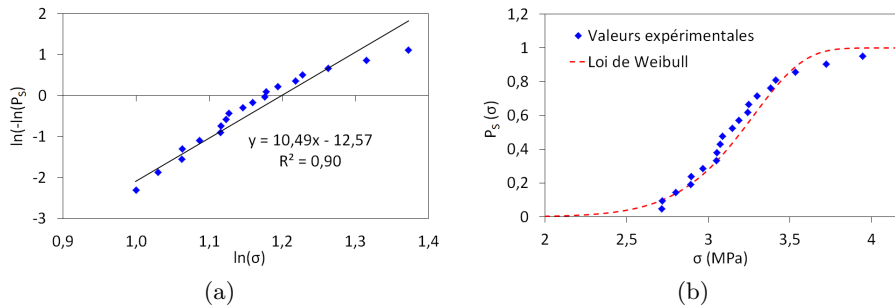
Figure D.1 – Valeurs expérimentales de contrainte à rupture de comprimés d' \text{UO}_2 : a) Détermination du module de Weibull m qui correspond à la pente de la droite, b) Loi de Weibull
