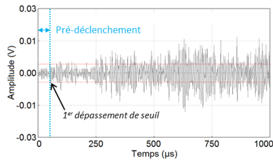
Figure 2.21 – Pré-déclenchement de 50 \mu s de la salve de la Figure 2.20a.
