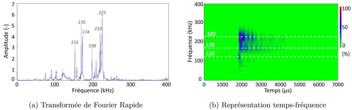
Figure 3.10 – Représentations fréquentielles de la salve acquise au moment de la rupture du granulé n°8 avec le dispositif de micro-compression : a) Transformée de Fourier Rapide, b) représentation temps-fréquence.
