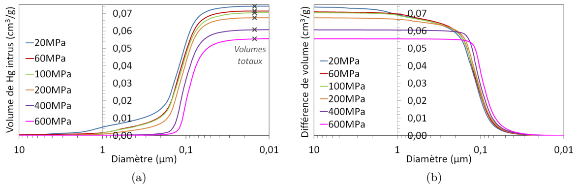
Figure 4.3 – Porosimétrie mercure des comprimés de granulés G160-500 \mu mis en forme à 20, 60, 100, 200, 400 et 600 MPa : a) mesure du volume total de mercure intrus dans les pores, b) calcul de la différence entre le volume total intrus et le volume intrus pour un diamètre donné.
