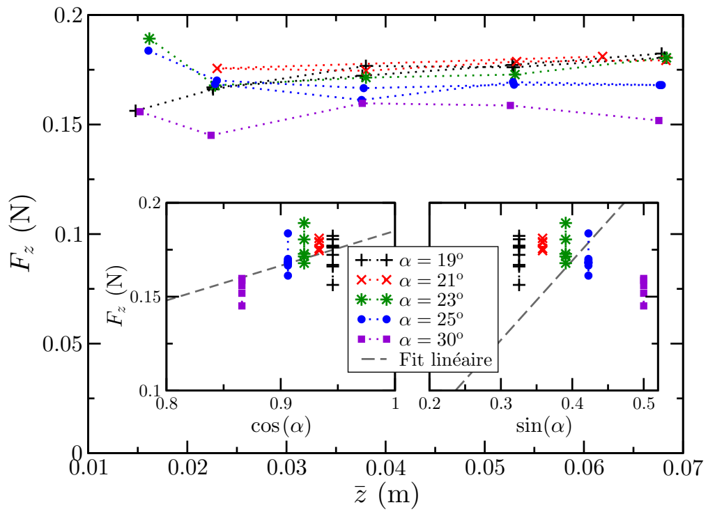
FIGURE 5.5 – Force verticale exercée sur la particule en fonction de son altitude finale, pour différents angles d’inclinaison du plan incliné. Inserts : F_z en fonction du cosinus (gauche) ou du sinus (droite) de \alpha . Les lignes pointillées grises sont les meilleures droites passant par 0.
