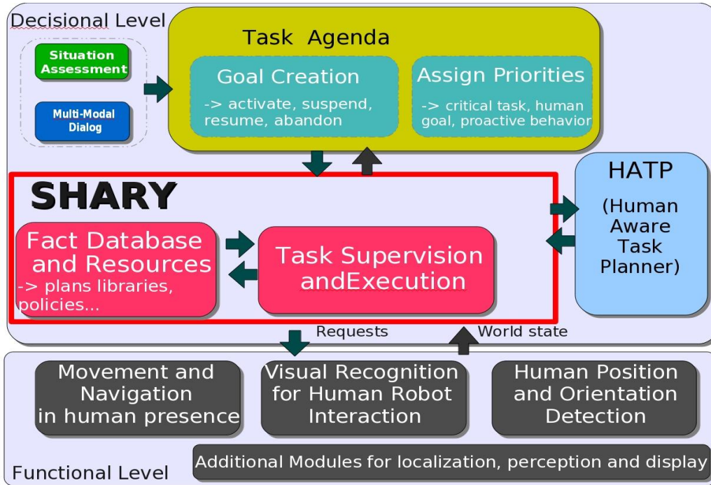
Figure 8.1: Architecture développée pour la gestion des buts et des comportements proactifs
