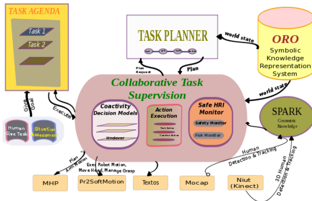
Figure 8.6 : Architecture du système pour le modèle de décision coactivité
