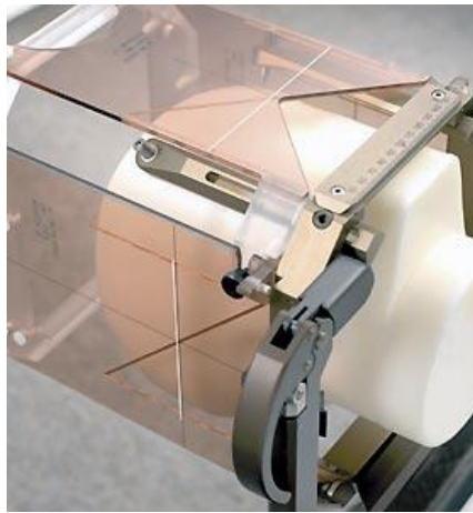
Figure 3 (cliché Elekta). Fixation des fiduciaires destinés au repérage scanner sur un cadre de Leksell.
