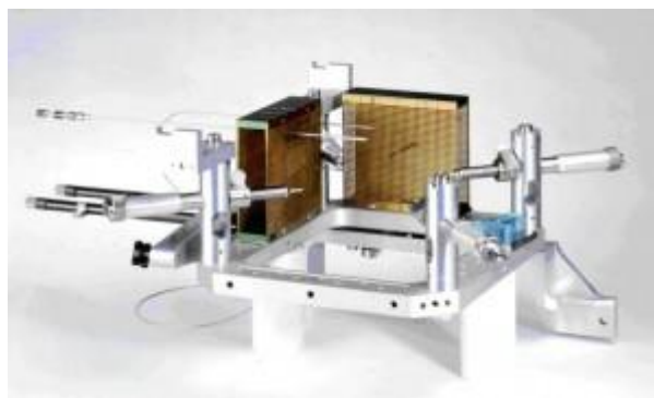
Figure 5 (cliché Dixi Medical). Cadre de stéréotaxie de Talairach, permettant la ponction orthogonale à travers un double système de grilles.
