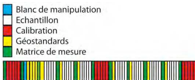
Figure II.23 : Schéma de séquence de mesure par ICP-MS. Les blocs rouges correspondent aux solutions de calibration, le carré bleu au blanc de manipulation, les verts à la matrice de mesure (2% \text{HNO}_3 ), les jaunes aux géostandards, et les blancs aux échantillons.
