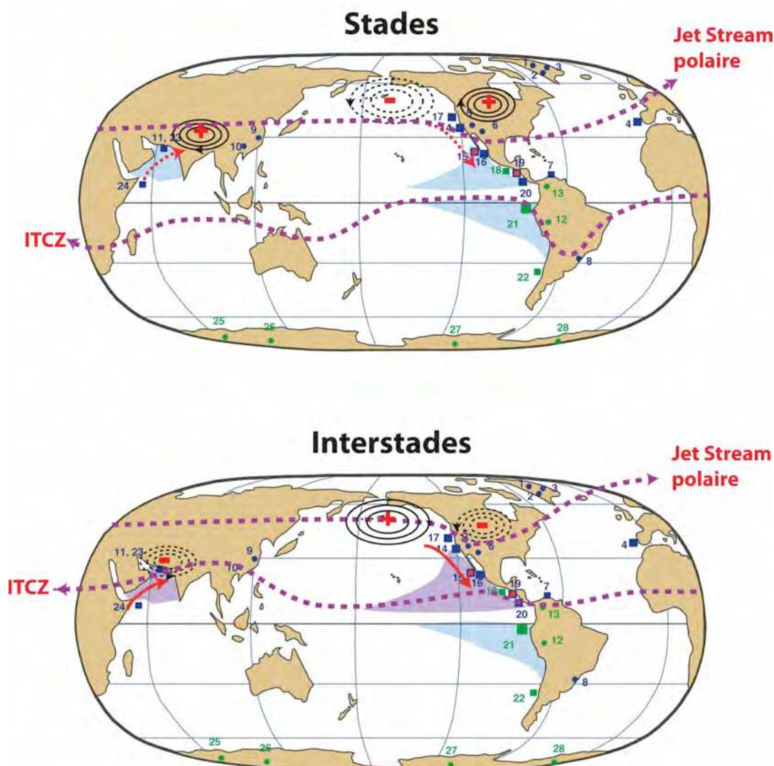
Figure V.3 : Représentation qualitative simplifiée des mécanismes qui affectent les OMZ, durant les stades et les interstades en ce qui concerne la circulation atmosphérique. Les cercles en trait plein (tiret) indiquent une augmentation (diminution) de la pression atmosphérique ; les flèches rouges pleines (tiret) indiquent des vents forts (faibles) dans les diagrammes du bas. La position relative des courants jets polaires et de l'ITCZ est indiquée.
