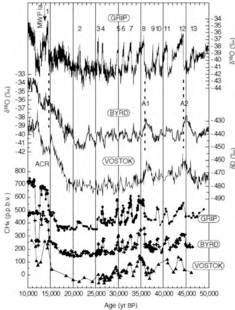
Figure I.11. : Indicateurs des paléotempératures au Groenland (GRIP) et en Antarctique (BYRD et VOSTOK) au cours des derniers 50000 ans, et concentration en méthane dans ces mêmes carottes [Blunier et Brook, 2001].
