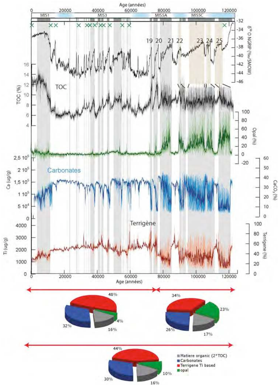
Figure IV.2 : Composants majeurs du sédiment dans la carotte MD02-2508. \delta^{18}\text{O} de la carotte NGRIP [Johnsen et al., 2001] ; Concentrations en TOC estimées par les mesures du Br (II.2.1.2 et III.1) ; Concentrations en opale estimées à l'aide du rapport Si/Ti (II.2.1.2) ; Concentrations en Ca et Ti mesurées par scanneur XRF et calibrées à l'aide des mesures par ICP-MS (II.5). Les concentration en carbonates sont estimées en considérant que le Ca appartient exclusivement à la phase carbonatée. Les concentrations en matériaux terrigènes sont estimées à partir des concentrations en Ti dans la carotte MD08 et dans la croûte continentale (UPC, [McLennan, 2001]). Les compositions moyennes pour les intervalles MIS1-MIS4, pour le MIS5, et l'intégralité de la carotte sont indiquées sur les diagrammes du bas. Les bandes verticales correspondent aux intervalles laminés dans la carotte MD08. Les bandes plus claires dans le MIS5 soulignent les interstades chauds identifiés dans la carotte NGRIP. Les positions des points utilisés pour établir le modèle d'âge (II.1) sont indiquées par des croix au sommet de la figure.
