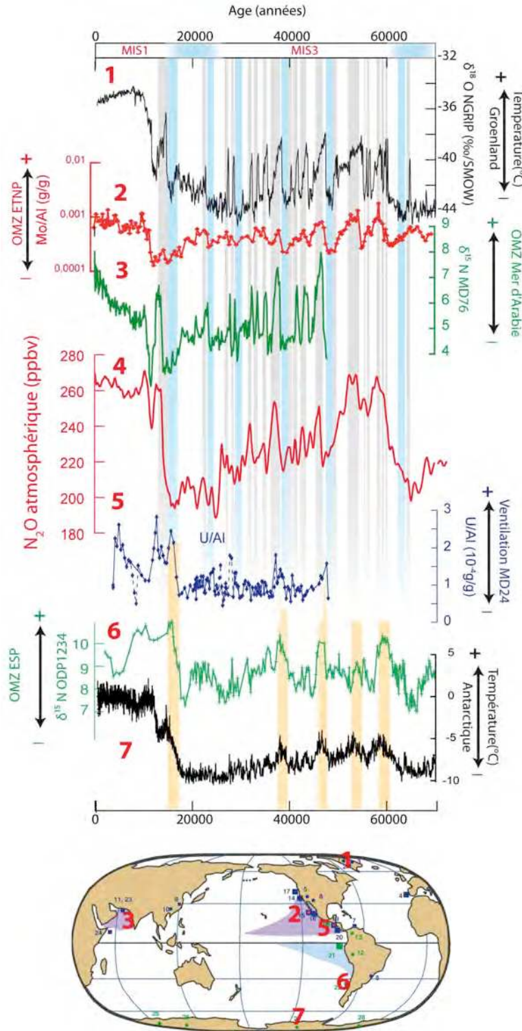
Figure V.2 : 1. \delta^{18}O de la carotte NGRIP [Johnsen et al., 2001]; 2. Rapport Mo/Al dans la carotte MD08 (cette étude) ; 3. \delta^{15}N de la carotte MD04-2876 [Pichevin et al., 2007]; 4. Concentrations en N_2O atmosphérique [Schilt et al., 2010] ; 5. Rapport U/Al de la carotte MD24 (cette étude) ; 6. \delta^{15}N de la carotte ODP1234 [Robinson et al., 2007] ; Températures au niveau de la carotte EDC [Jouzel et al., 2007]. La position des enregistrements est indiquée sur la carte au bas de la Figure.
