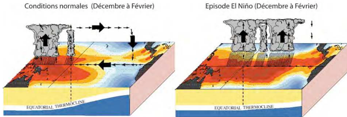
Figure I.4. : Cellule de Walker dans le Pacifique tropical. Les conditions normales de décembre à février sont représentées sur le graphique de gauche. La convection est marquée à l'Ouest, tandis que la profondeur de la thermocline est faible à l'Est. L'illustration de droite représente les conditions dans le Pacifique tropical lors d'une année El Nino. Les eaux chaudes et la convection atmosphérique migrent vers l'est du Pacifique, engendrant un réchauffement des eaux de surface à l'Est, et un approfondissement de la thermocline. D'après [Cane, 2005].
