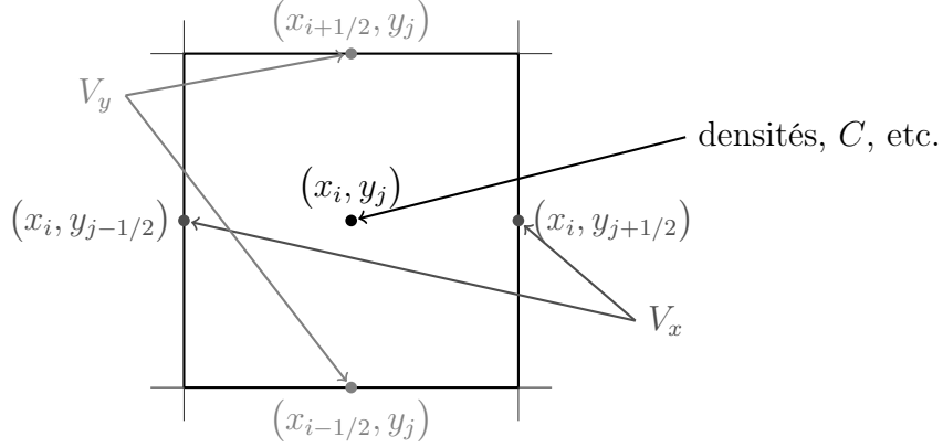
FIGURE 5.2 – Discrétisation des différentes quantités
