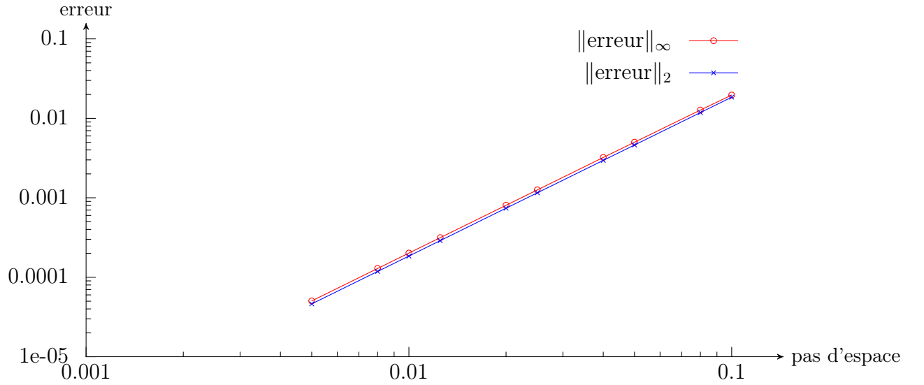
FIGURE 5.8 – Erreur relative pour l'équation de Poisson anisotrope avec un coefficient constant et sans pénalisation. Les nuages de points représentent les erreurs numériques mesurées et les courbes les interpolations retenues (par une fonction de la forme x \rightarrow bx^a ), ayant fourni les ordres numériques annoncés : ordre 1,99 en norme L^\infty et 2,00 en norme L^2 .
