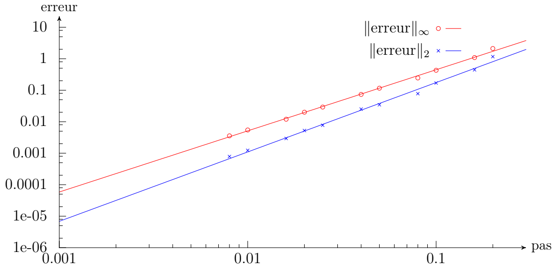
FIGURE 5.19 – Erreur relative - Les nuages de points représentent les erreurs numériques mesurées et les courbes les interpolations retenues (par une fonction de la forme x \rightarrow bx^a ), donnant les ordres numériques annoncés. On mesure un ordre numérique égal à 1,94 sur la norme L^\infty et 2,20 sur la norme L^2 .
