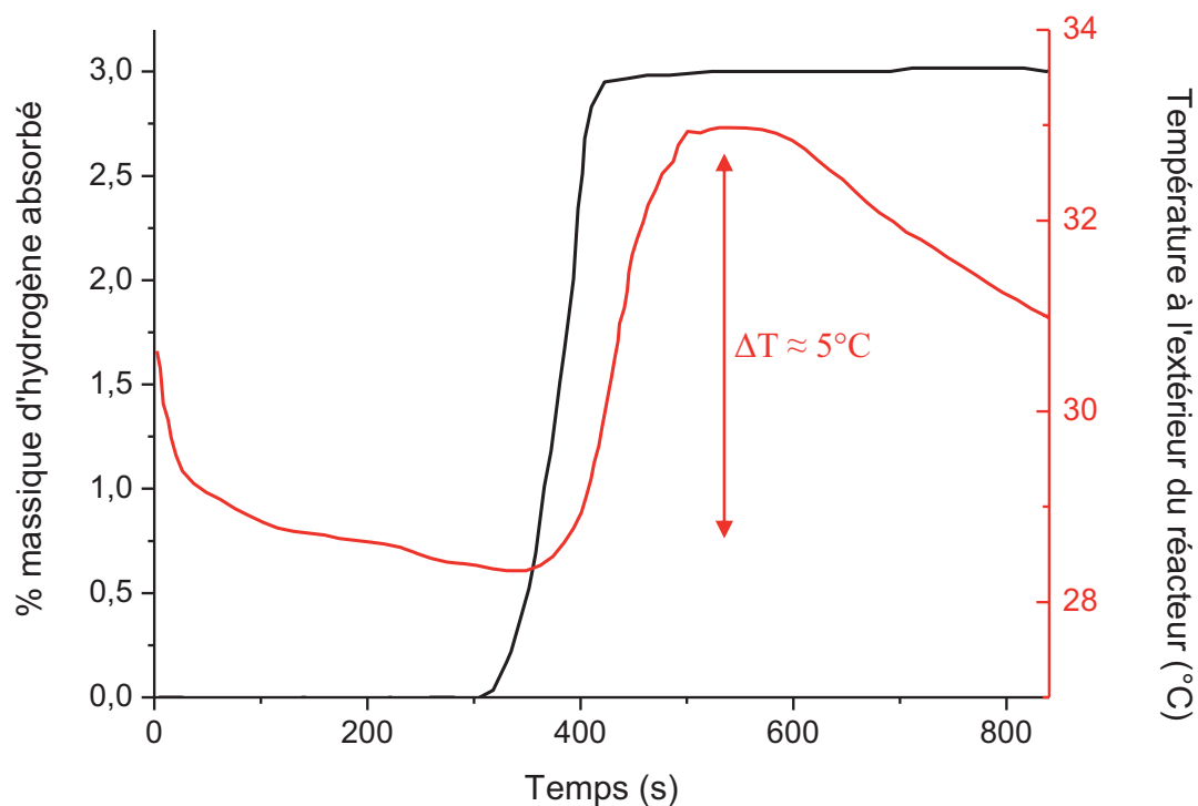
Figure III. 10 : Suivi de la température extérieure du réacteur lors de l'hydruration de \text{Y}_4\text{NiMg} à 20^\circ\text{C} sous 10 bar de \text{H}_2 [17].
