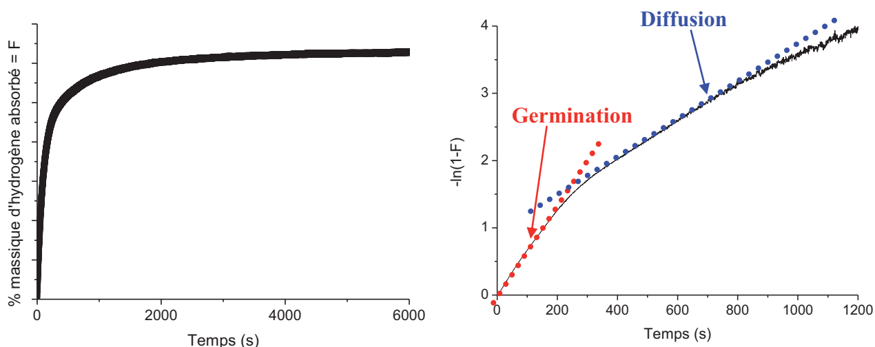
Figure I.6 : Allure d'une courbe d'absorption (gauche) exploitée à l'aide du modèle cinétique Avrami-Erofeev (droite).
