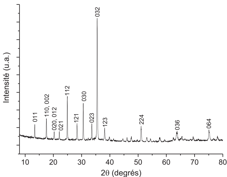
Figure IV.2 : Diffractogramme de rayons X de l'échantillon \text{La}_{10}\text{Cu}_{10}\text{Mg}_{80} (appelé par la suite \text{LaCuMg}_8 ) après fusion. Seul les pics les plus intenses ont été indexés.
