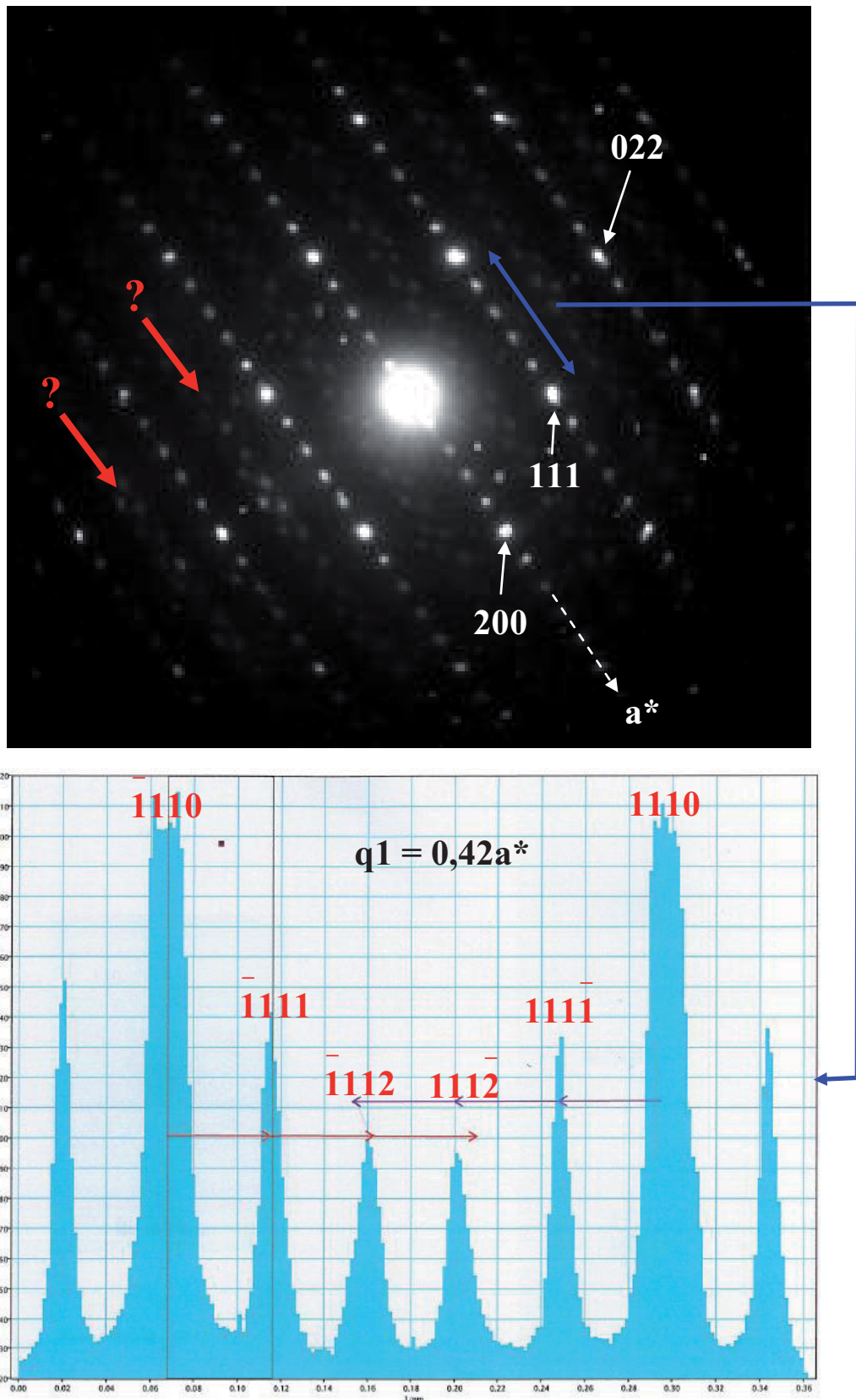
Figure IV.38 : Evolution des intensités de chaque spot de diffraction du cliché IV.37.d, selon l'axe a^* . L'indexation des spots de diffraction, en considérant une structure modulée incommensurable de vecteur 0,42a^* est proposée sous la figure.
