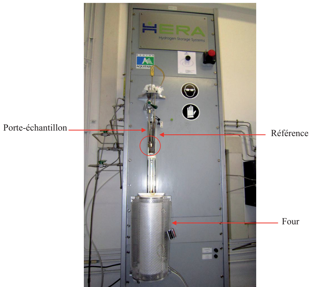
Figure II.5 : Photo du banc d'hydruration HERA. L'échantillon est placé dans le réacteur (cercle rouge).
