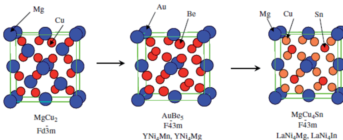
Figure I.14 : Relation structurale entre la structure type cubique AB_2 et les structures types dérivées de \text{AuBe}_5 et \text{MgCu}_4\text{Sn} . Le changement de groupe d'espace induit de nouvelles conditions de réflexion pour le plan [h00] avec h = 2n et le plan [hk0] avec h+k = 2n [104].
