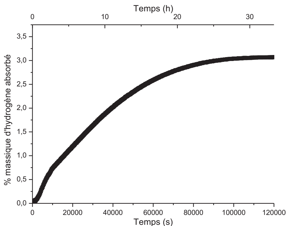
Figure IV.13 : Première cinétique d'absorption à 300°C du composé \text{LaCuMg}_8 sous une pression de 10 bar de \text{H}_2 .
