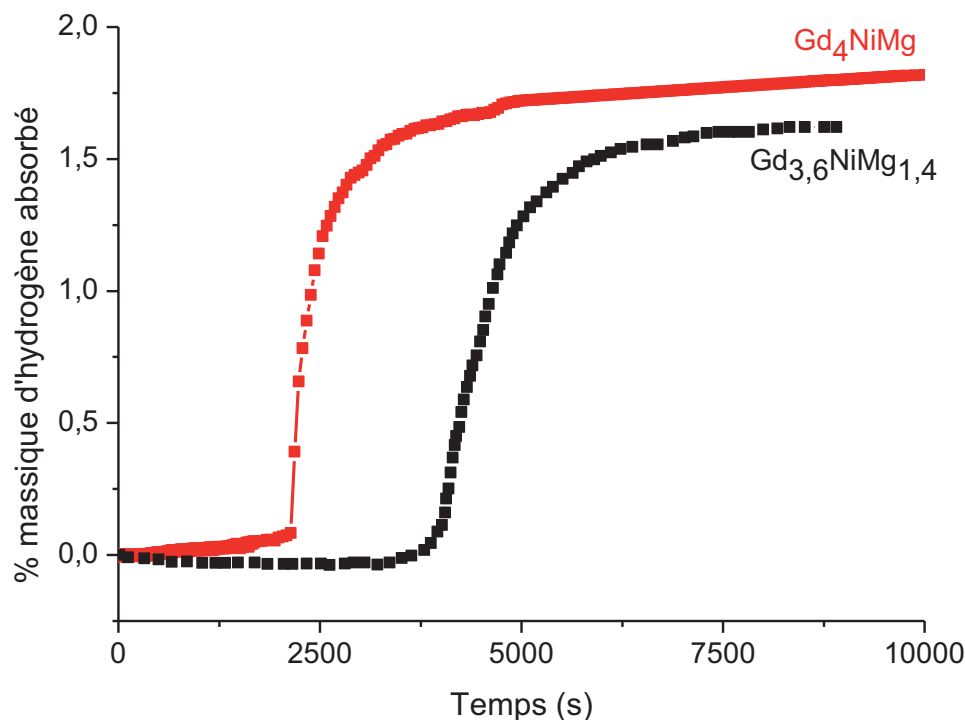
Figure III.24 : Cinétique d'absorption pour les composés \text{Gd}_4\text{NiMg} (rouge) et \text{Gd}_{3,6}\text{NiMg}_{1,4} (noir), sous 10 bar d'hydrogène à 20°C.
