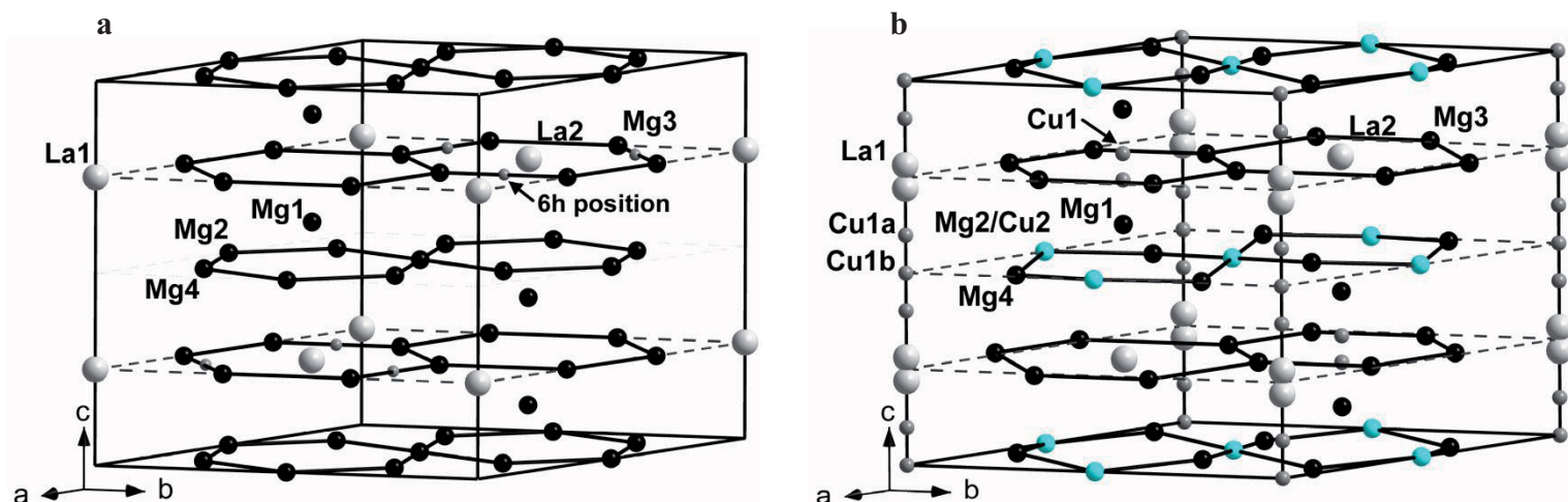
Figure IV.7 : Structures cristallines des composés \text{La}_2\text{Mg}_{17} (a) et \text{LaCuMg}_8 (b). Le réseau de magnésium, semblable au graphite, est accentué sur la figure en reliant les atomes de magnésium entre eux.
