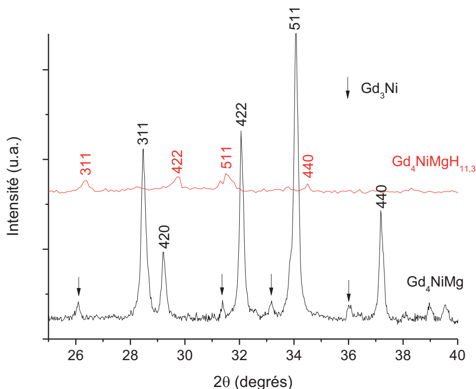
Figure III.6 : Diffractogramme de rayons X entre 25° et 40° de l'échantillon \text{Gd}_4\text{NiMg} avant hydruation (noir) et après hydruation (rouge).
