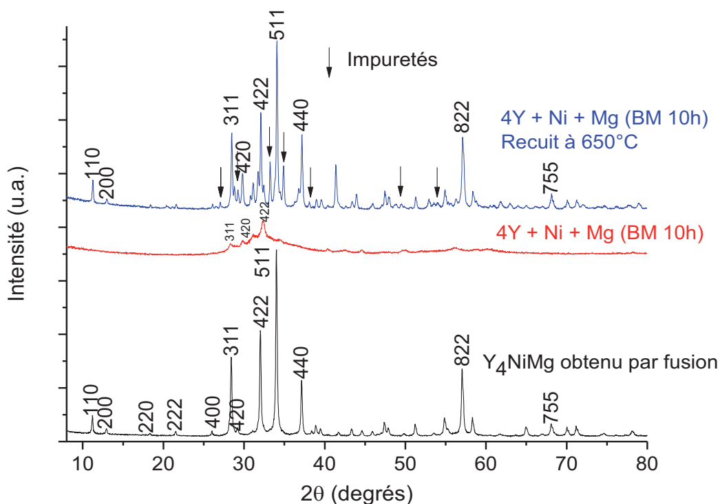
Figure III.3 : Diffractogramme de rayons X de l'échantillon Y_4NiMg synthétisé en tube de tantale après recuit (noir), par mécanosynthèse pendant 10h (rouge) puis recuit à 650°C pendant 1h (bleu). Les pics de diffraction non identifiés peuvent être indexés avec la structure type Gd_4RhIn mais, par souci de clarté, seuls les plus intenses sont indexés ici.
