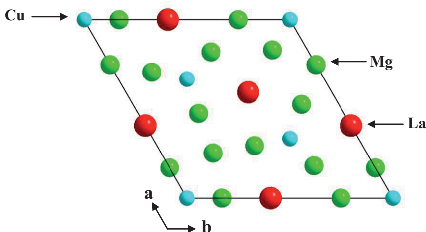
Figure I.15 : Structure cristalline du composé \text{LaCuMg}_4 [114].
