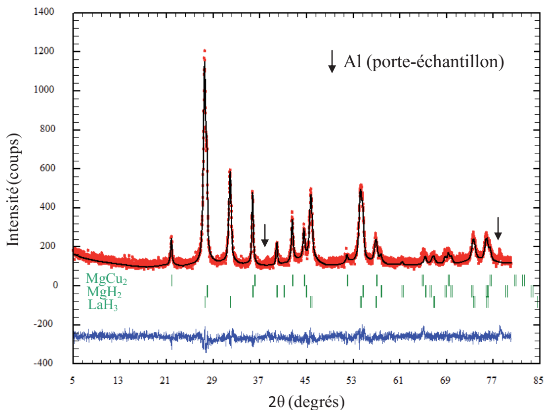
Figure IV.15 : Affinement Rietveld du diffractogramme de rayons X relatif au composé \text{LaCuMg}_8 , après la première absorption d'hydrogène sous 10 bar de \text{H}_2 à 300°C.
