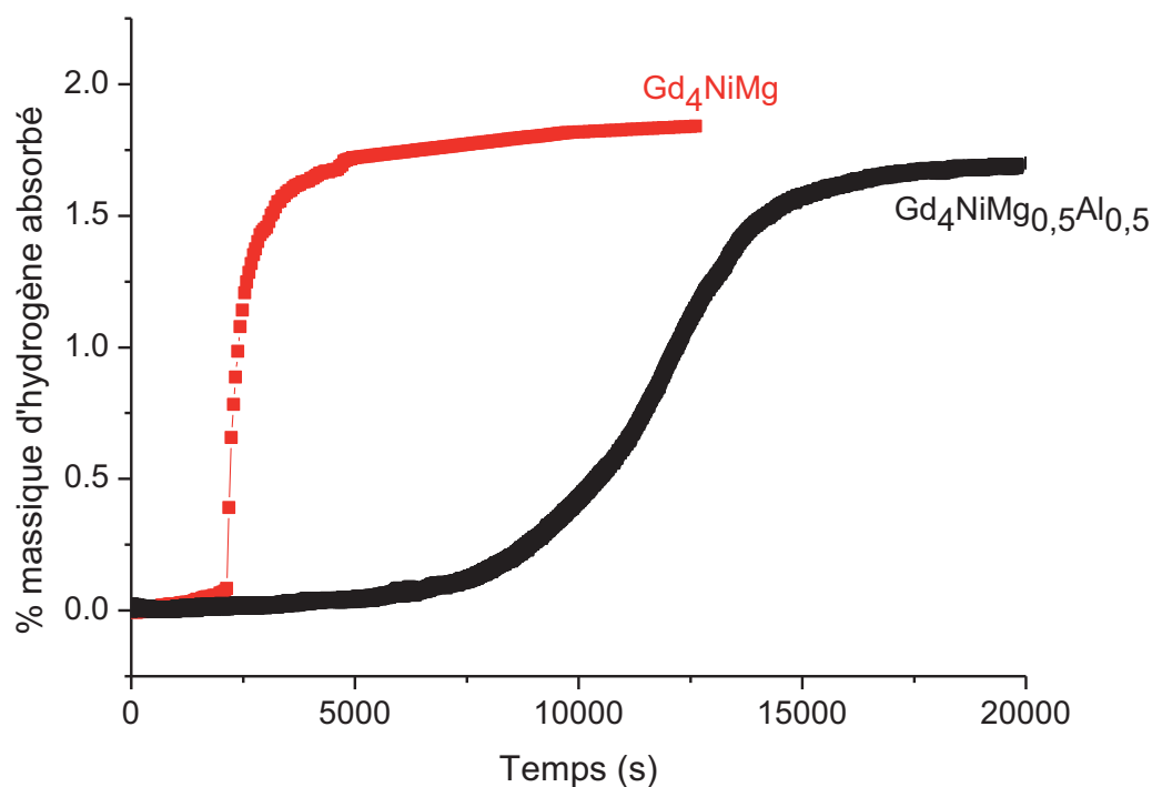
Figure III. 22 : Cinétique d'absorption pour les composés \text{Gd}_4\text{NiMg} (rouge) et \text{Gd}_4\text{NiMg}_{0,5}\text{Al}_{0,5} (noir), sous 10 bar d'hydrogène à 20°C.
