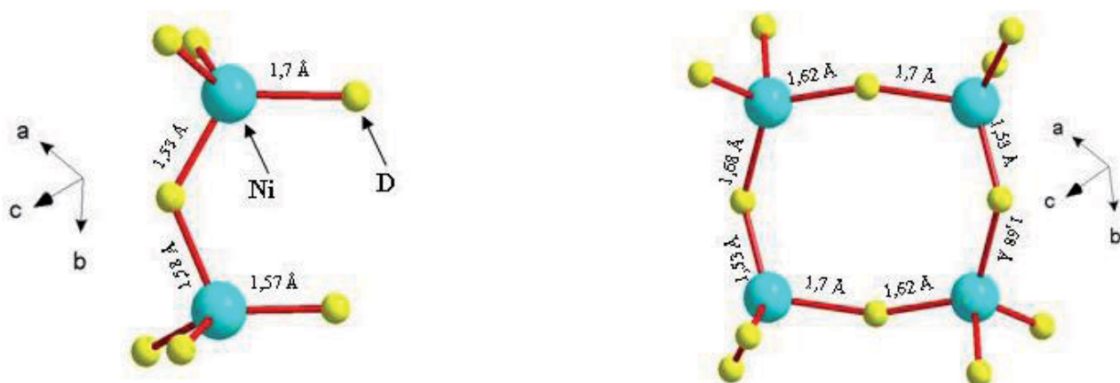
Figure I.10 : Complexes [\text{Ni}_2\text{D}_7]^{7-} (gauche) et [\text{Ni}_4\text{D}_{12}]^{12-} (droite) dans le deutéride \text{La}_2\text{Ni}_2\text{MgD}_8 [68]
