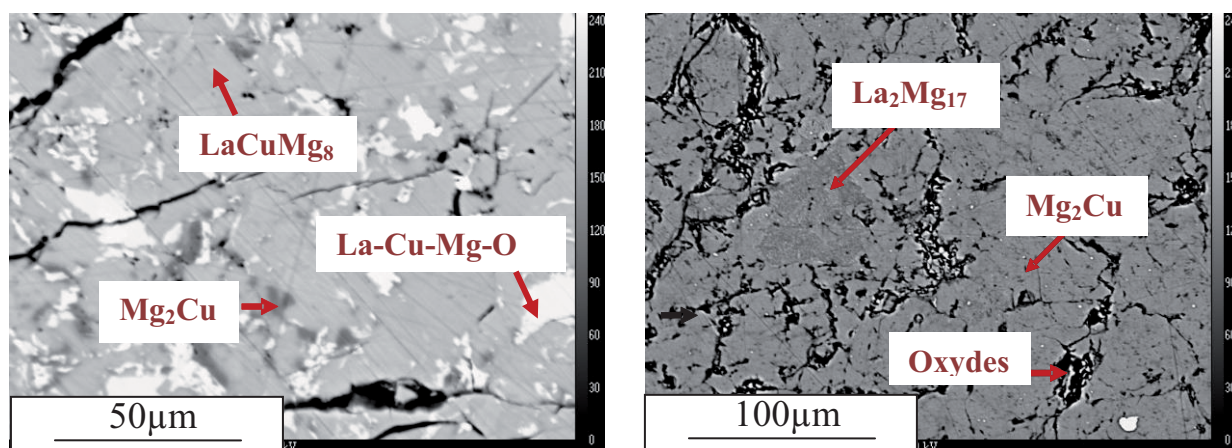
Figure IV.10 : Images microsonde (a) du composé \text{LaCuMg}_8 obtenu par fusion et (b) du mélange \text{La}_2\text{Mg}_{17} + \text{Mg}_2\text{Cu} obtenu par mécanosynthèse après 20 laminages.
