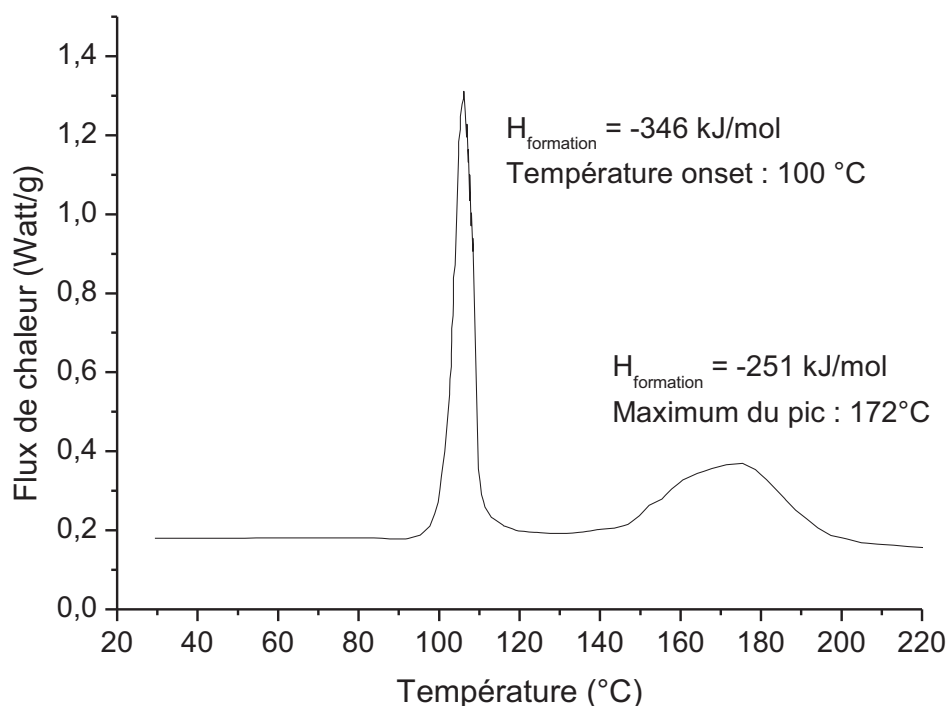
Figure III. 9 : Analyse DSC sur l'échantillon \text{Gd}_4\text{NiMg} sous 10 bar d'hydrogène (montée en température de 1^\circ\text{C}/\text{min} ) réalisée en collaboration avec l'équipe du Dr. F. Castro (Argentine) [17].
