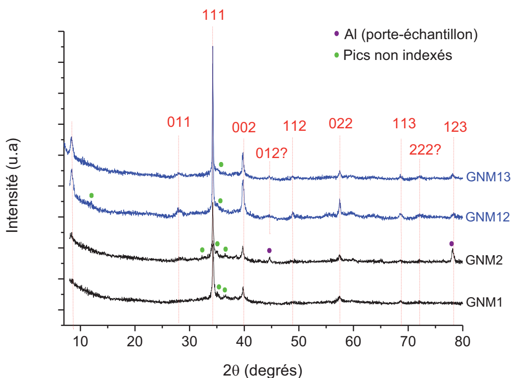
Figure IV.34 : Diffractogramme de rayons X des échantillons GNM1, GNM2, GNM12 et GNM13. Les pics de diffraction de la maille cubique de paramètre a \approx 4,55 Å sont donnés en pointillés rouges.
