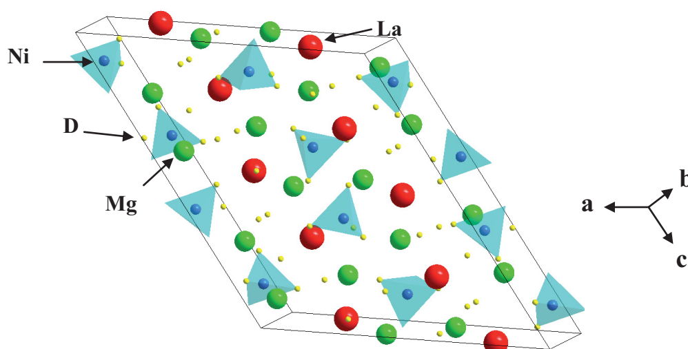
Figure I.11 : Structure de l'hydruide \text{LaNiMg}_2\text{D}_7 . Les tétraèdres [\text{NiD}_4]^{4-} sont représentés en bleu [69].
