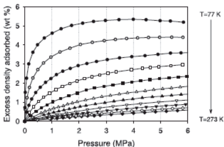
Figure I.1 : Evolution de la capacité massique d'hydrogène absorbé par un charbon actif AX-21TM à 77\text{ K} puis de 93 à 273\text{ K} par pas de 20\text{ K} [8].
