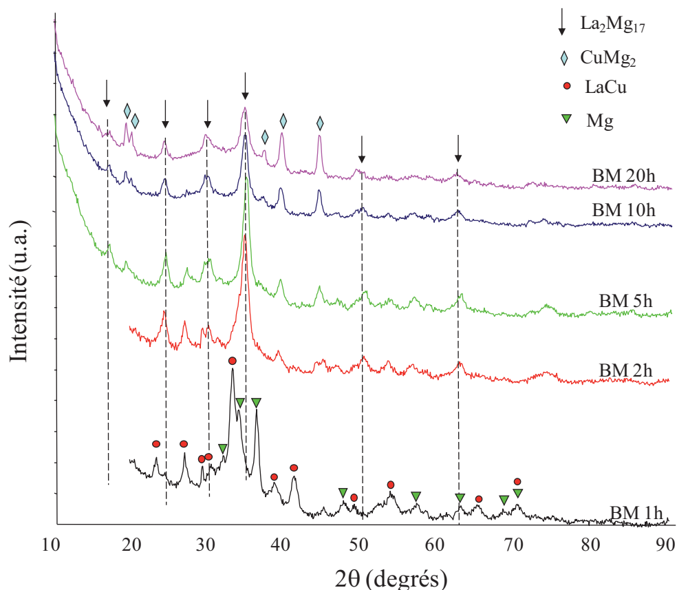
Figure IV.9. Diffractogrammes de rayons X du mélange de poudres \text{LaCu} + 8\text{Mg} , après 1h, 2h, 5h, 10h et 20h de broyage (BM).
