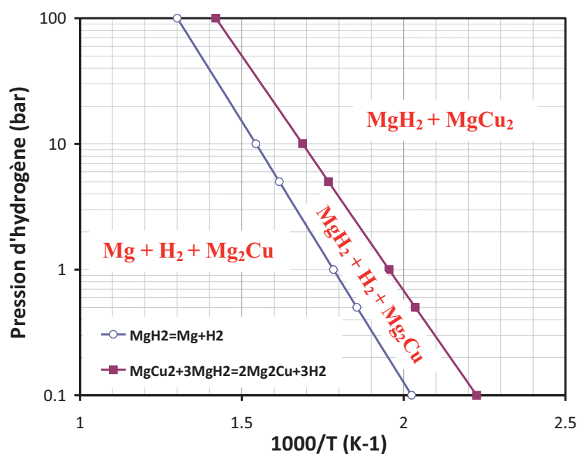
Figure IV.21 : Droites de Van't Hoff pour la réaction du magnésium (bleu) et du composé \text{Mg}_2\text{Cu} (rouge) avec l'hydrogène.
