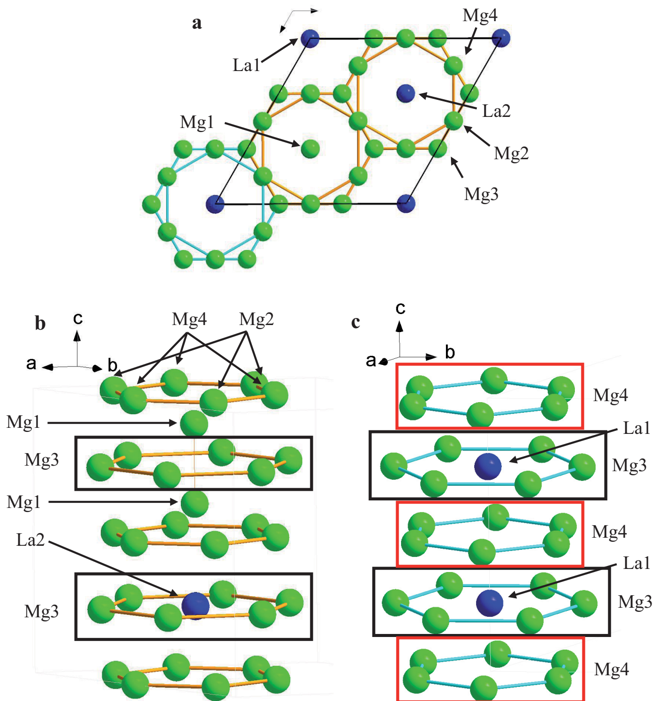
Figure IV.5 : Structure type \text{La}_2\text{Mg}_{17} dans le plan (a,b) (a) et selon l'axe c (b,c). Deux types de canaux sont observés selon l'axe c : le canal centré en (1/3, 2/3, z) (b) et le canal centré en (0, 0, z) (c).
