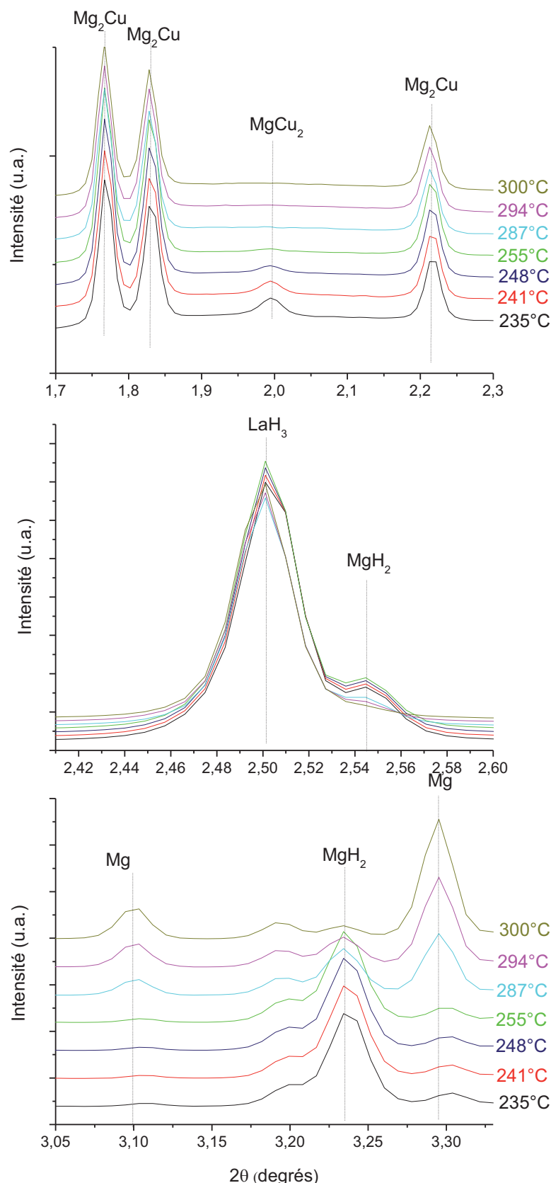
Figure IV.24 : Suivi de la réaction de déshydruration par diffraction des rayons X (rayonnement synchrotron, \lambda = 0,14254 \text{ \AA} ) de la poudre \text{LaCuMg}_8 activée sous 1 bar d'argon en fonction de la température. Pour plus de clarté, trois zooms sont proposés ( 1,7^\circ < 2\theta < 2,3^\circ ; 2,41^\circ < 2\theta < 2,6^\circ et 3,05^\circ < 2\theta < 3,35^\circ ).
