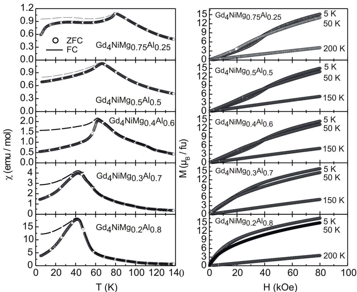
Figure III.20 : Mesure magnétique pour la solution solide \text{Gd}_4\text{NiMg}_{1-x}\text{Al}_x : Evolution de la susceptibilité magnétique en fonction de la température en mode ZFC et FC et dans un champ extérieur de 100 Oe (a). Evolution de l'aimantation en fonction du champ appliqué pour différentes températures (b).
