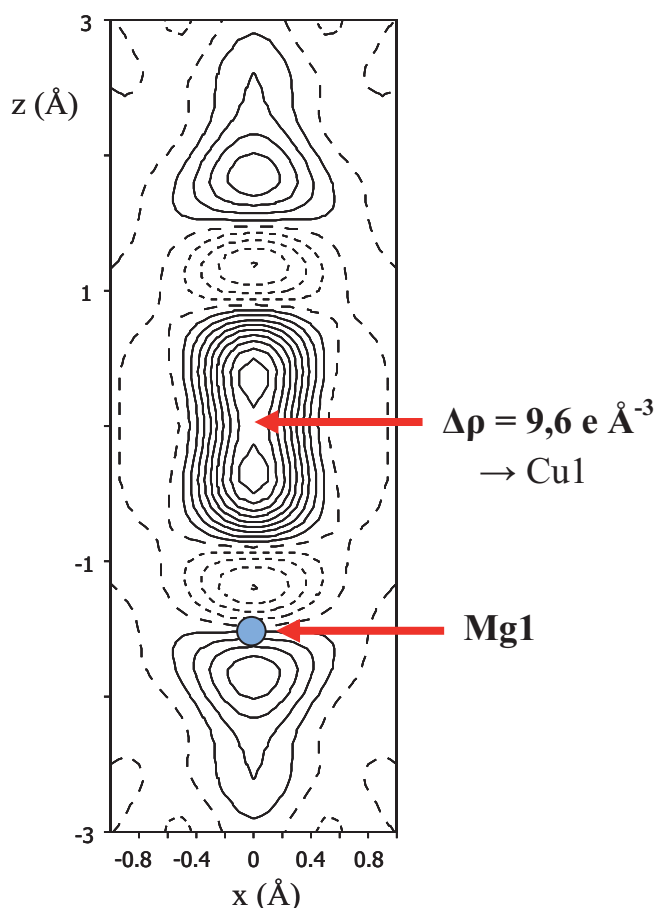
Figure IV.6 : Cartes de Fourier-Différence des chaînes (0, 0, z) et (1/3, 2/3, z) obtenues à partir de la mesure de diffraction des rayons X sur monocristal avec le modèle de départ basé sur la structure type \text{La}_2\text{Mg}_{17} .
