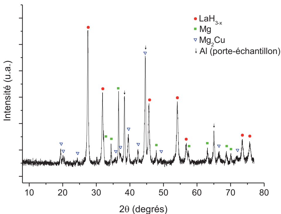
Figure IV. 16 : Diffractogramme de rayons X de l'échantillon \text{LaCuMg}_8 après décomposition sous hydrogène et désorption à 300°C sous 0,2 bar d'hydrogène.
