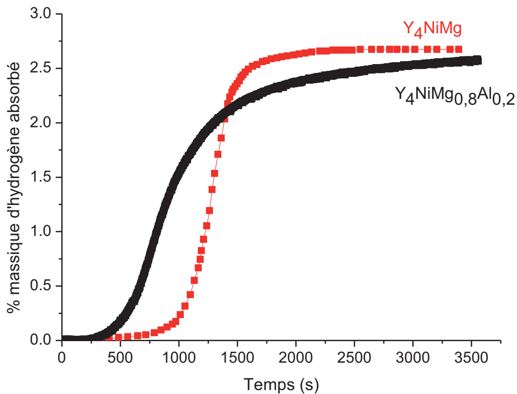
Figure III.23 : Cinétique d'absorption pour les composés \text{Y}_4\text{NiMg} (rouge) et \text{Y}_4\text{NiMg}_{0,8}\text{Al}_{0,2} (noir), sous 10 bar d'hydrogène à 20°C.
