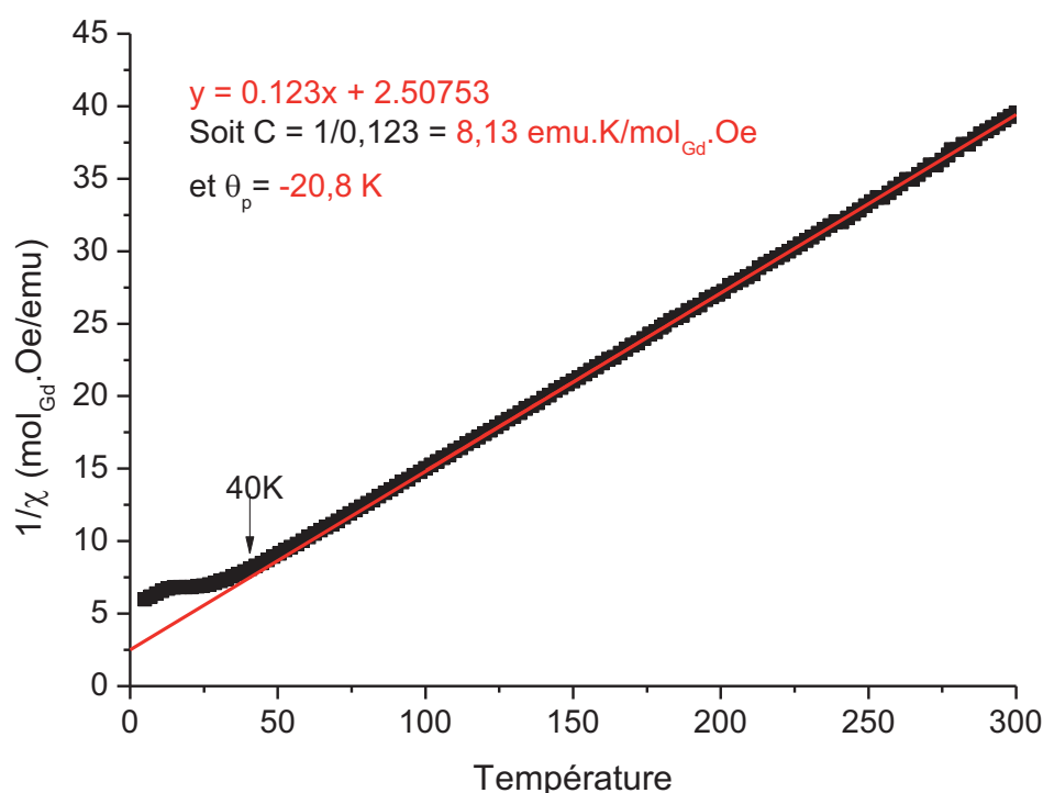
Figure IV.49 : Loi de Curie-Weiss pour l'échantillon \text{Gd}_{13}\text{Ni}_{9,5}\text{Mg}_{77,5} .
