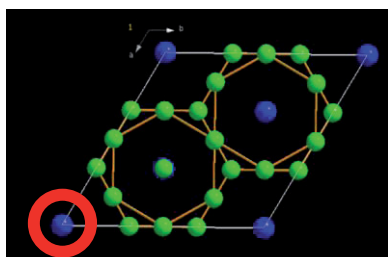
Chaîne (0, 0, z)
