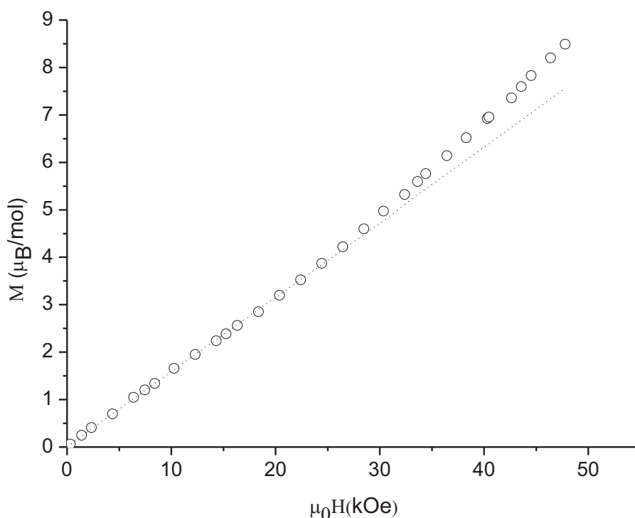
Figure III.13 : Evolution de l'aimantation du composé \text{Gd}_4\text{NiMg} en fonction du champ, à 10 K [7].
