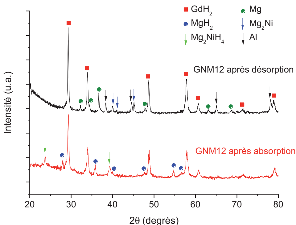
Figure IV.43 : Diffractogrammes de rayons X de l'échantillon GNM12 mesuré en fin d'absorption et en fin de désorption.
