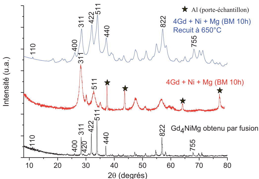
Figure III.2 : Diffractogramme de rayons X de l'échantillon Gd_4NiMg synthétisé en tube de tantale après recuit (noir), par mécanosynthèse pendant 10h (rouge) puis recuit à 650°C pendant 1h (bleu). Tous les pics de diffraction non identifiés peuvent être indexés avec la structure type Gd_4RhIn mais, par souci de clarté, seuls les plus intenses sont indexés ici.
