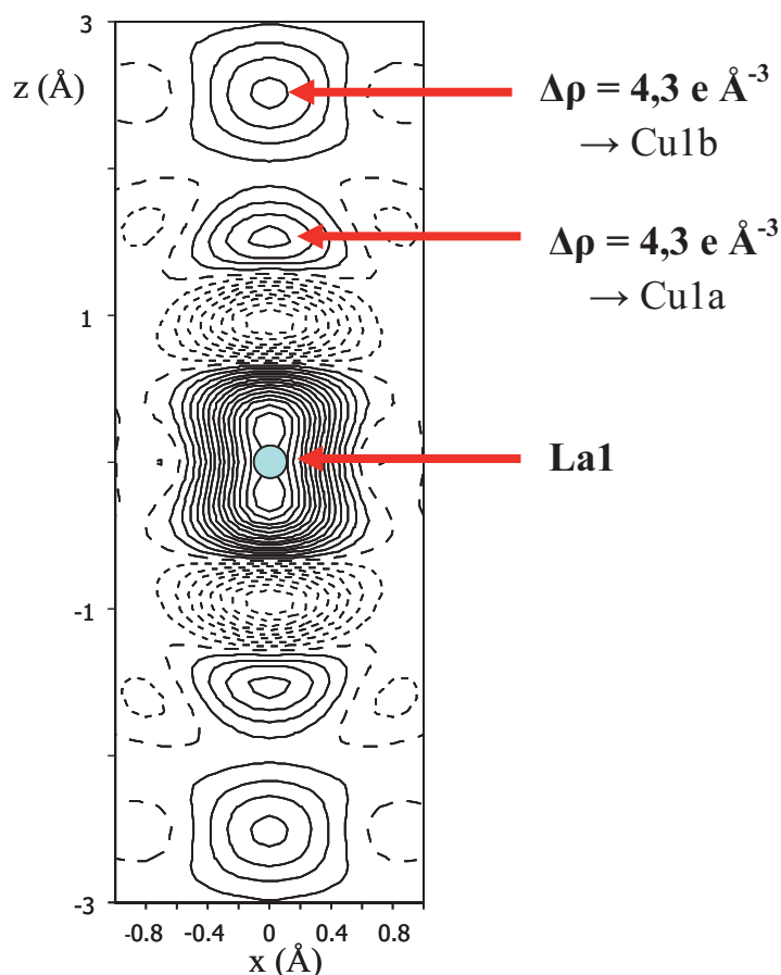
Figure IV.6 : Cartes de Fourier-Différence des chaînes (0, 0, z) et (1/3, 2/3, z) obtenues à partir de la mesure de diffraction des rayons X sur monocristal avec le modèle de départ basé sur la structure type \text{La}_2\text{Mg}_{17} .
