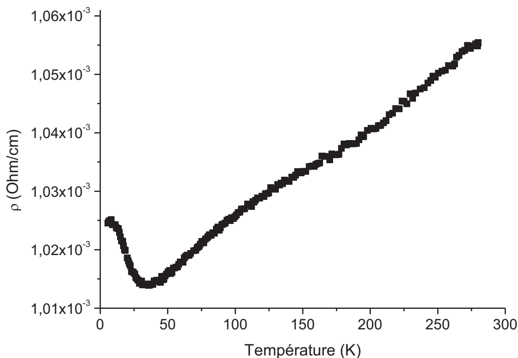
Figure IV.46 : Evolution de la résistivité de l'échantillon \text{Gd}_{13}\text{Ni}_{9,5}\text{Mg}_{77,5} en fonction de la température obtenue à l'aide d'une mesure 4 pointes.
