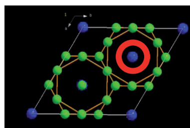
Chaîne (1/3, 2/3, z)
