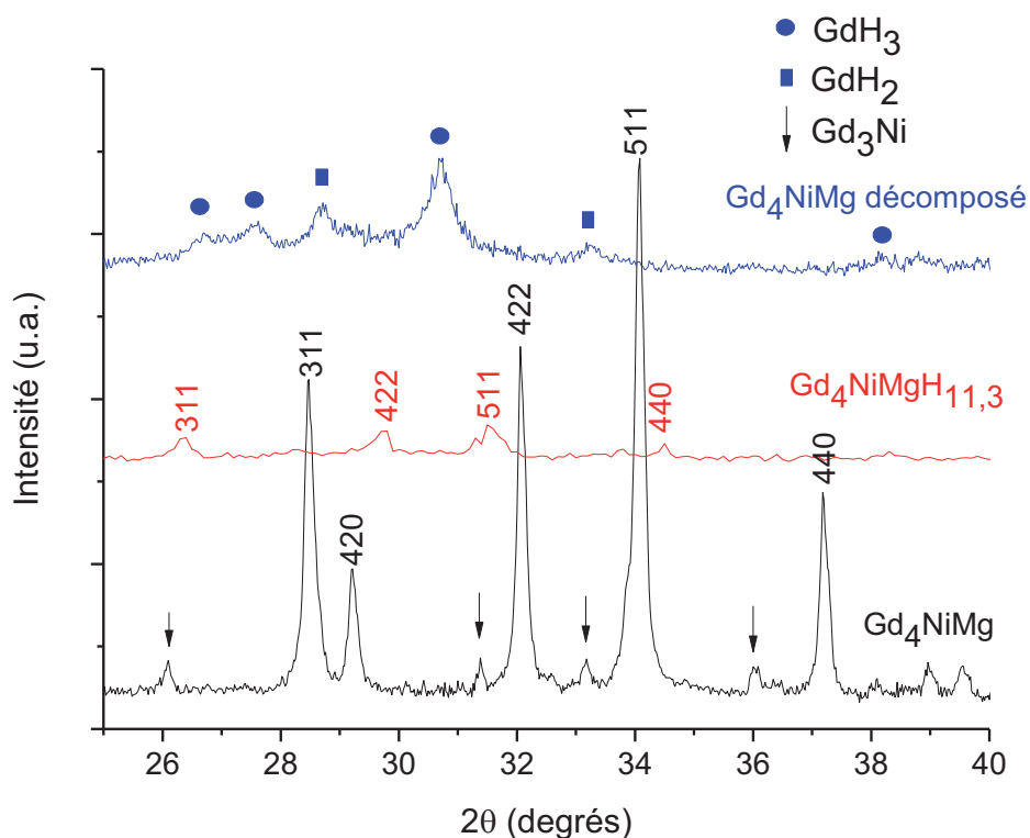
Figure III. 8 : Diffractogramme de rayons X entre 25^\circ et 40^\circ de l'échantillon \text{Gd}_4\text{NiMg} avant hydruation (noir), après hydruation à 20^\circ\text{C} sous 10 bar de \text{H}_2 (rouge) et après décomposition à 100^\circ\text{C} sous 10 bar de \text{H}_2 (bleu)[7].
