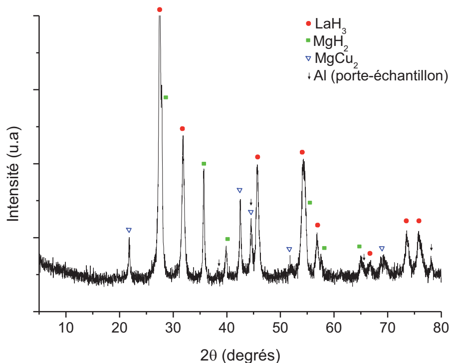
Figure IV.14 : Diffractogramme de rayons X de l'échantillon \text{LaCuMg}_8 après la première absorption d'hydrogène sous 10 bar de \text{H}_2 à 300°C.
