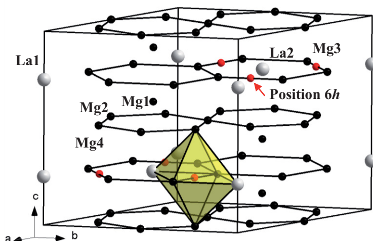
Figure IV.8 : Structure du composé \text{La}_2\text{Mg}_{17} faisant apparaître le site 6h hypothétique de l'hydrogène (en rouge) lors de la formation de l'hydruire \text{La}_2\text{Mg}_{17}\text{H}_x .
