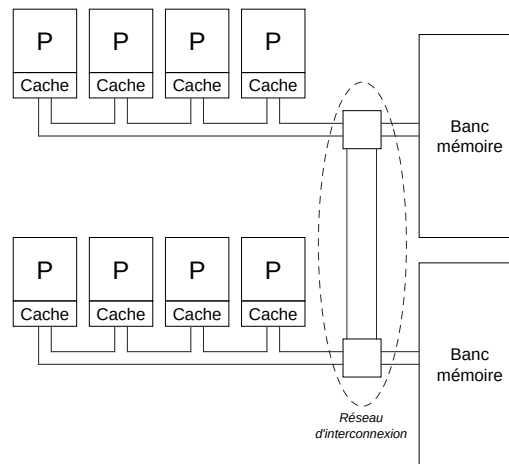
FIG. 1.3 – Architecture NUMA à deux nœuds de quatre processeurs.
