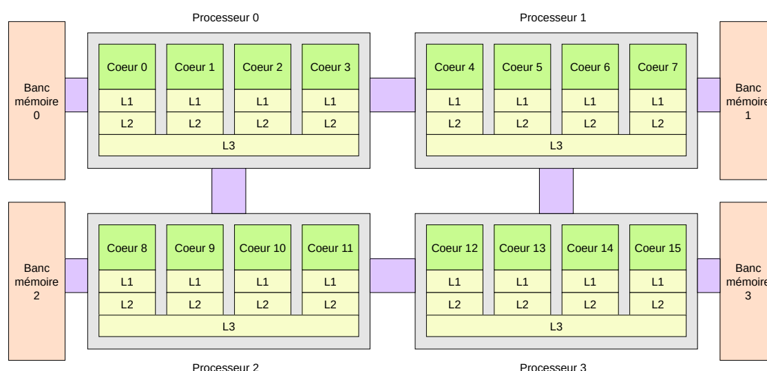
FIG. 2.1 – Architecture multicœur composée de 4 processeurs à 4 cœurs de type Opteron.
