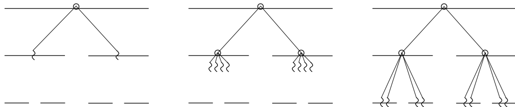
(a) Placement des threads après ordonnancement de la région parallèle externe. (b) Création locale des threads issus des régions parallèles imbriquées. (c) Ordonnement local des équipes nouvellement créées.
