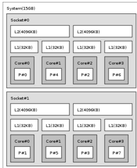
FIG. 2.2 – Architecture bi-quadriceur Opteron modélisée par la bibliothèque hwloc.
