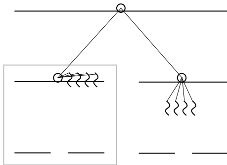
(c) Eclatement de bulle par l'ordonnanceur.
