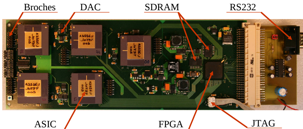
Figure 2.8. Photographie de la carte Gaillimh
