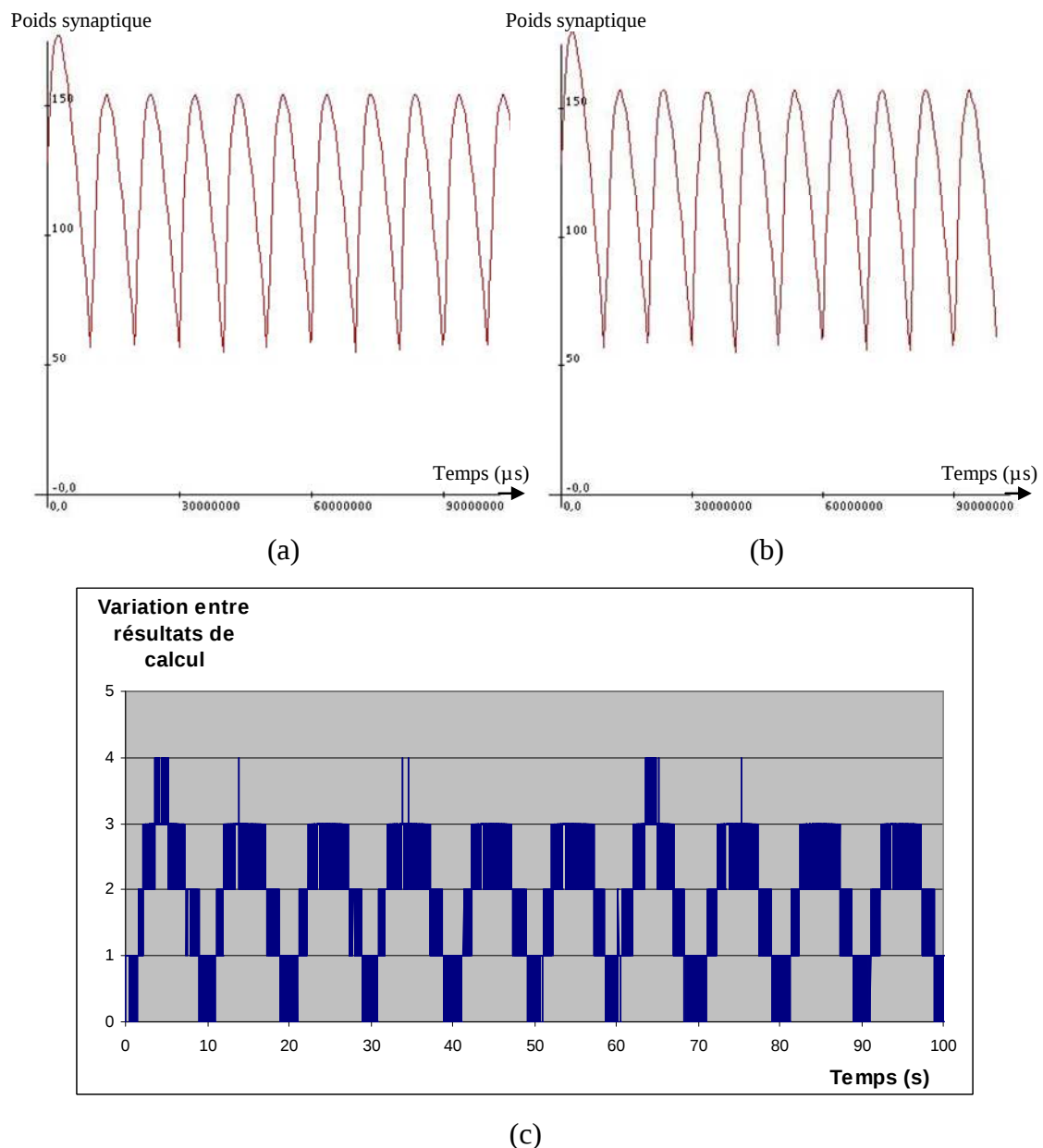
Figure 4.18. Mise en évidence de l'erreur accumulée. (a) Résultat de la simulation matérielle d'une connexion à évolution périodique. (b) Résultat de la simulation logicielle. (c) Valeur absolue de la variation de l'erreur entre le calcul logiciel et le calcul matériel.
