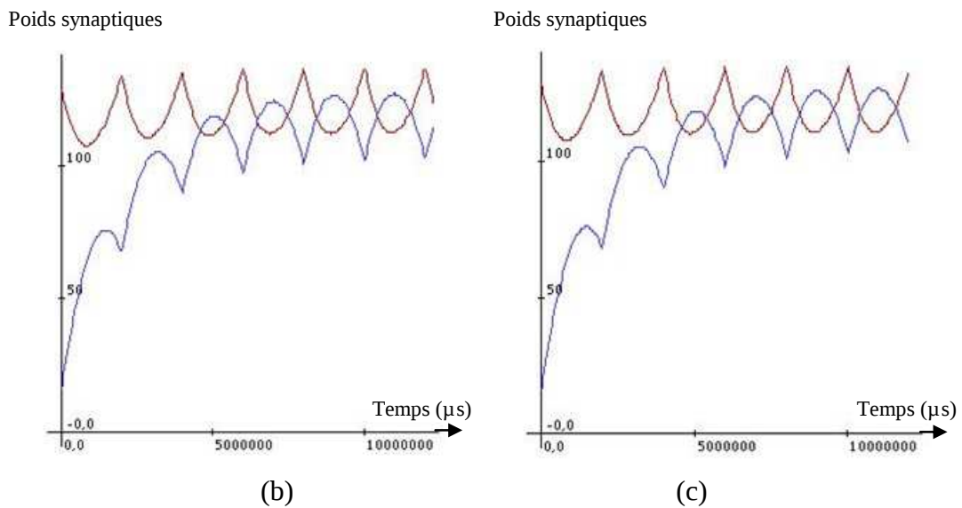
Figure 4.16. Simulation d'un réseau de deux neurones et deux connexions : les fréquences d'oscillation sont légèrement différentes pour créer une périodicité dans les changements des phases. Les paramètres du calcul de la plasticité sont les mêmes que l'expérimentation illustrée par la figure 4.14. (a) Spécification du réseau : les poids initiaux ont des valeurs différentes (16 et 128). Les changements de sens dans le groupement des paires de potentiels d'action créent, à un certain moment, des inversions de signes dans la différence des phases. Quand cette dernière est nulle, on parle alors de superposition de phases. (b) Simulation matérielle conforme aux résultats attendus : les deux connexions évoluent d'une façon antagoniste en présentant des changements de sens périodiques. (c) La simulation logicielle : un comportement similaire au calcul matériel.
