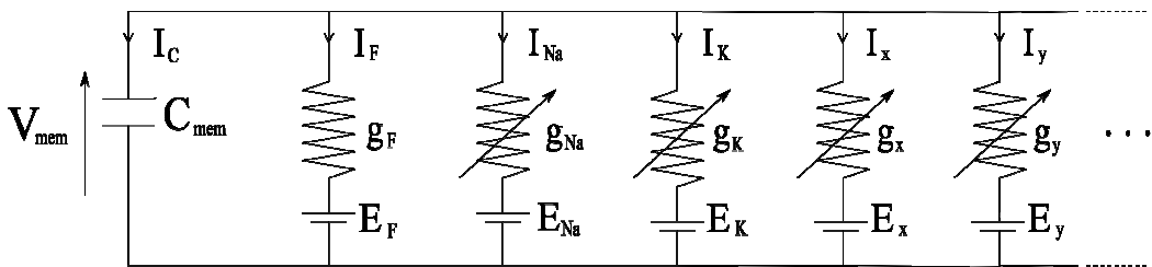
Figure 1.6 Le formalisme de Hodgkin-Huxley.
