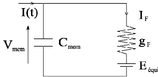
Figure 1.4 Mise en circuit du modèle Integrate-and-Fire avec fuite.
