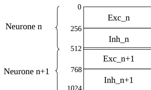
Figure A.7. Organisation d'une RAM de stockage des ISIs.
