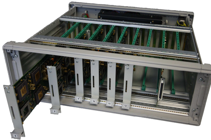
Figure 2.13. Photographie du système rack avec six cartes Ekerö et une carte Thalamus .
