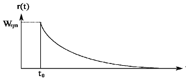
Figure 1.7. Evolution de la synapse en exponentielle décroissante suite à une stimulation produite à t_0 selon l'équation (1.6)
