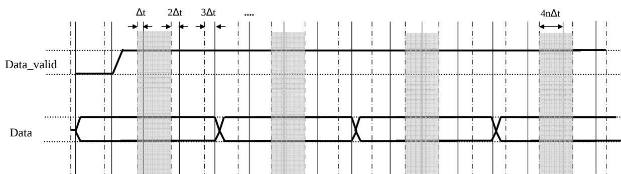
Figure 4.4. Illustration de l'incertitude sur la fréquence d'oscillation dans la communication parallèle asynchrone.
