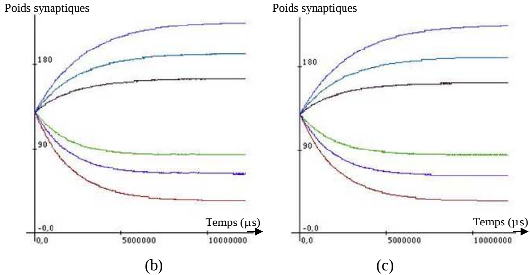
Figure 4.15. Simulations d'un réseau composé de 3 neurones et 6 connexions : les paramètres de l'équation de la plasticité sont identiques pour la LTP et la LTD : \tau_p = \tau_q = 14,8 ms, \tau_j = 28 ms, \tau_i = 88 ms, A_p = A_q = 0,1 , w_{LTP} = 255 et w_{LTD} = 0 . (a) La spécification du réseau est réalisée de telle sorte que tous les neurones sont connectés dans les deux sens au neurone N1 . (b) Résultat de la simulation matérielle : les poids convergent vers 6 valeurs finales différentes. (c) La simulation logicielle donne des valeurs très proches.
